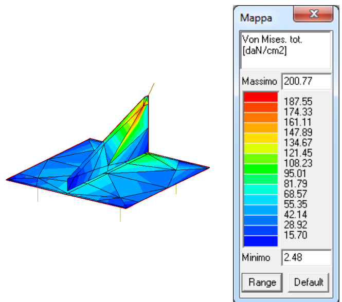
Tensioni condizione D
