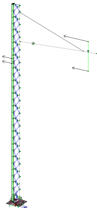
Carichi dovuti al vento trasversale (X)
