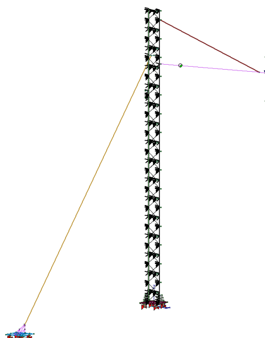
Carichi dovuti al vento longitudinale (Y)
