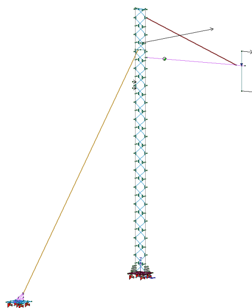
Carichi dovuti al tiro dei conduttori
