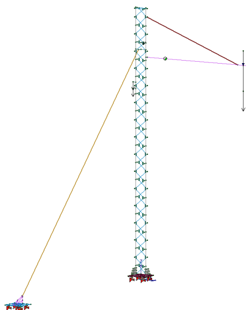
Carichi dovuti al peso dei conduttori
