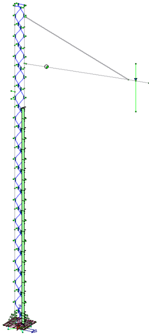
Carichi dovuti al vento trasversale aerodinamico (X)
