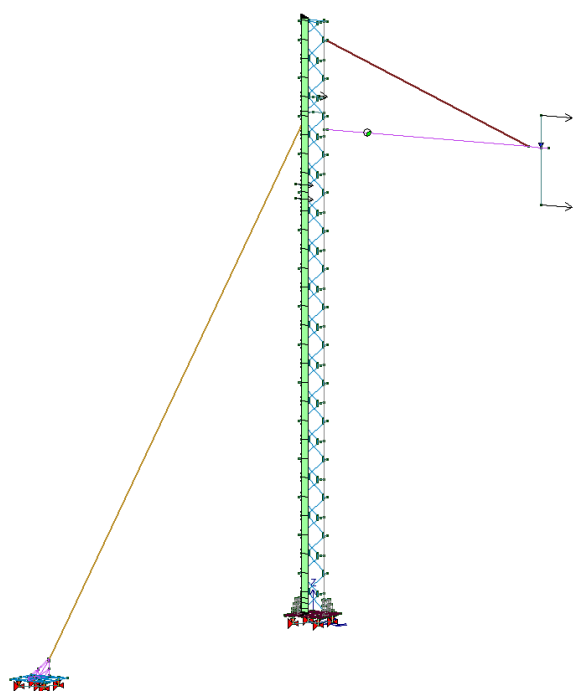
Carichi dovuti al vento trasversale (X)
