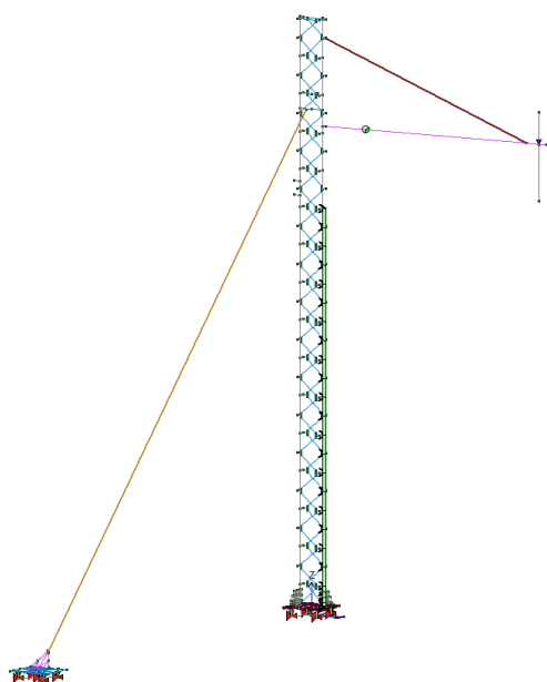
Carichi dovuti al vento trasversale aerodinamico
