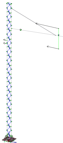
Carichi dovuti al tiro dei conduttori
