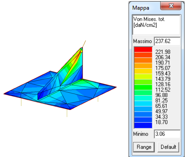
Tensioni condizione D
