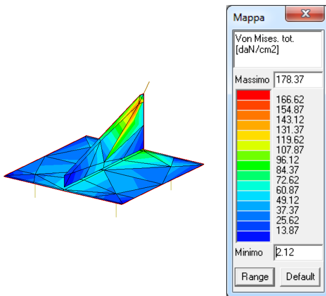
Tensioni condizione B
