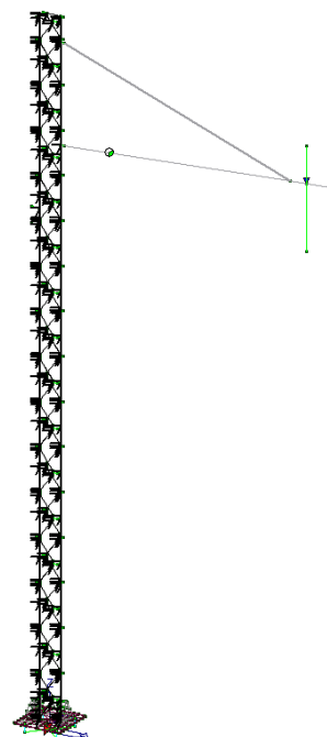
Carichi dovuti al vento longitudinale (Y)
