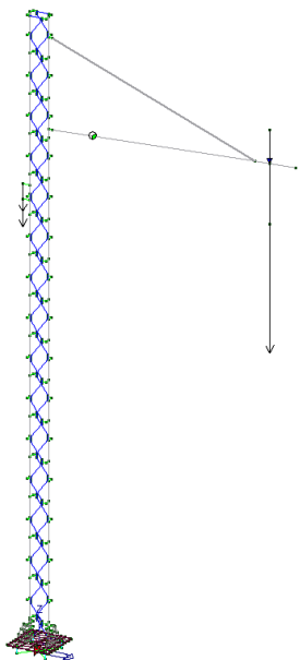
Carichi dovuti al peso dei conduttori
