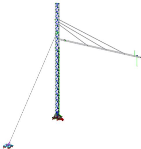
Carichi dovuti al vento aerodinamico (X)
