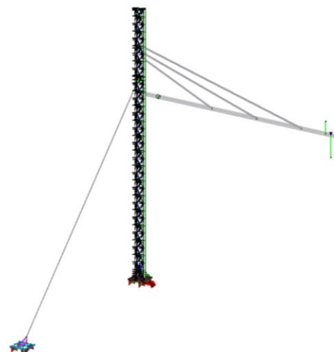
Carichi dovuti al vento longitudinale (Y)
