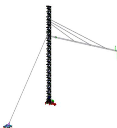
Carichi dovuti al vento longitudinale (Y)
