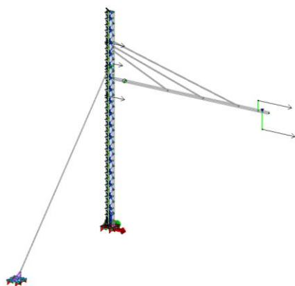
Carichi dovuti al vento trasversale (X)
