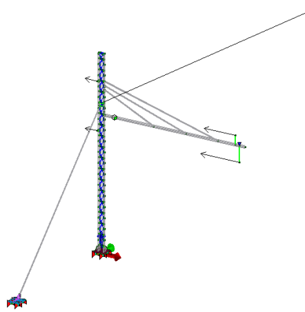
Carichi dovuti al tiro dei conduttori
