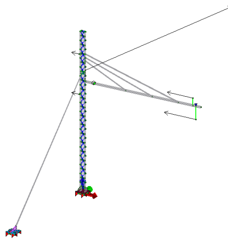
Carichi dovuti al tiro dei conduttori
