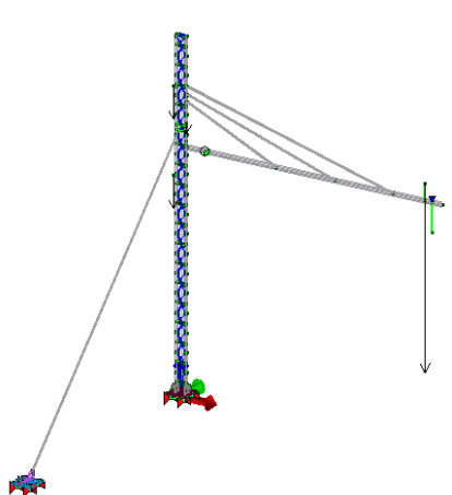
Carichi dovuti al peso dei conduttori
