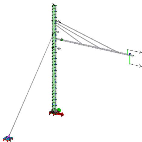
Carichi dovuti al vento trasversale (X)
