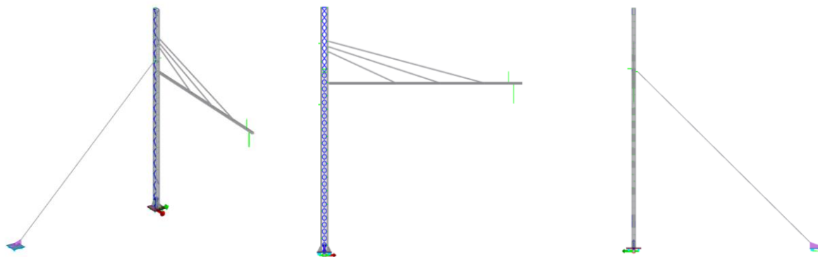
Modellazione del palo picc. 172PR agli elementi finiti
