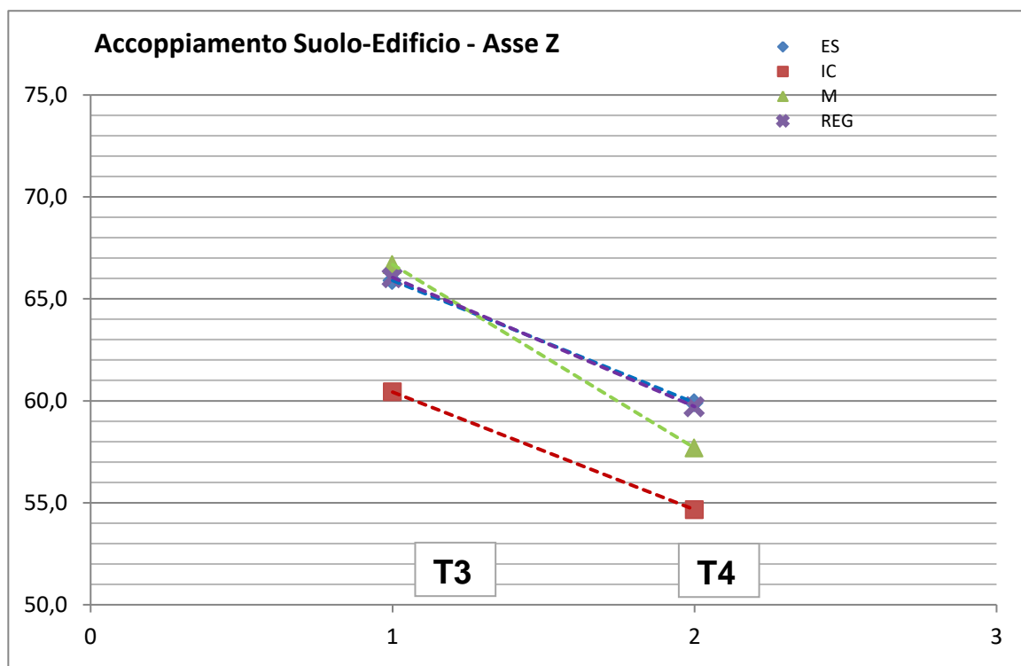
Figura 4: Attenuazione complessiva per accoppiamento suolo-fondazioni e amplificazione risonanza solaio, ricavata dai rilievi sperimentali del Leq,t_e sull'attuale linea in esercizio, lungo l'asse Z
