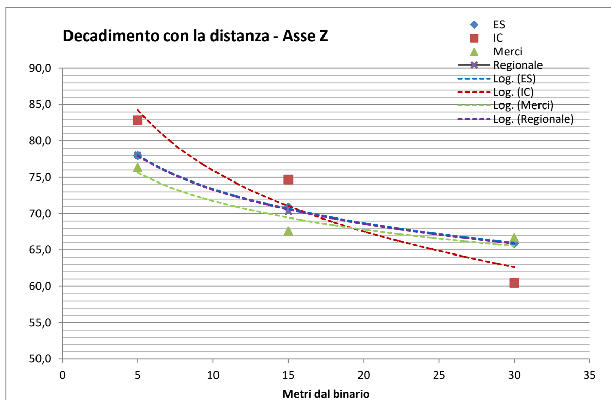
Figura 3: Curva di attenuazione del Leq,te in funzione della distanza dal binario, ricavata dai rilievi sperimentali sull'attuale linea in esercizio lungo l'asse Z, in corrispondenza della Terna 1 (5 metri), della Terna 2 (15 metri) e della Terna 3 (30 metri).
