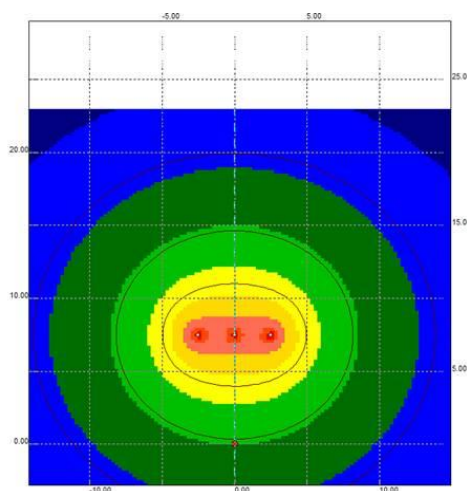
Fig.2 – Fascia di rispetto a 3 \mu T su terna di sbarre AT ( I=200 A)
