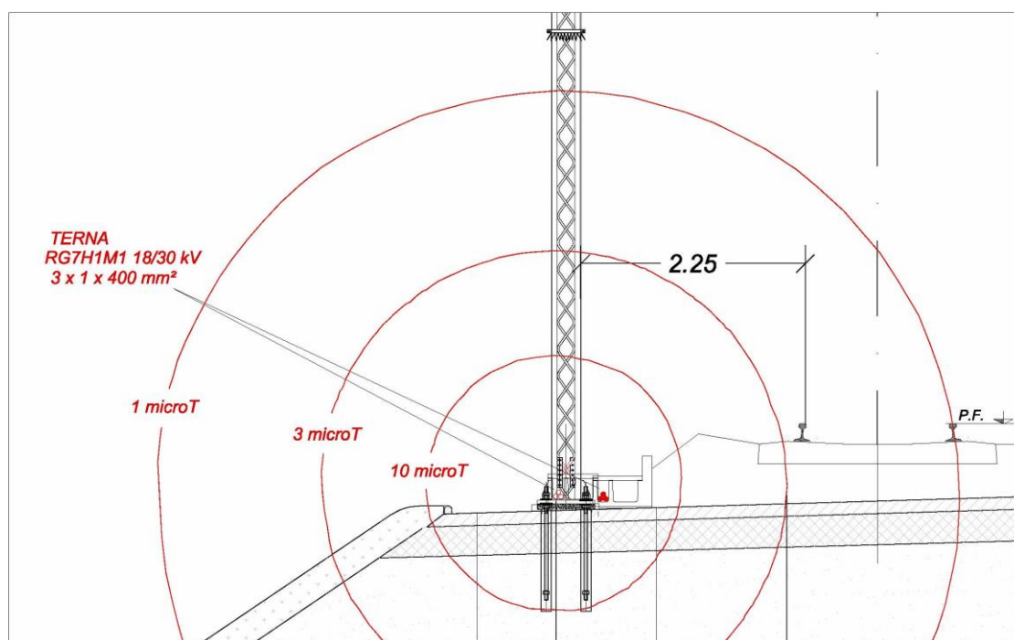
Fig.3 – Campo magnetico generato dal cavidotto a 30 kV
