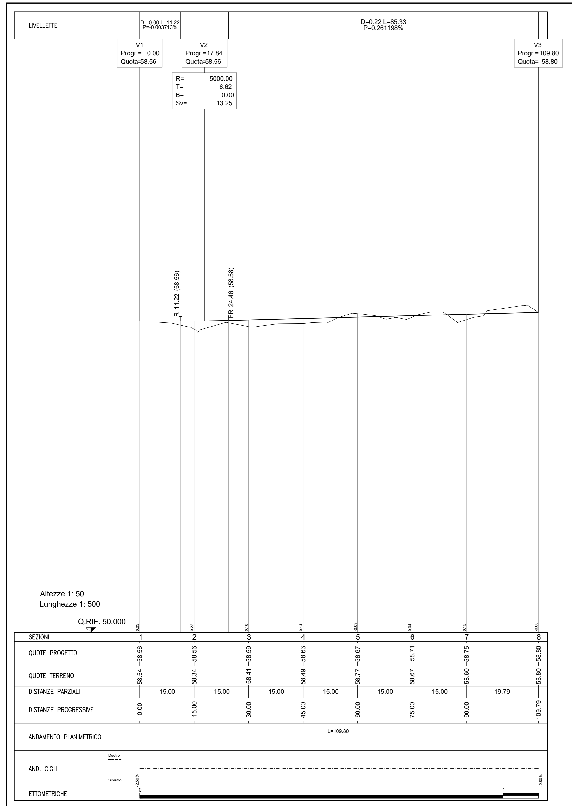
PROFILO LONGITUDINALE 1:500
