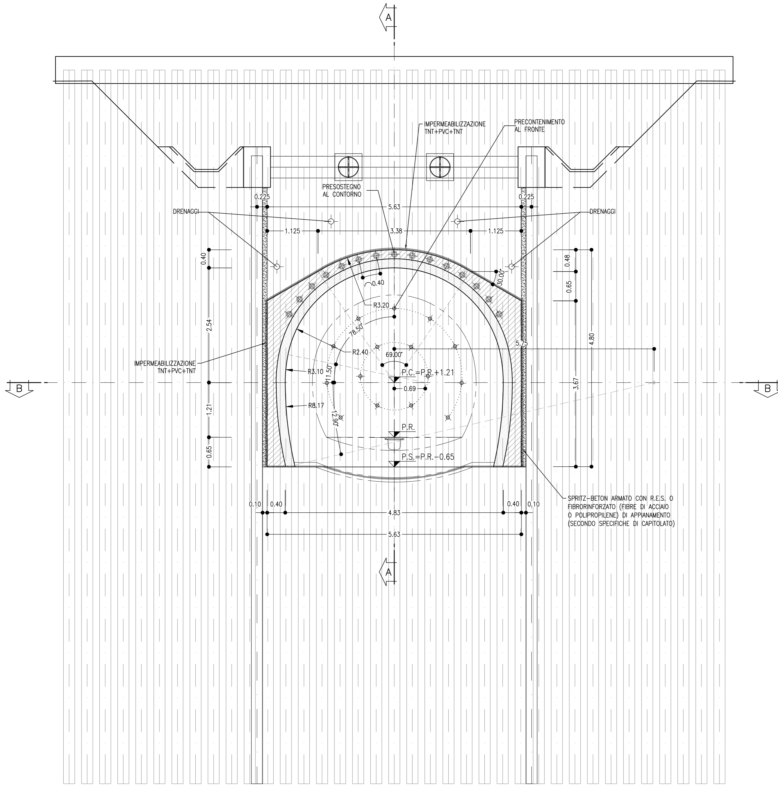
SEZIONE TRASVERSALE TIPOLOGICA SCALA 1:50 DIMA D'ATTACCO
