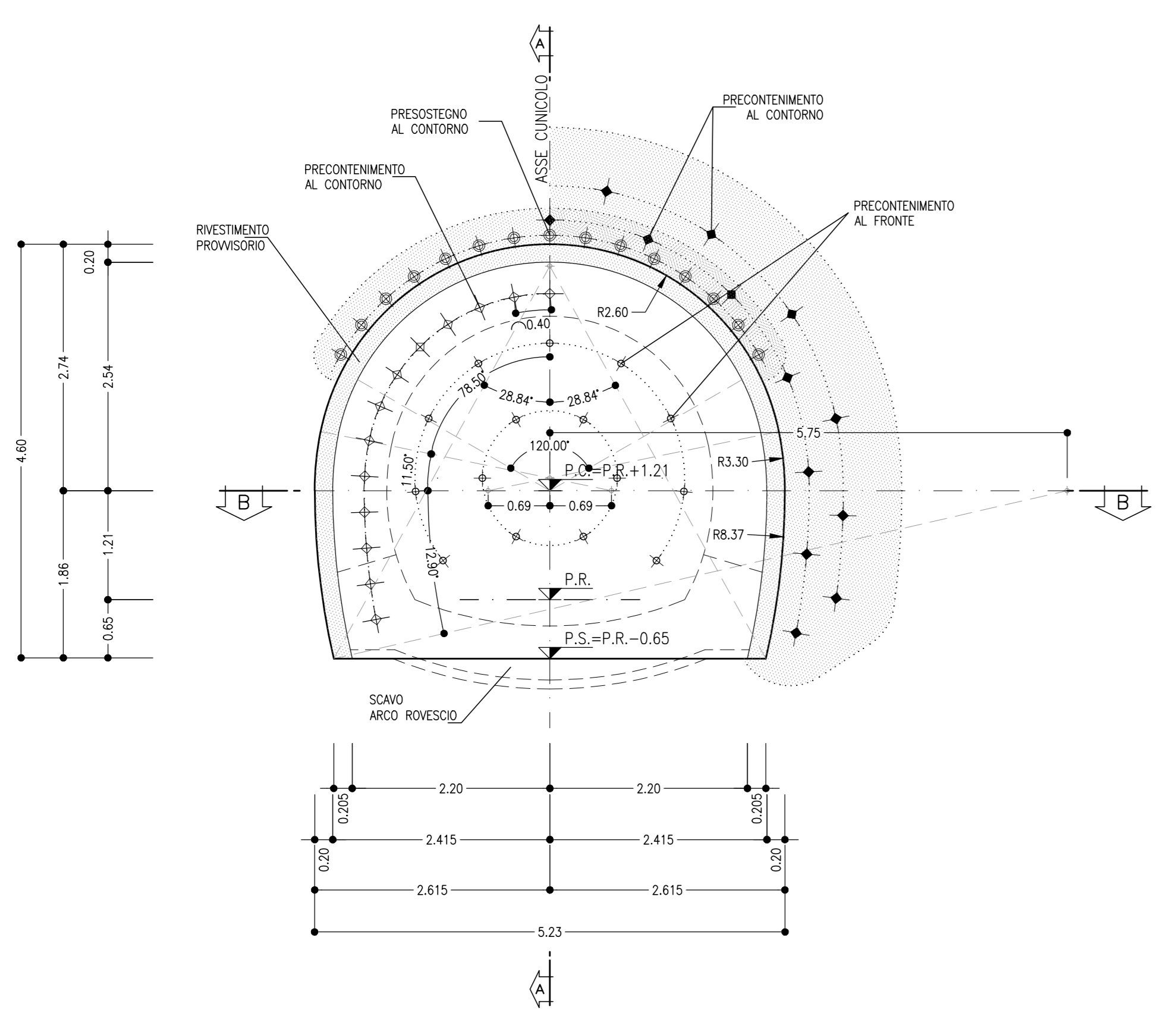
SEZIONE TRASVERSALE TIPOLOGICA SCALA 1:50 CONCIO D'ATTACCO
