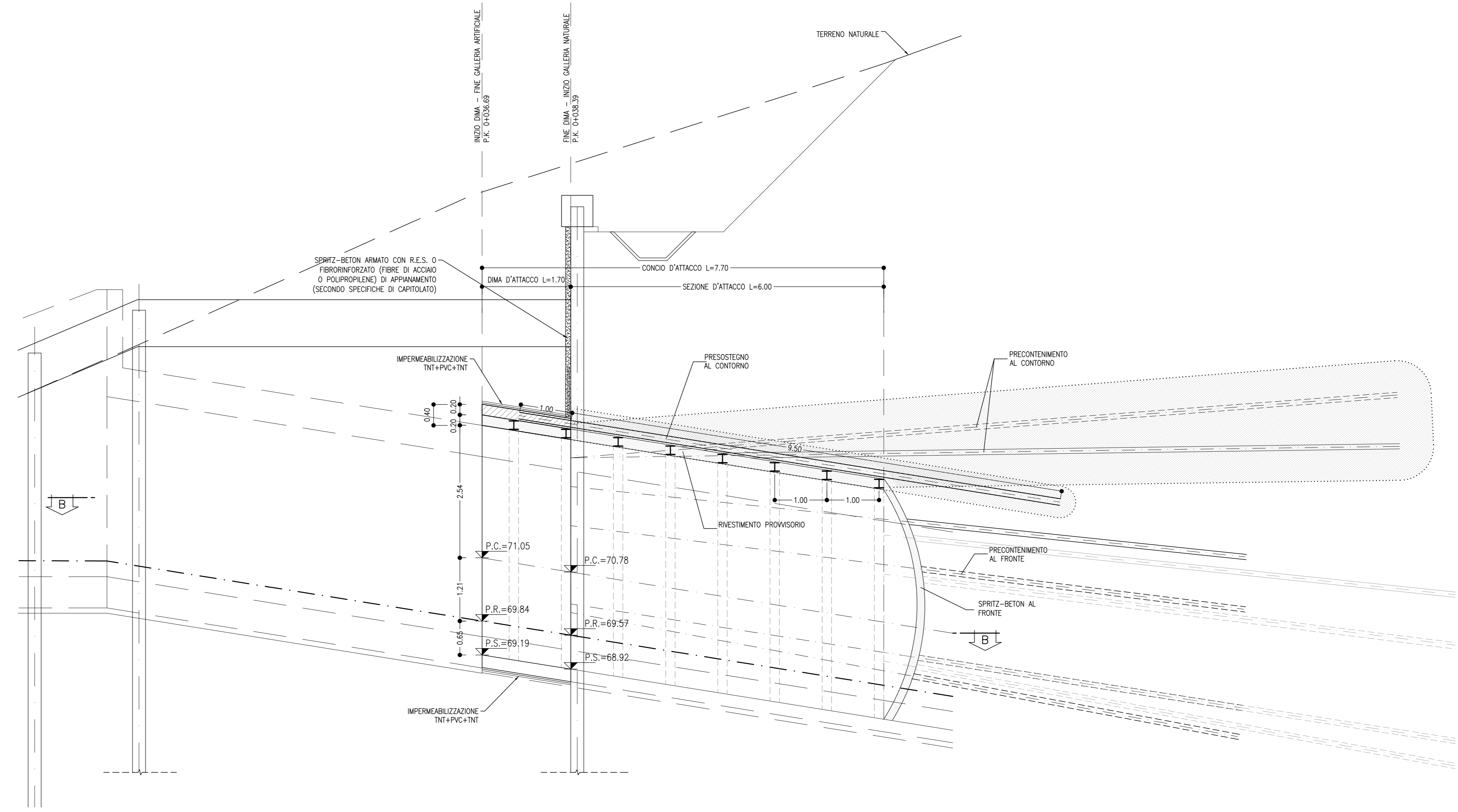
PROFILO LONGITUDINALE SCALA 1:50 SEZIONE A-A
