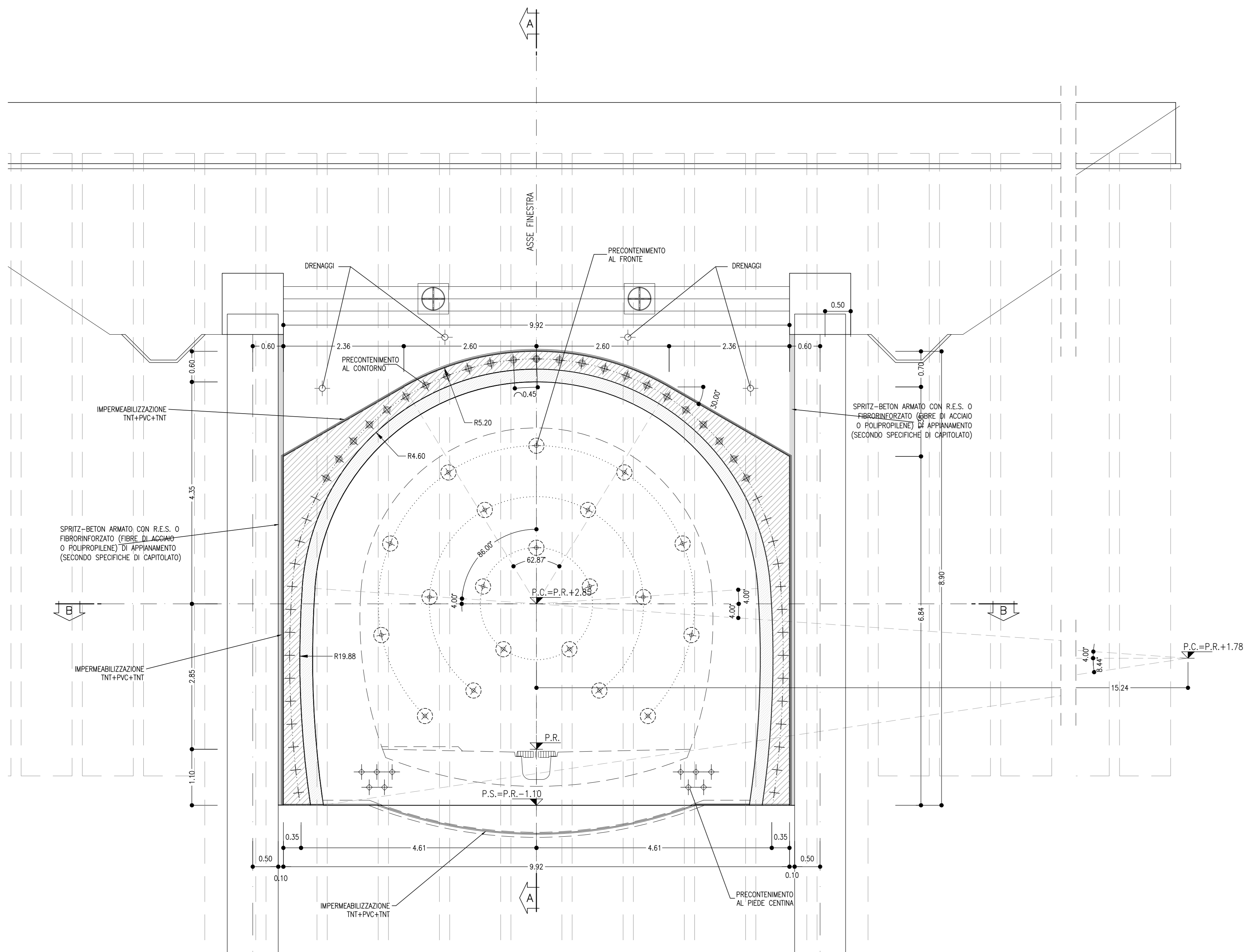
SEZIONE TRASVERSALE TIPOLOGICA SCALA 1:50 DIMA D'ATTACCO
