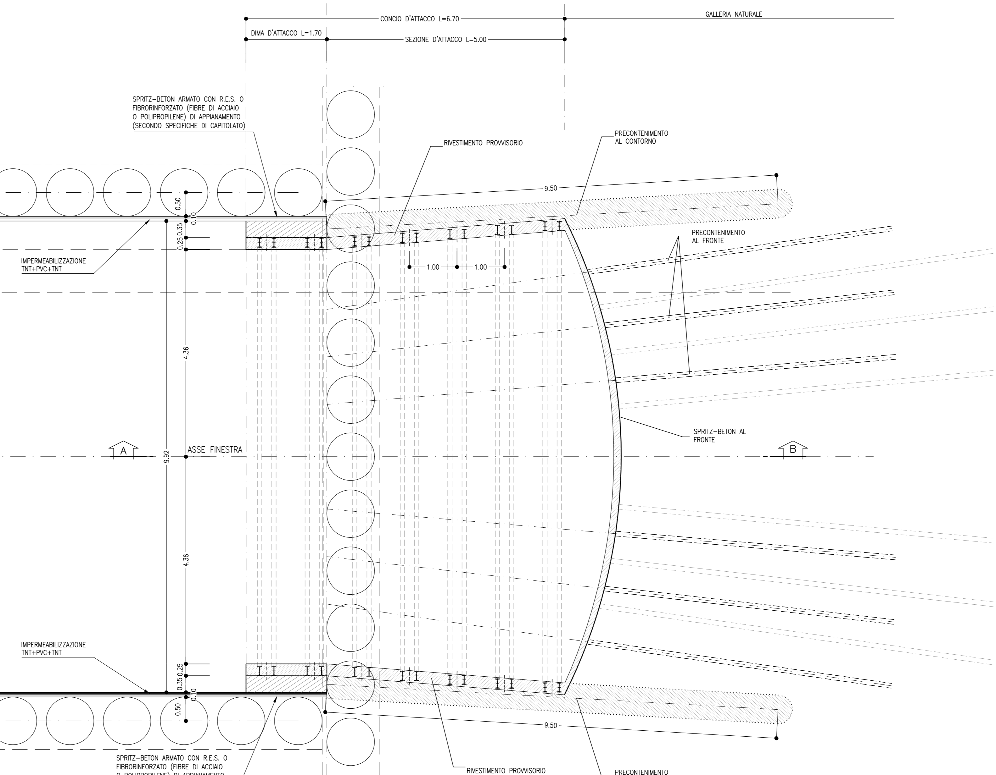
DIMA E CONCIO D'ATTACCO SCALA 1:50 SEZIONE B-B
