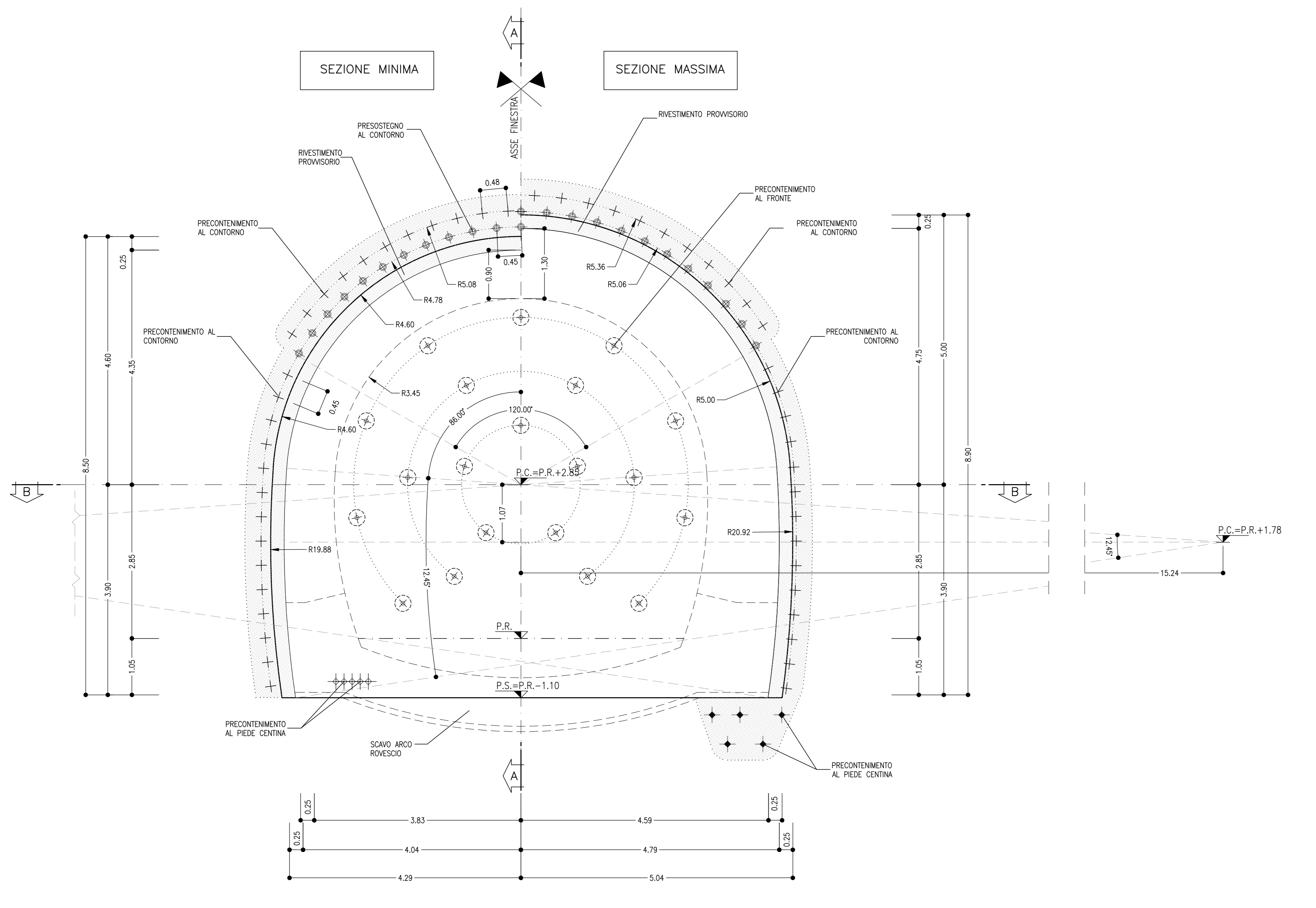
SEZIONE TRASVERSALE TIPOLOGICA SCALA 1:50 CONCIO D'ATTACCO
