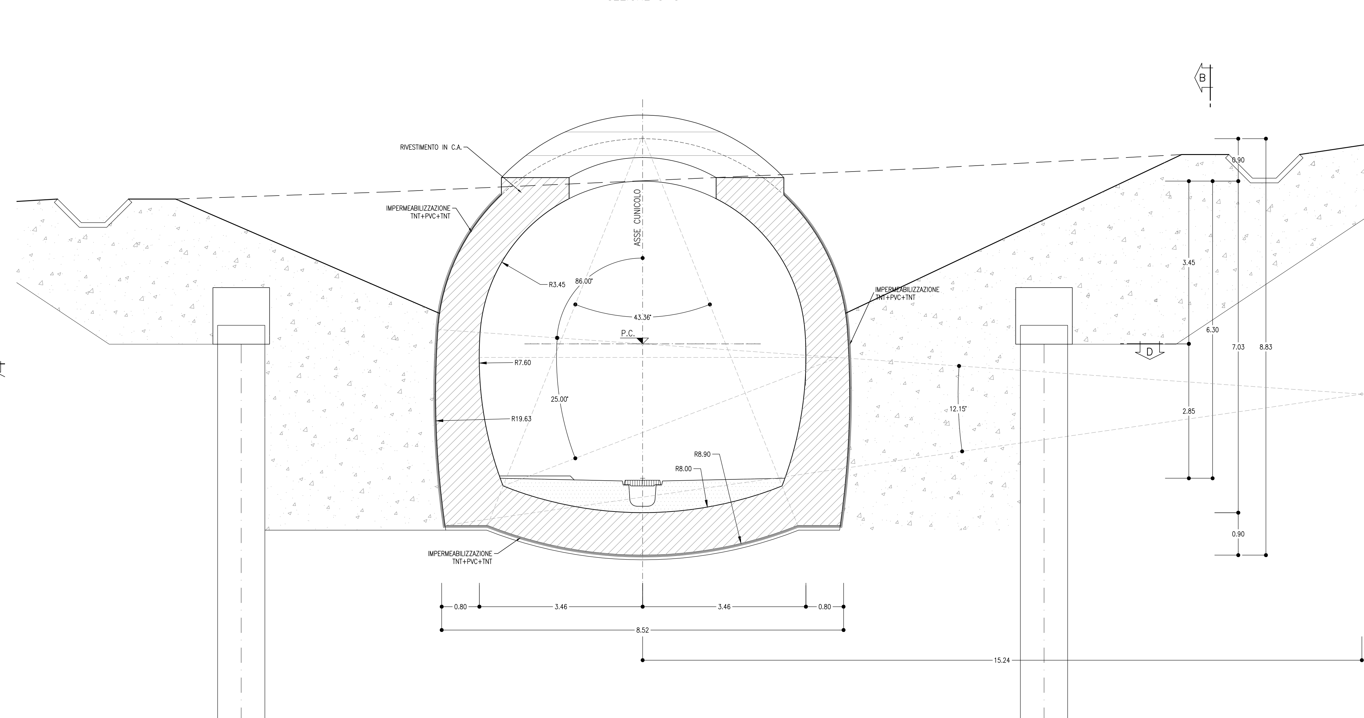
PORTALE D'IMBOCCO SCALA 1:50 SEZIONE C-C
