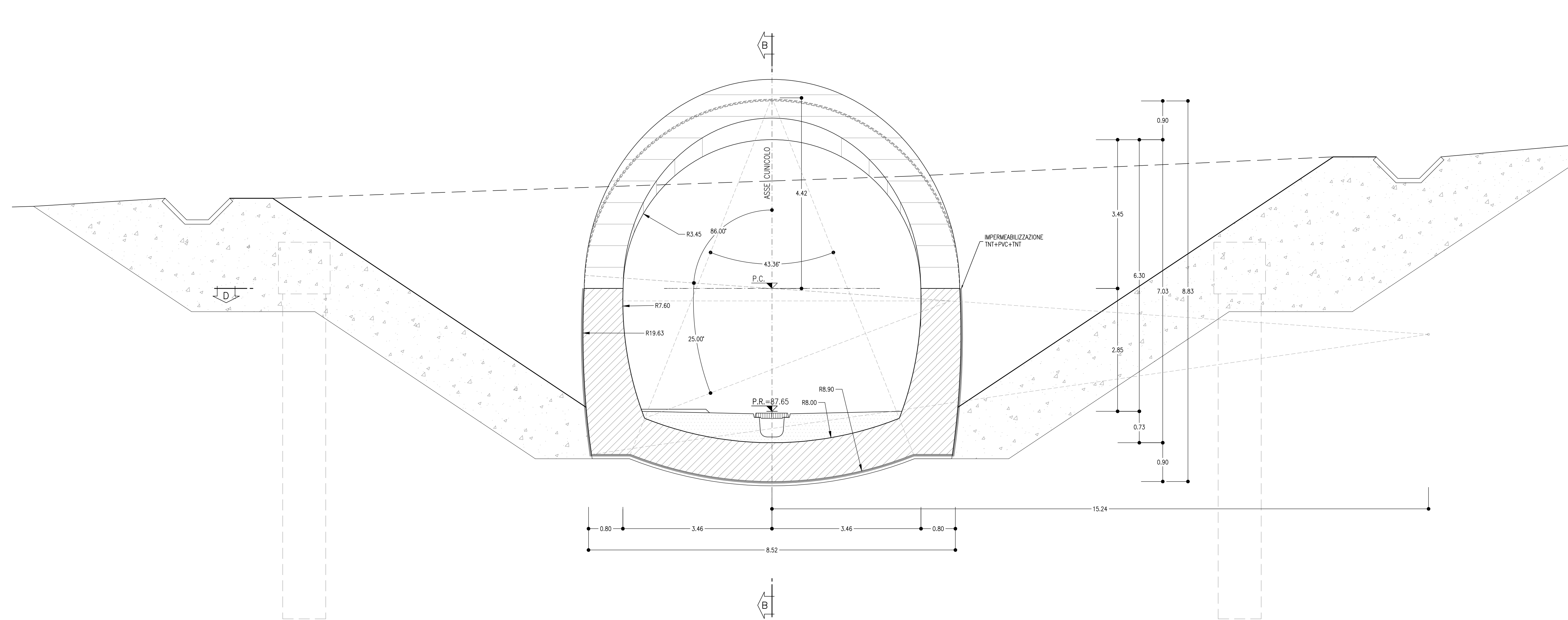
PORTALE DI IMBOCCO SCALA 1:50 SEZIONE A-A
