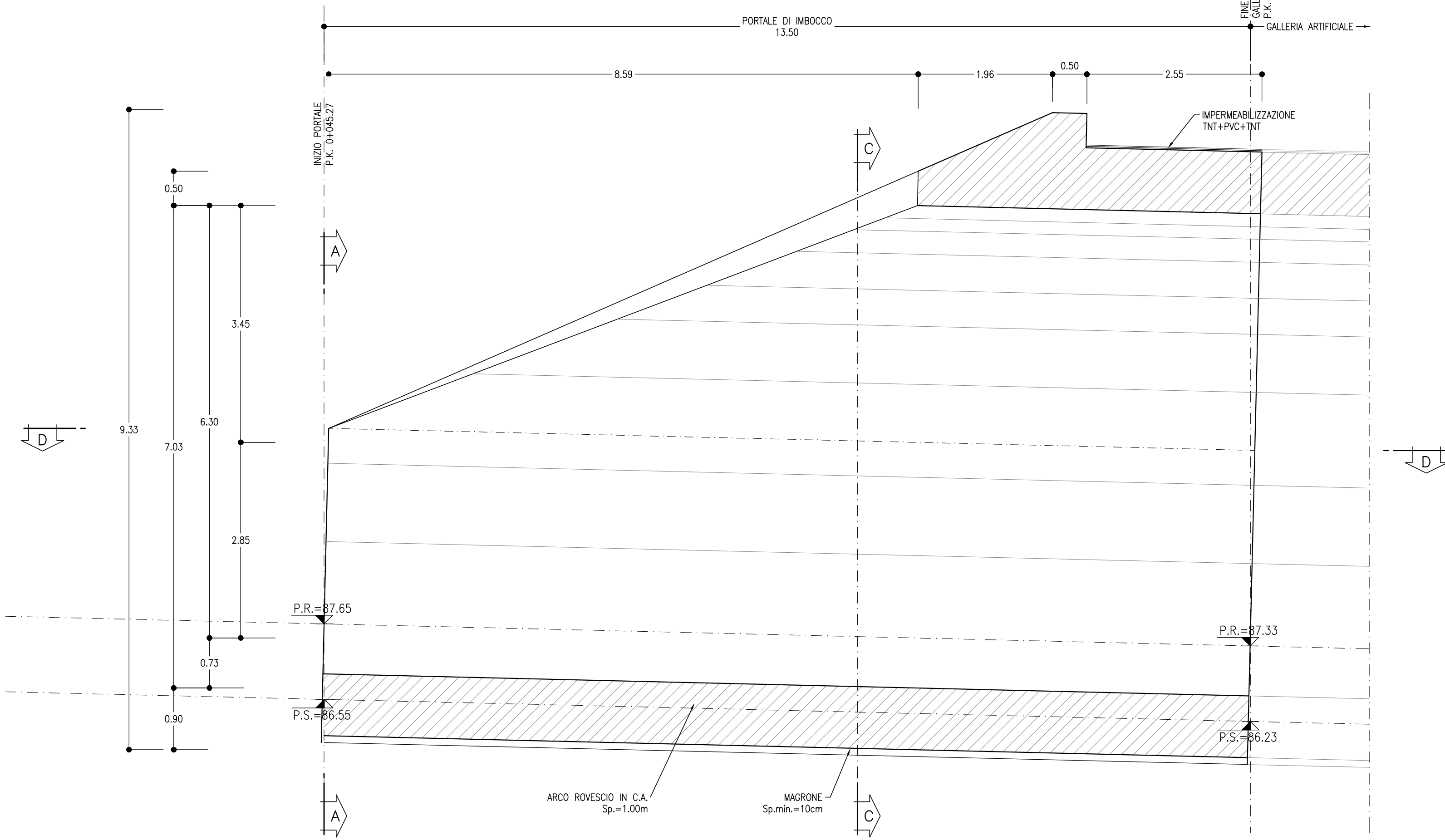
PROFILO LONGITUDINALE SCALA 1:50 SEZIONE B-B
