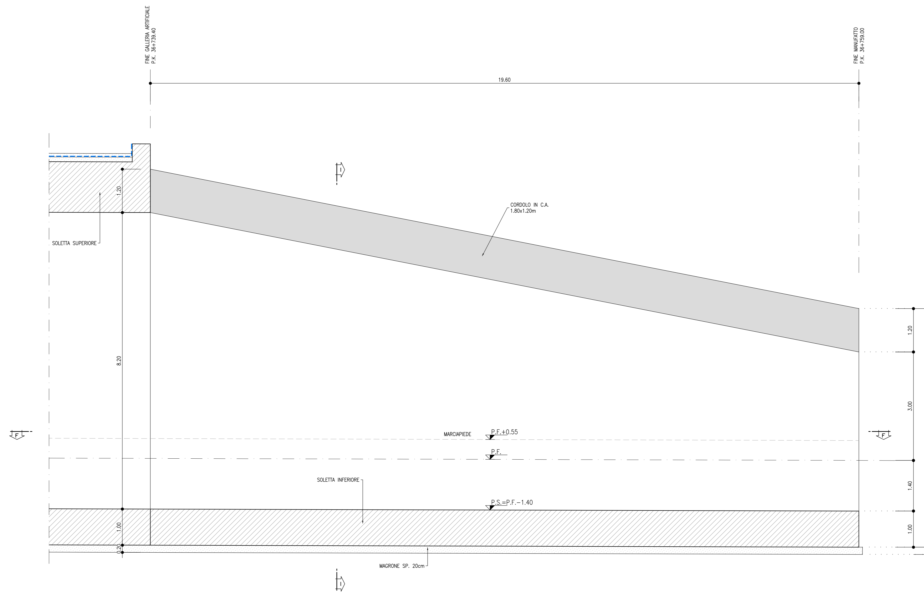
PROFILO LONGITUDINALE SCALA 1:50 SEZIONE E-E
