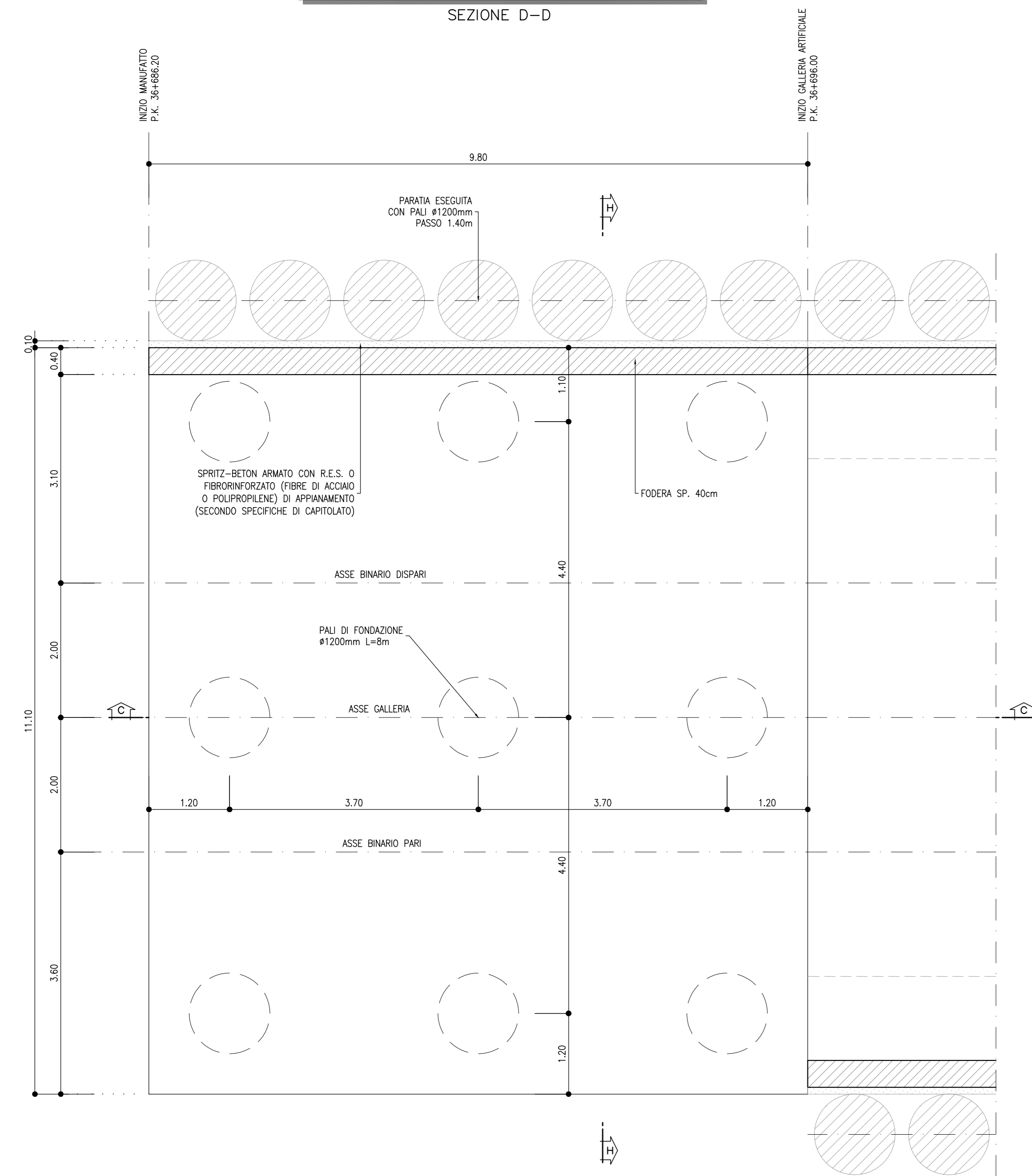
PIANTA SCALA 1:50 SEZIONE D-D
