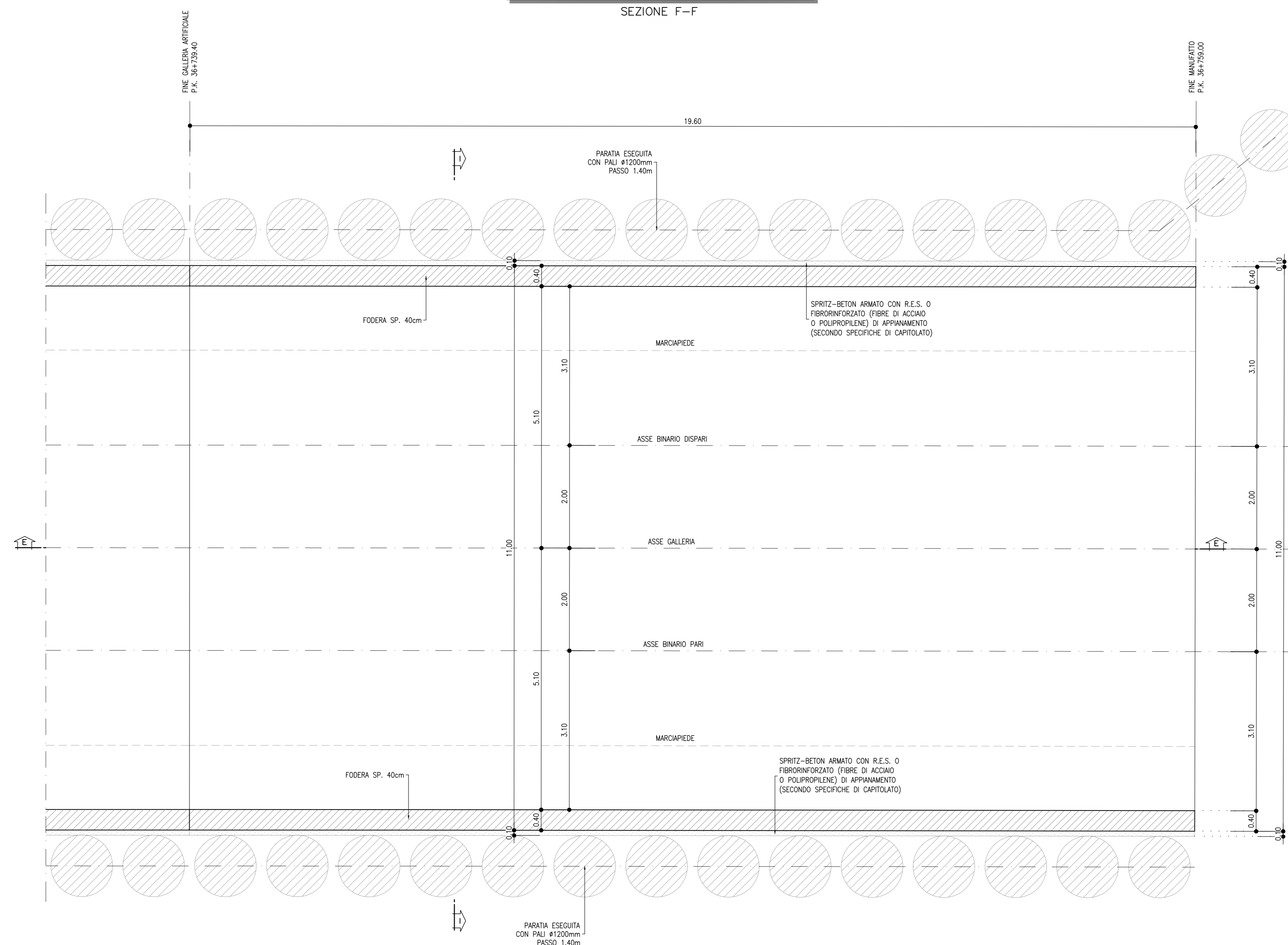
PIANTA SCALA 1:50 SEZIONE F-F
