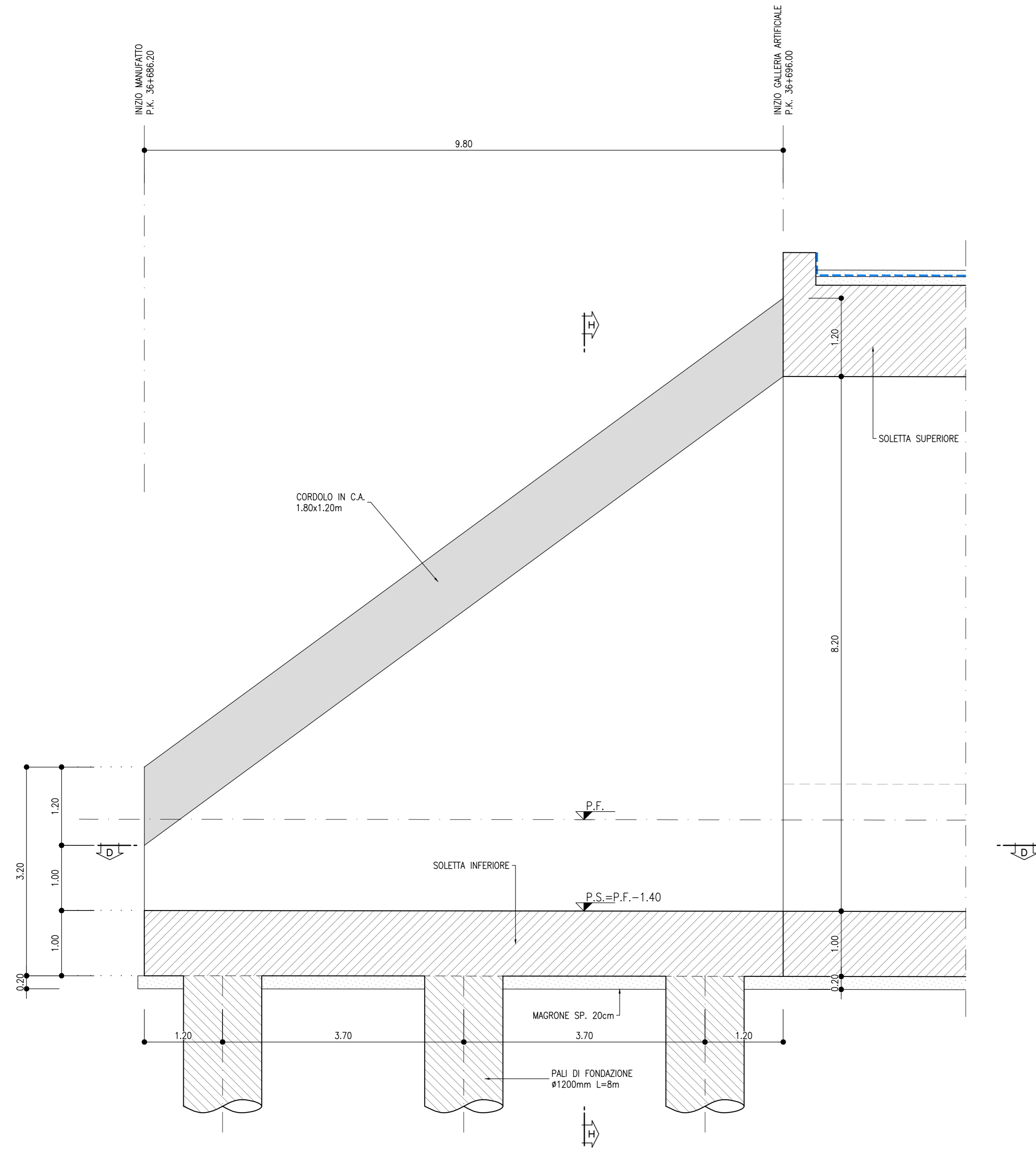
PROFILO LONGITUDINALE SCALA 1:50 SEZIONE C-C
