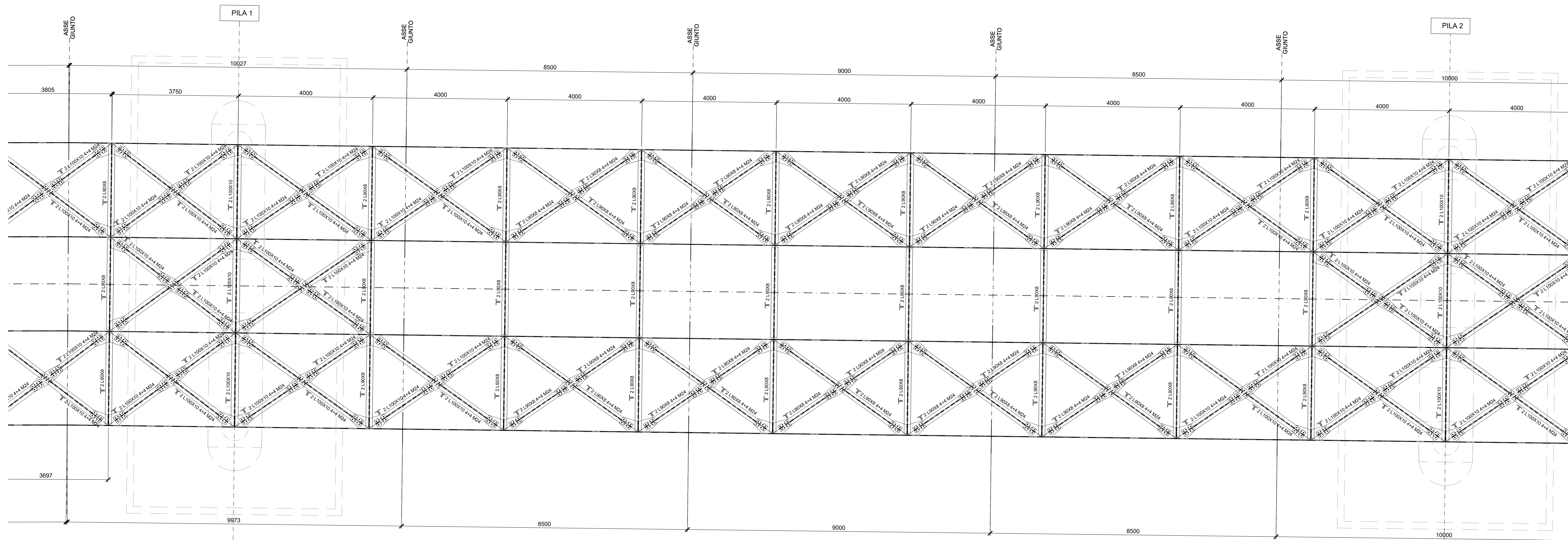
PIANTA CONTROVENTI INFERIORI - TRAVATA 2 Scala 1:50
