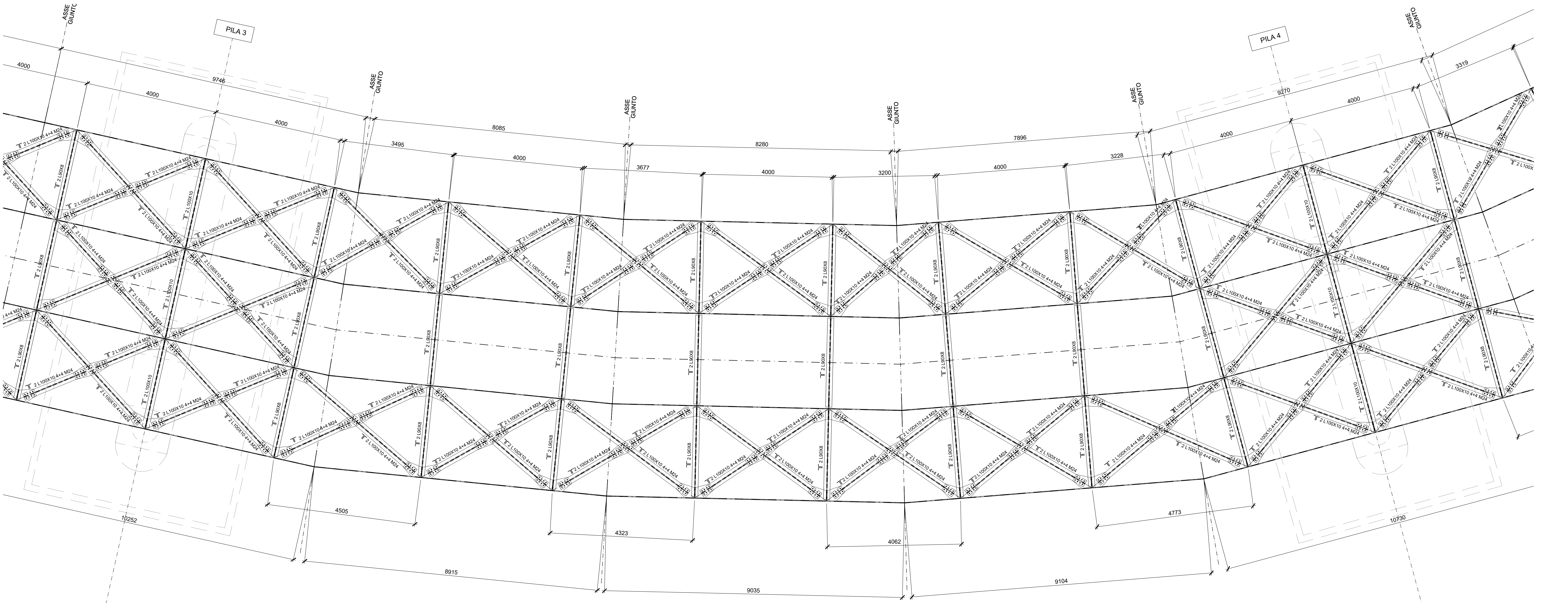
PIANTA CONTROVENTI INFERIORI - TRAVATA 4 Scala 1:50
