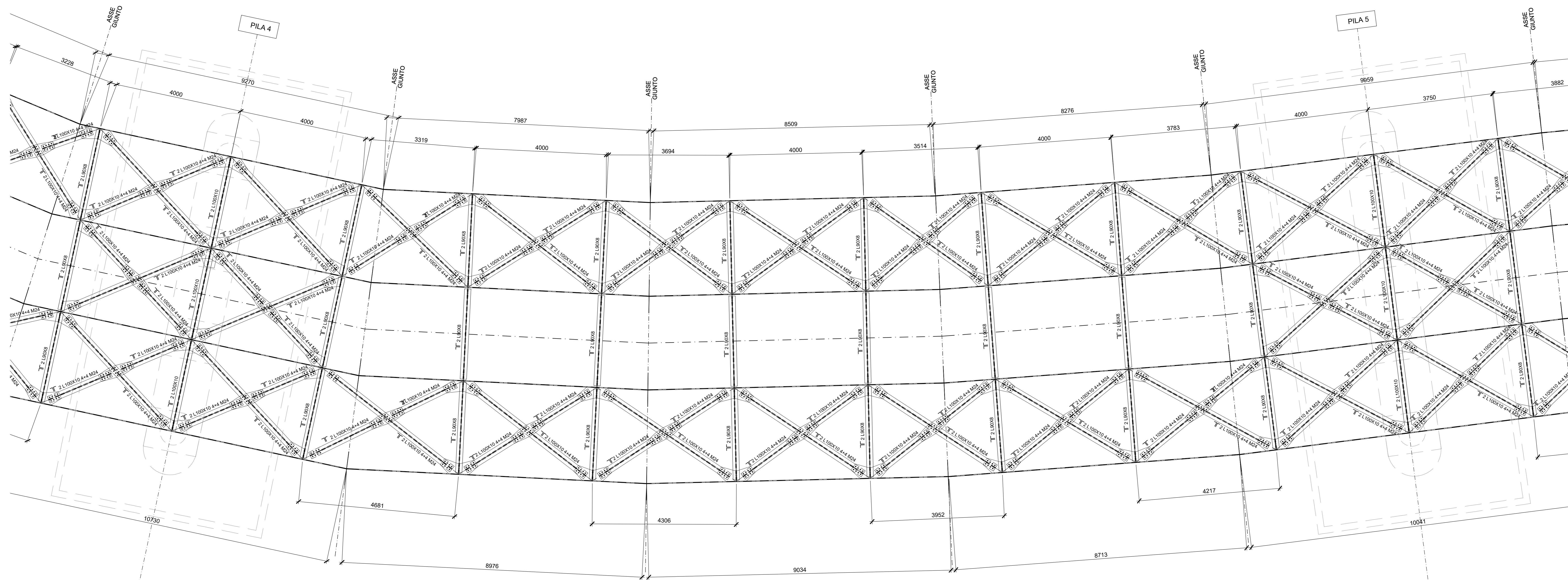
PIANTA CONTROVENTI INFERIORI - TRAVATA 5 Scala 1:50
