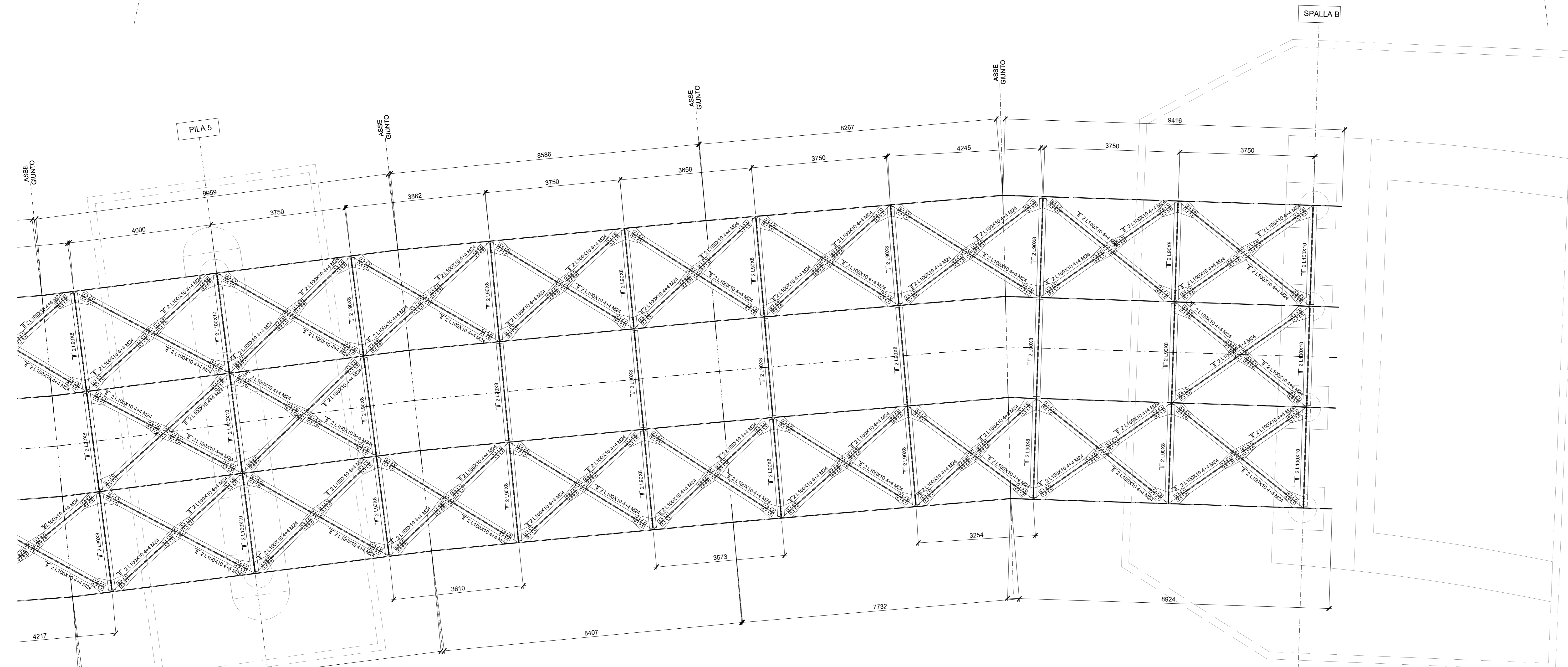
PIANTA CONTROVENTI INFERIORI - TRAVATA 6 Scala 1:50
