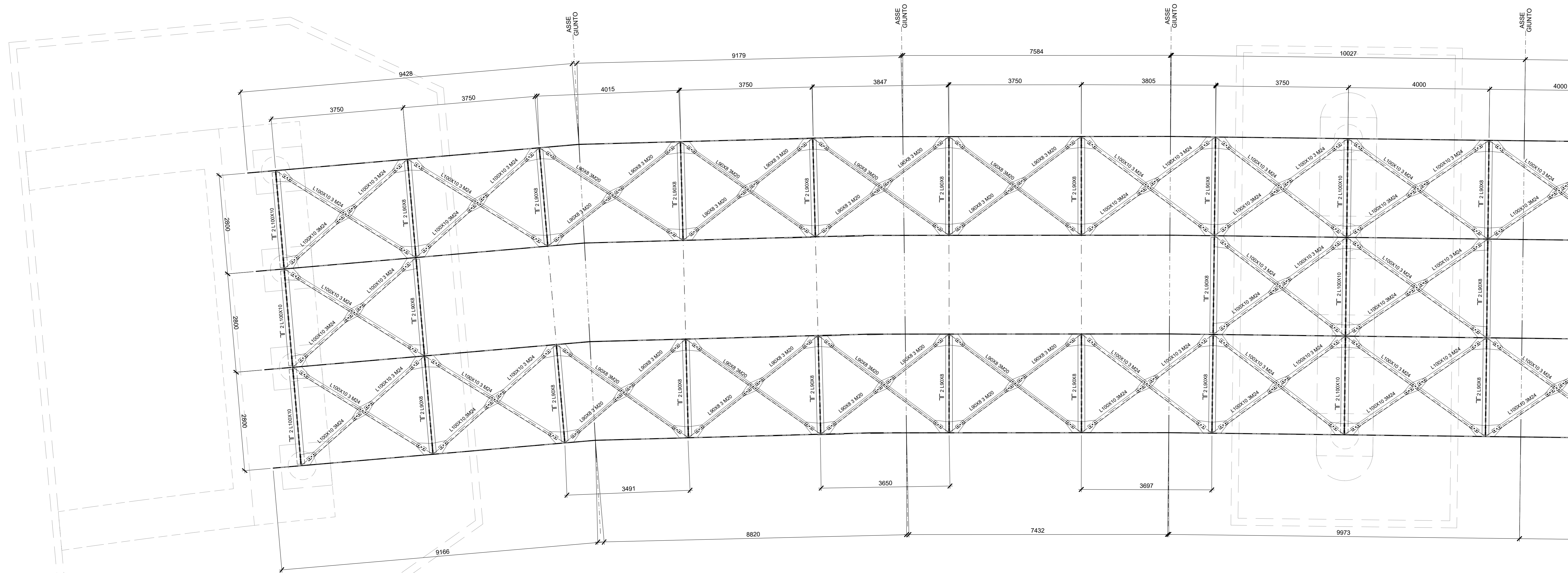
PIANTA CONTROVENTI SUPERIORI - TRAVATA 1 Scala 1:50
