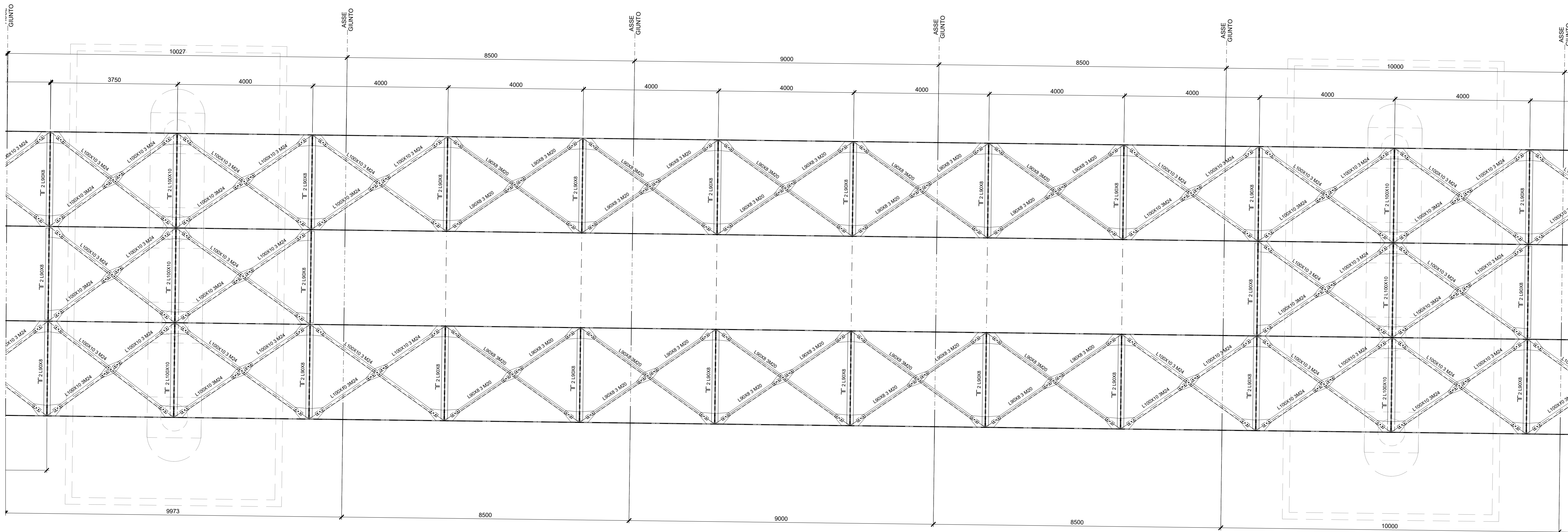
PIANTA CONTROVENTI SUPERIORI - TRAVATA 2 Scala 1:50
