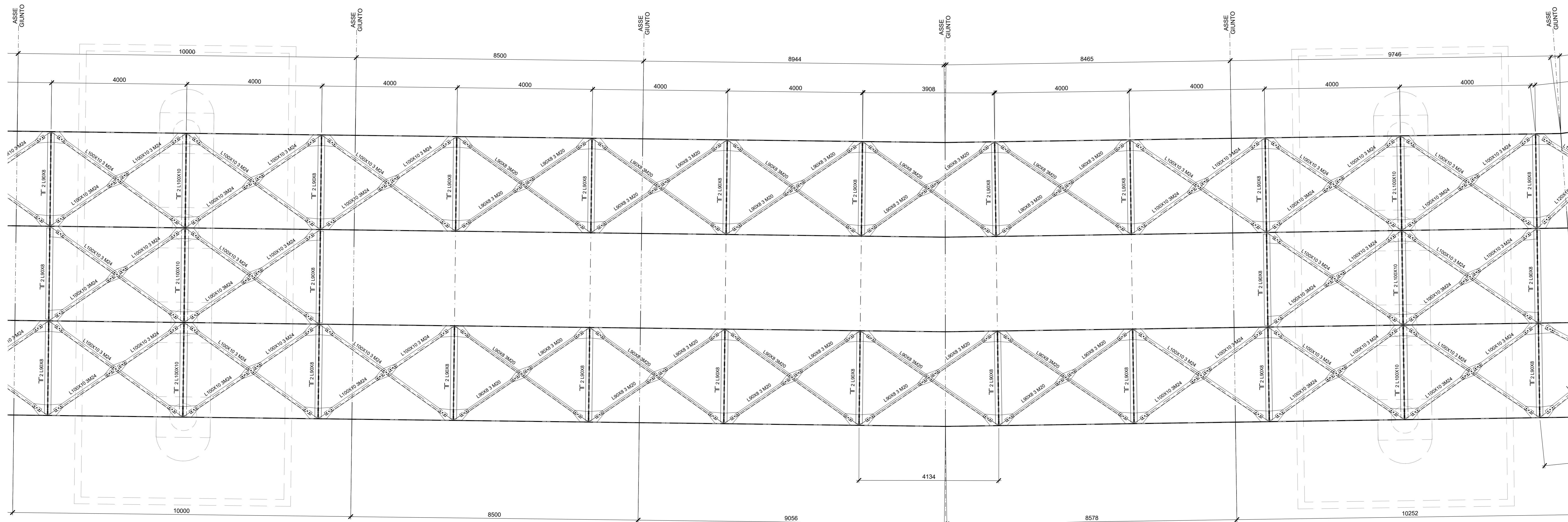
PIANTA CONTROVENTI SUPERIORI - TRAVATA 3 Scala 1:50
