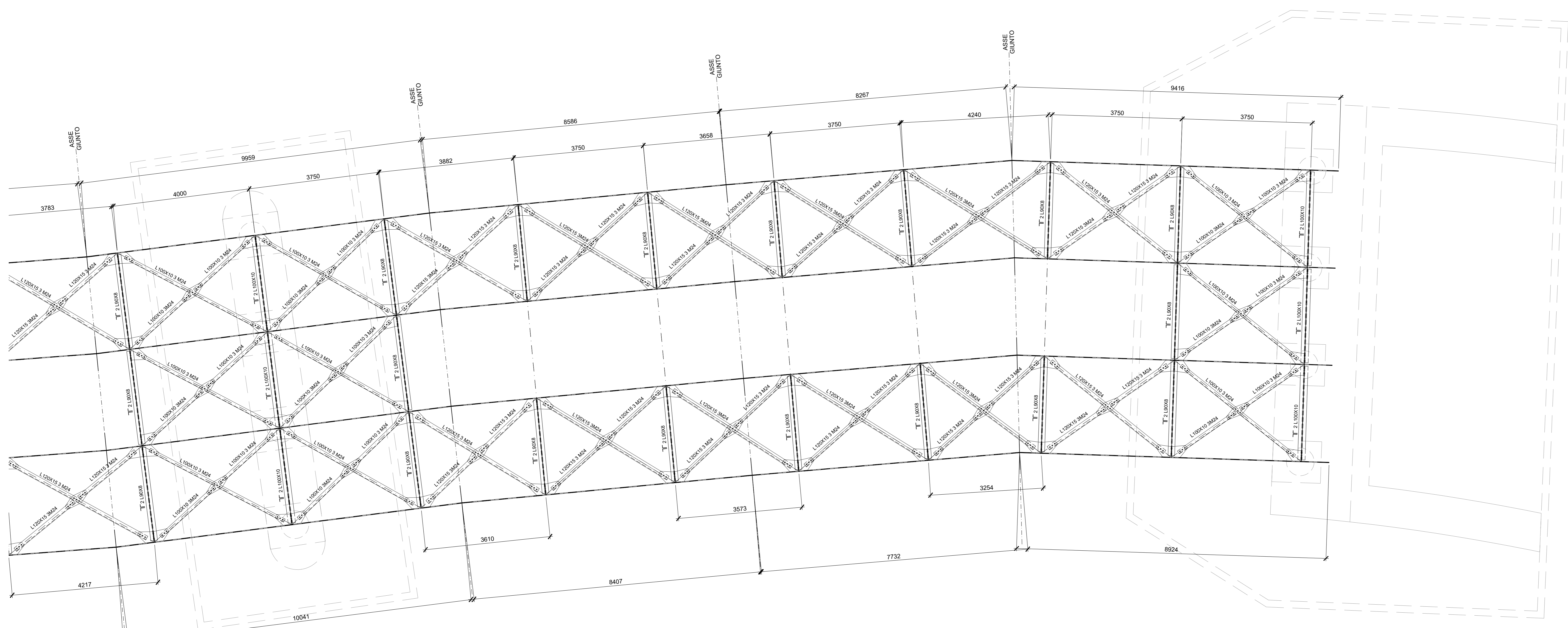
PIANTA CONTROVENTI SUPERIORI - TRAVATA 6 Scala 1/50
