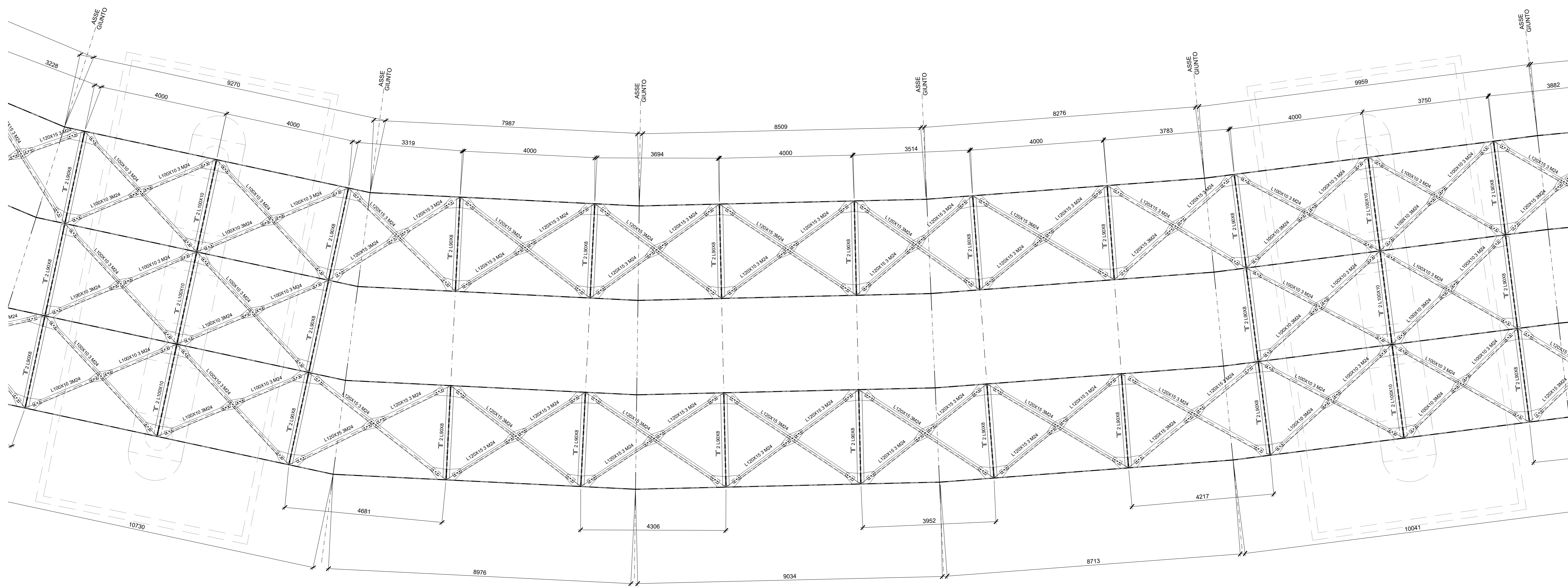
PIANTA CONTROVENTI SUPERIORI - TRAVATA 5 Scala 1/50
