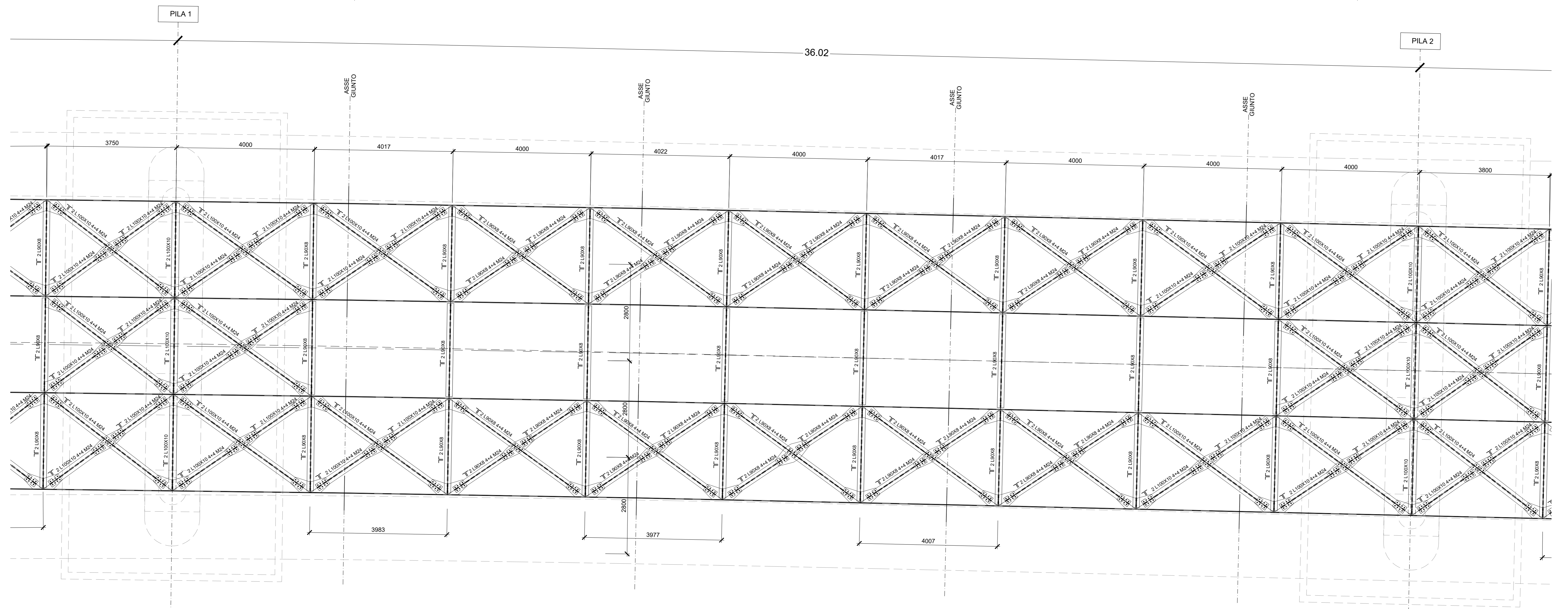
PIANTA CONTROVENTI INFERIORI - TRAVATA 2 Scala 1:50
