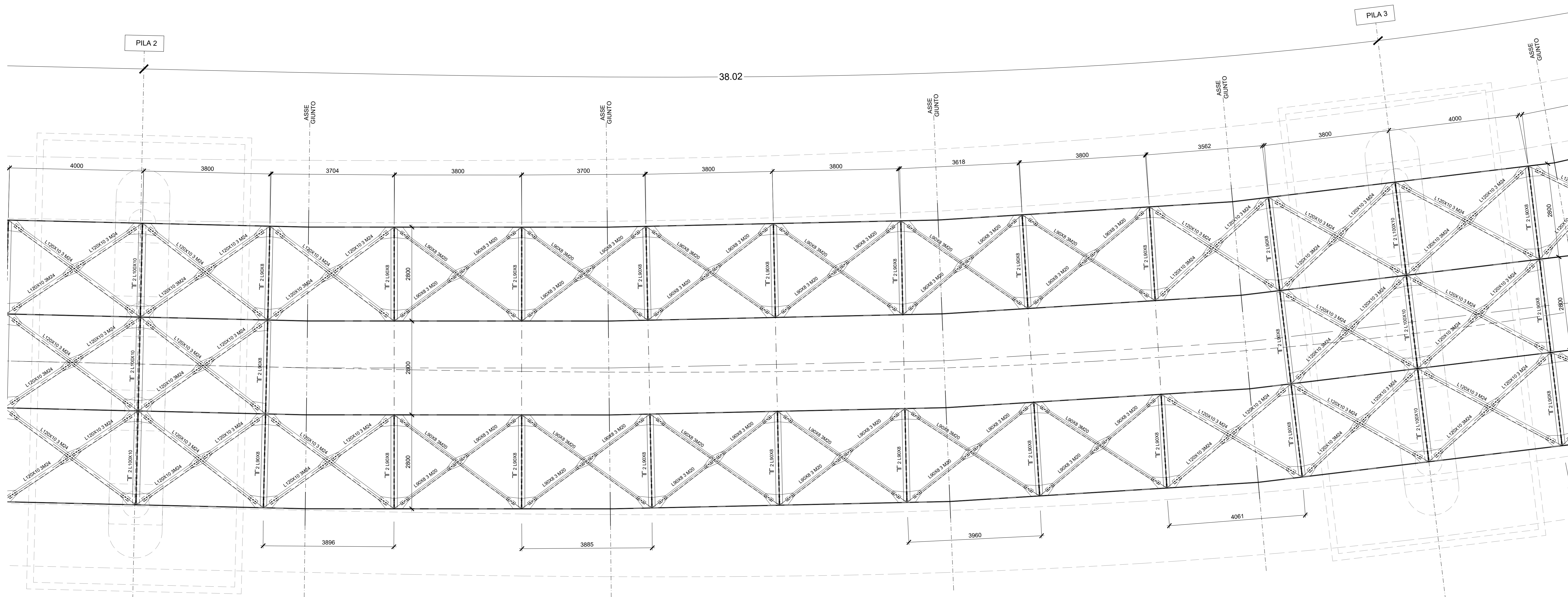
PIANTA CONTROVENTI INFERIORI - TRAVATA 3 Scala 1:50
