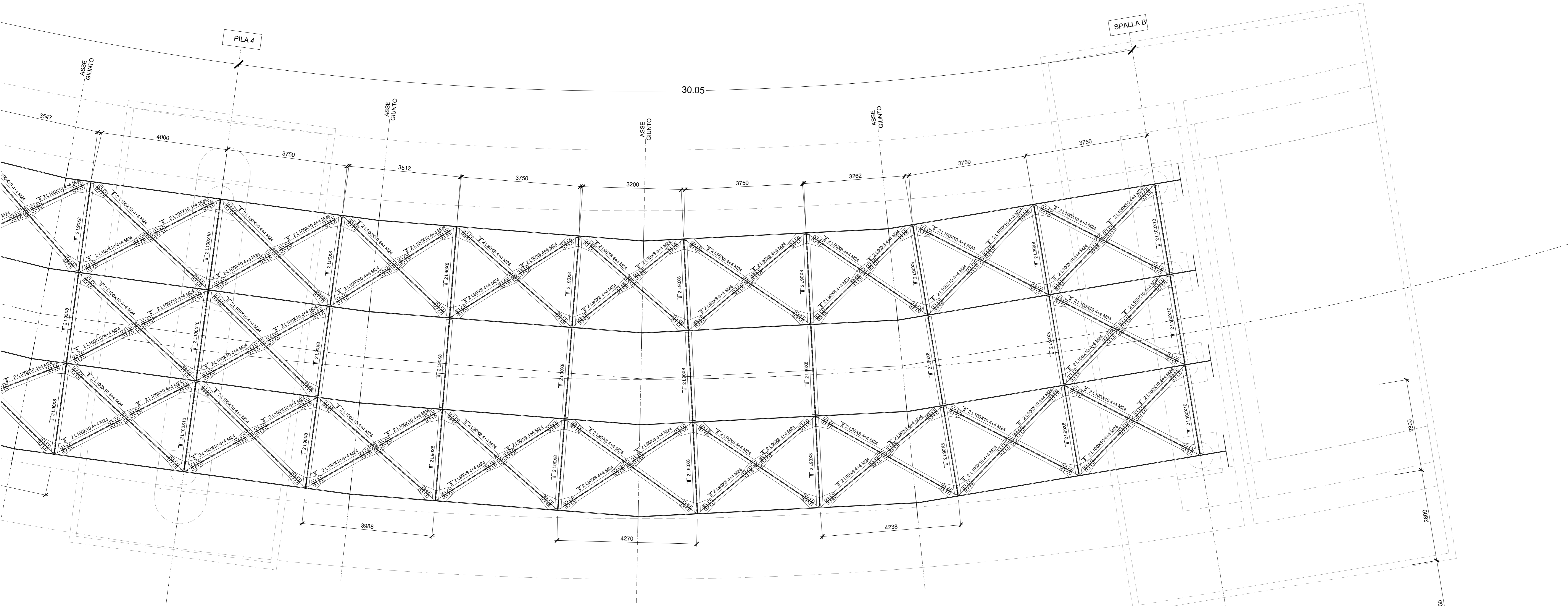
PIANTA CONTROVENTI INFERIORI - TRAVATA 5 Scala 1:50
