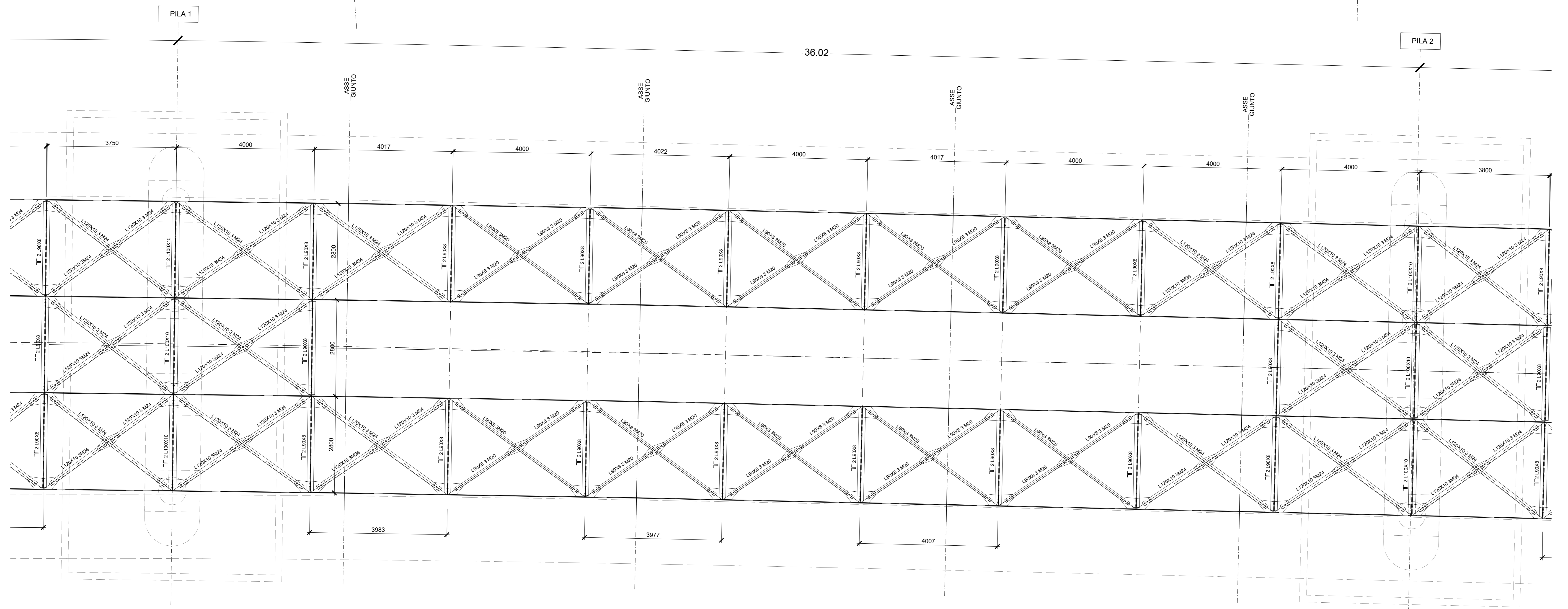
PIANTA CONTROVENTI SUPERIORI - TRAVATA 2 Scala 1:50
