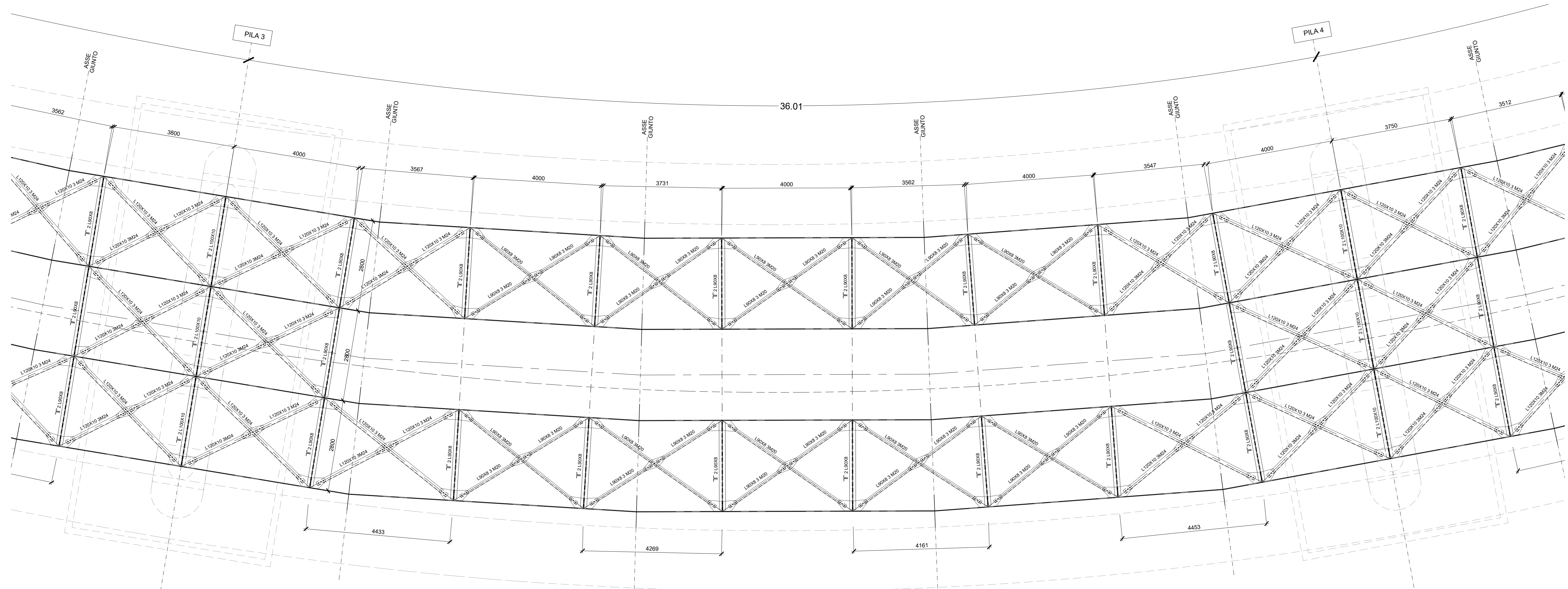
PIANTA CONTROVENTI SUPERIORI - TRAVATA 4 Scala 1:50
