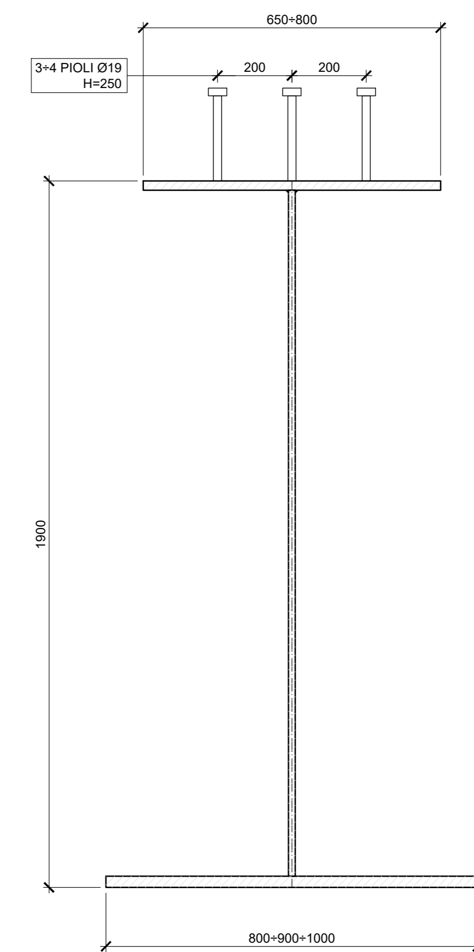
SEZIONE TIPO TRAVE PRINCIPALE Scala 1:10
