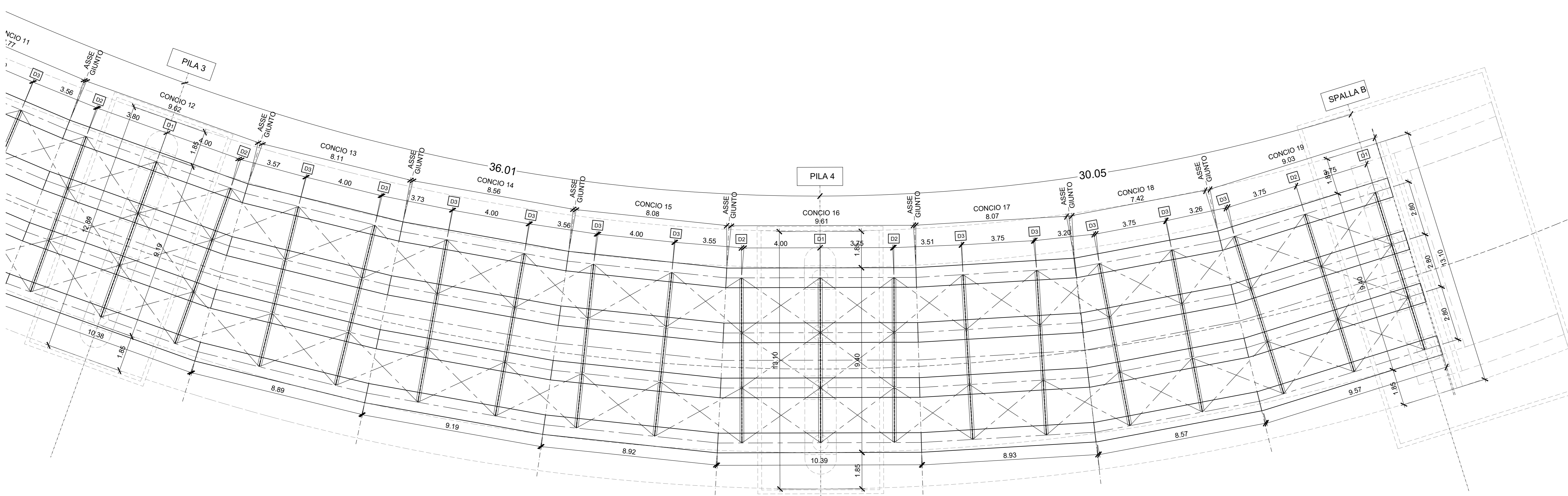
PIANTA TRAVI PRINCIPALI - TRAVATA 4 E 5 Scala 1:100
