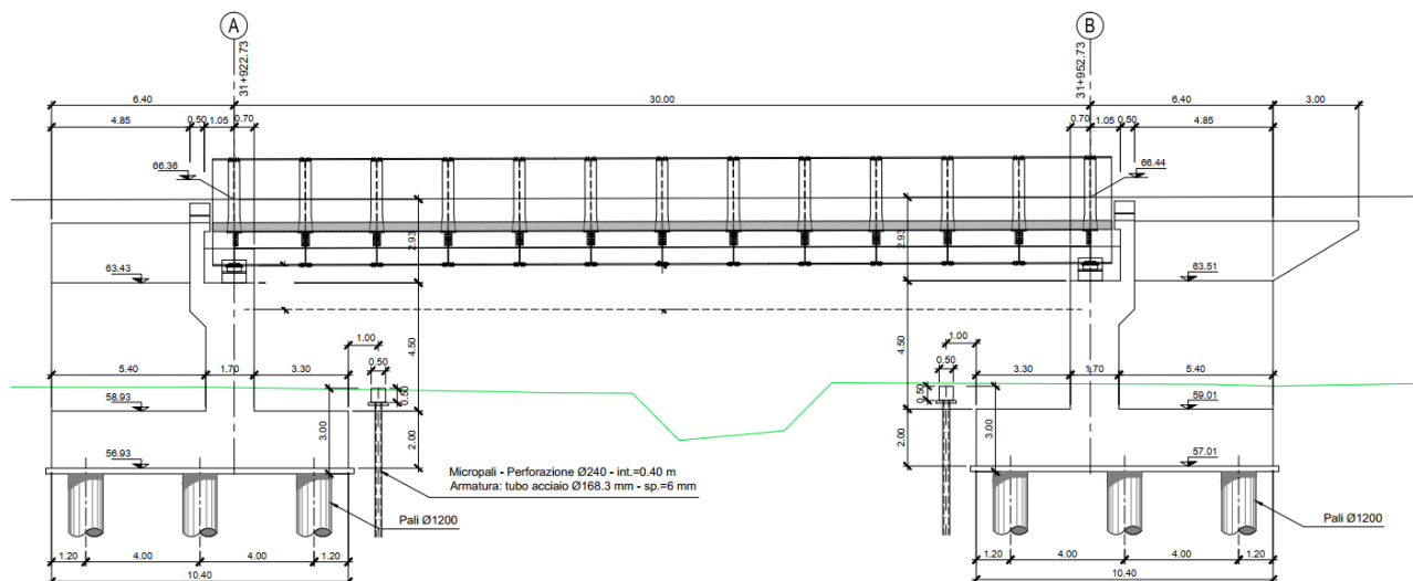
Figura 1 – Sezione Longitudinale Viadotto
