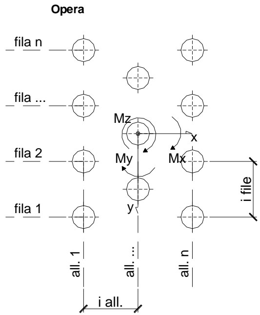
Disposizione Pali
