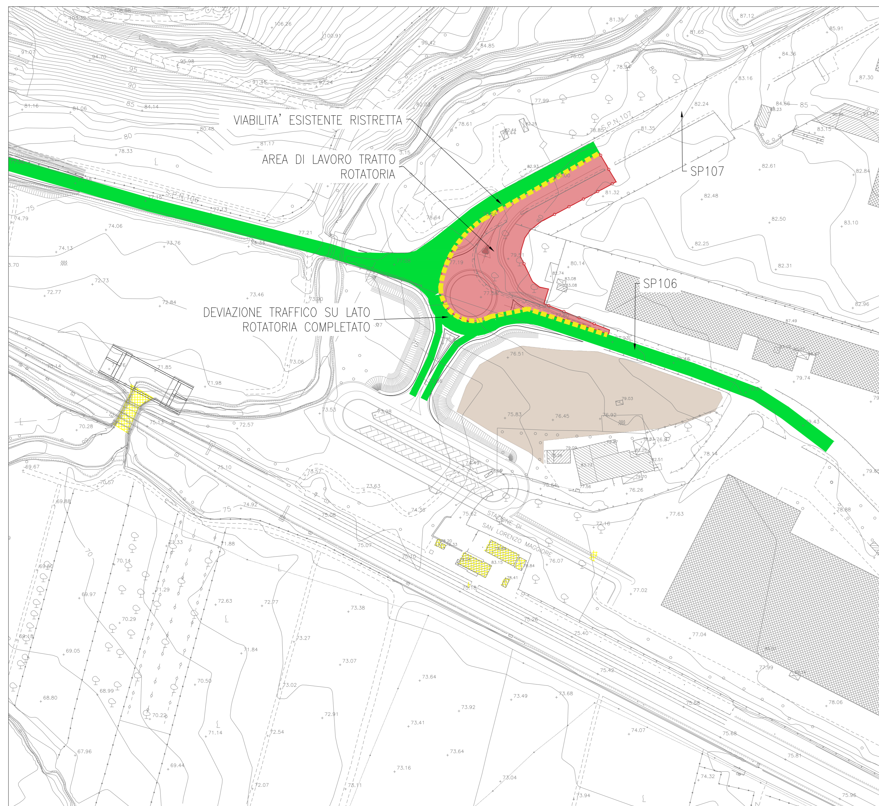
ROT. FERMATA S. LORENZO SCALA 1:1000 FASE2
