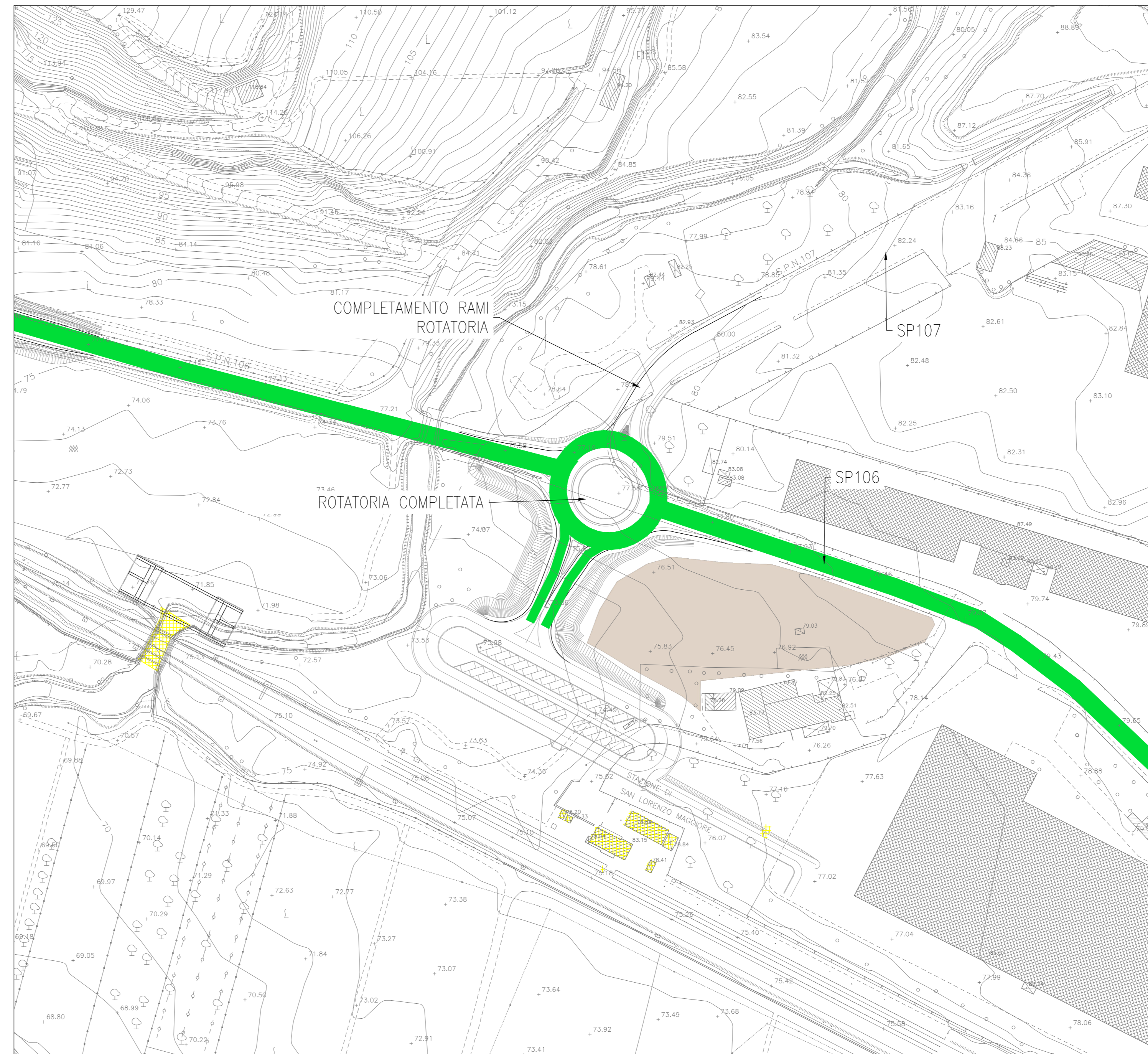
ROT. FERMATA S. LORENZO SCALA 1:1000 FASE3
