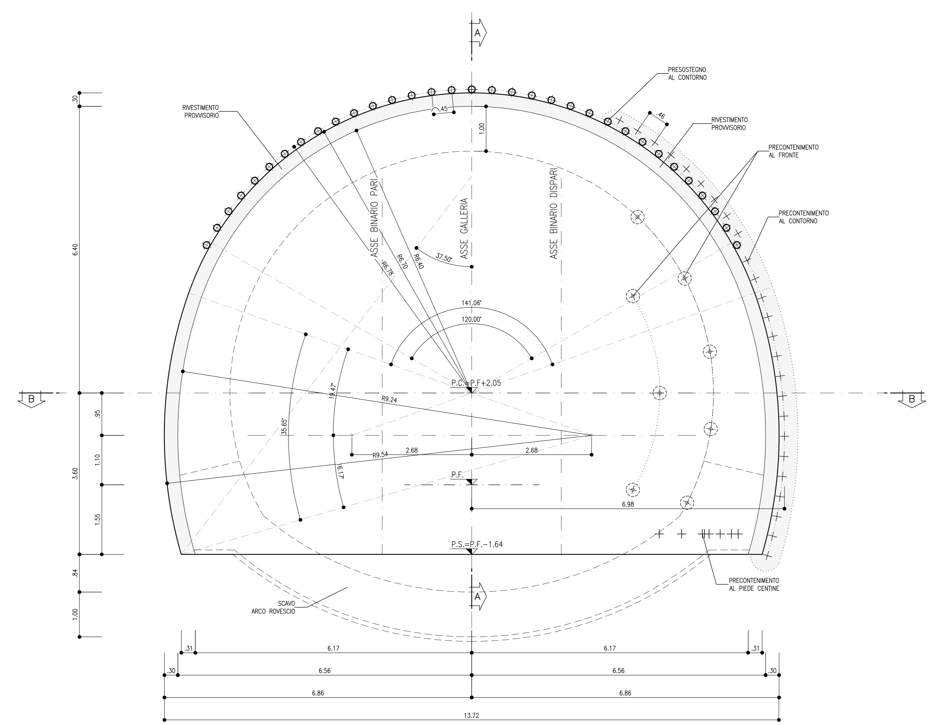
SEZIONE C-C SCALA 1:50 CONSOLIDAMENTI IN AVANZAMENTO
