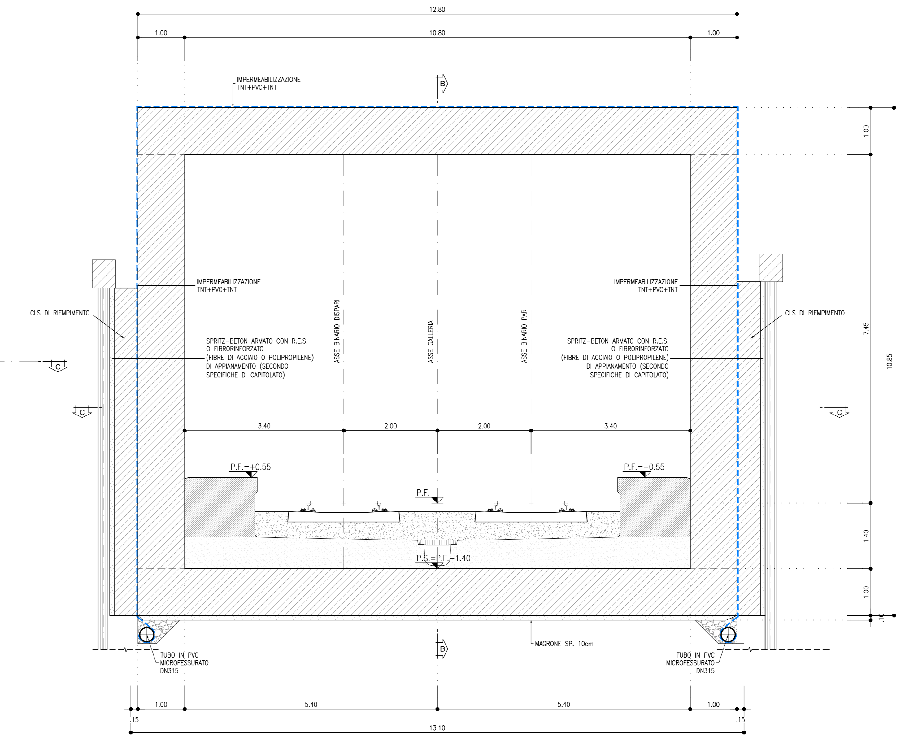
GALLERIA ARTIFICIALE SCATOLARE SCALA 1:50 SEZIONE A-A
