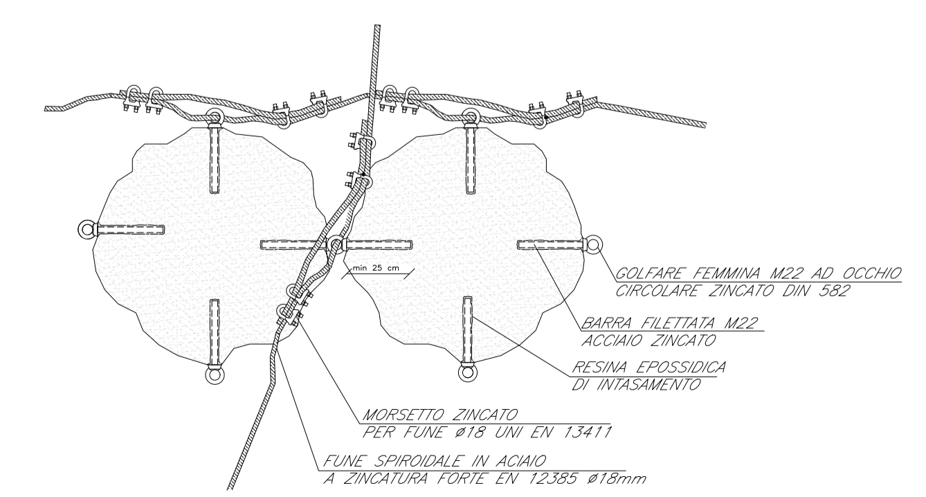
PARTICOLARE SPONDE RIVESTITE CON MASSI EMERGENTI LEGATI E INTASATI CON MATERIALE D'ALVEO MINIMO 80 cm PESO >700 Kg
