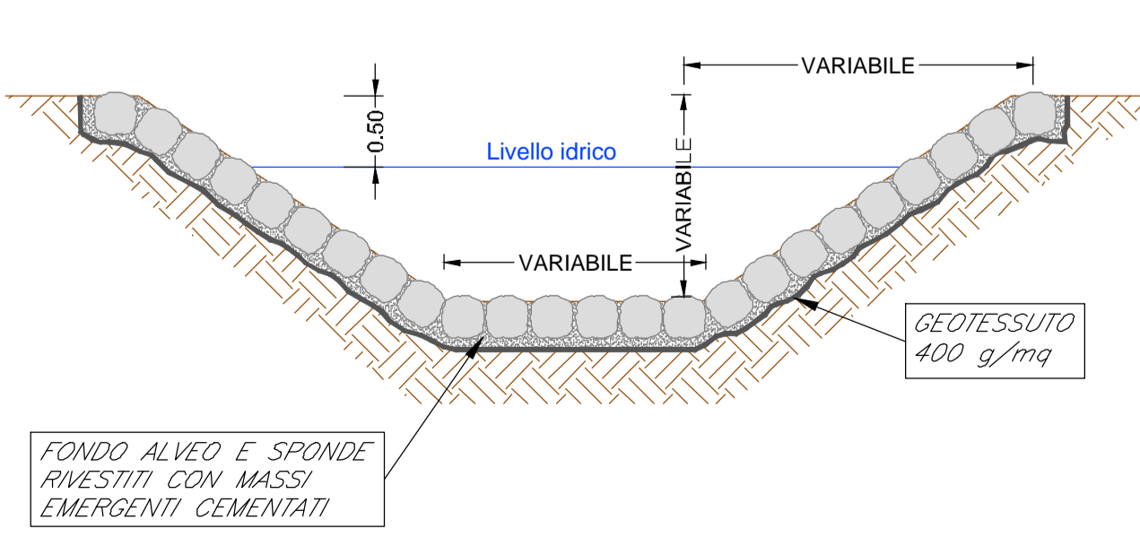
PARTICOLARE ALVEO RIVESTITO CON MASSI CEMENTATI
