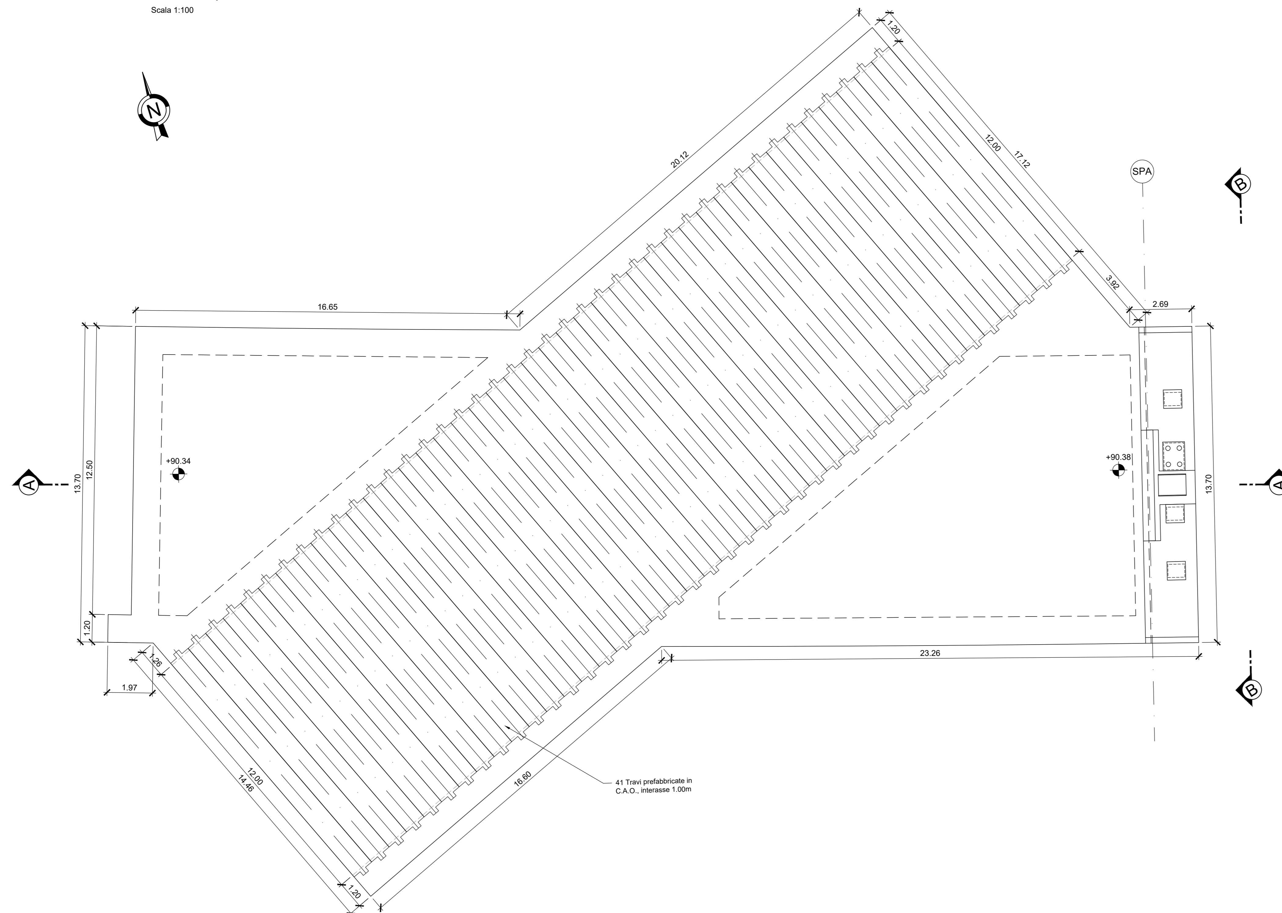
PIANTA QUOTA TRAVI Scala 1:100
