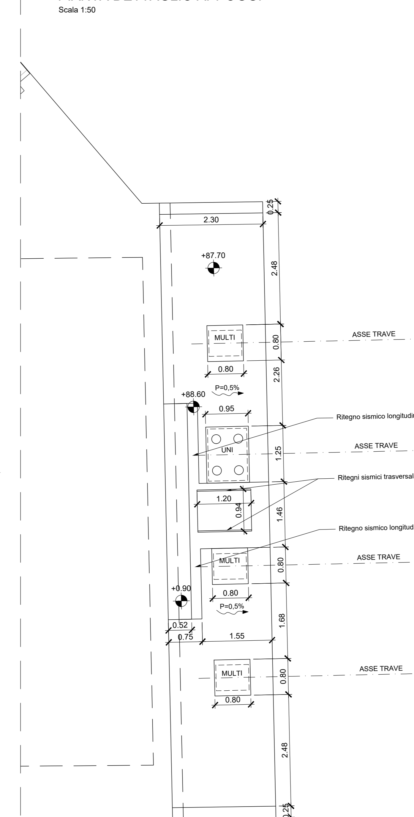
PIANTA DETTAGLIO APPOGGI Scala 1:50
