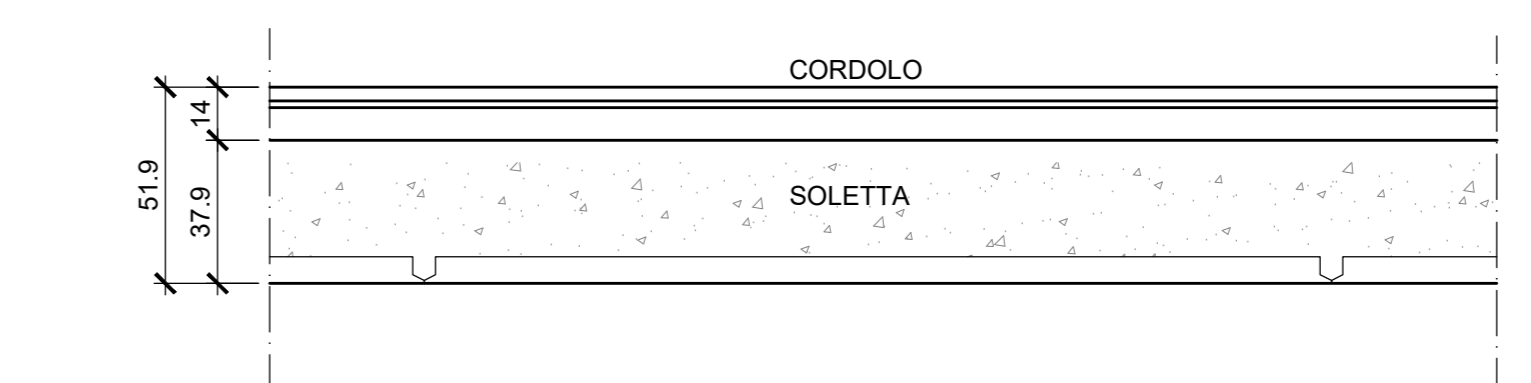
SEZIONE LONGITUDINALE B-B Scala 1:20
