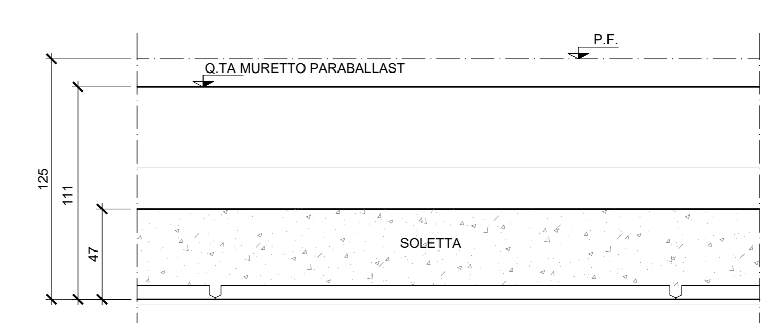
SEZIONE LONGITUDINALE A-A Scala 1:20
