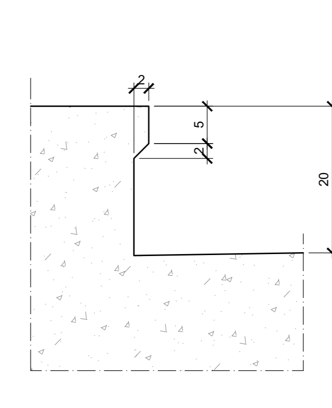
DETTAGLIO -1- CORDOLO Scala 1:5
