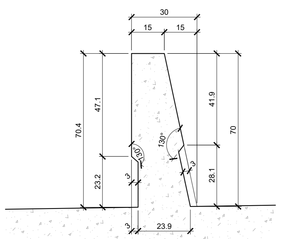
DETTAGLIO -2- CARPENTERIA MURETTO Scala 1:10
