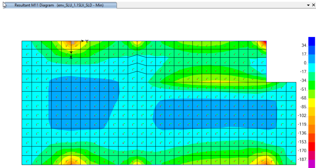
Figura 35: Diagramma momento flettente M_{11,min} ; comb. env_SLU/1.1SLV/SLD
