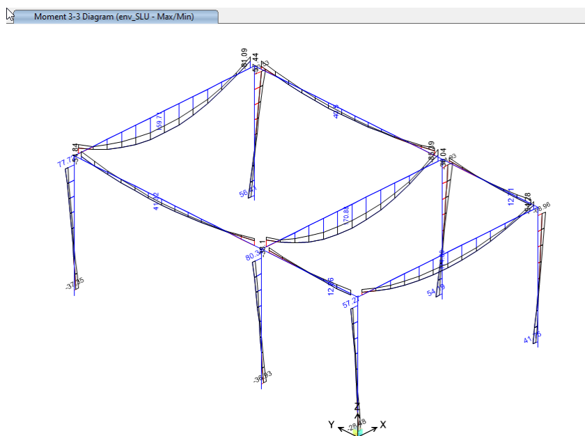
Figura 29: Diagramma momento flettente M3; comb. env_SLU
