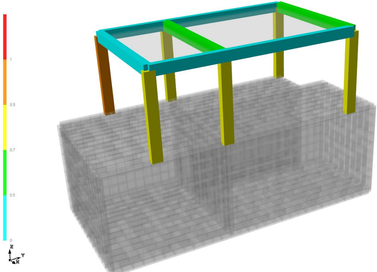
Figura 66: Struttura in elevazione; rapporti D/C verifiche di gerarchia a taglio, comb. SLV-SLD
