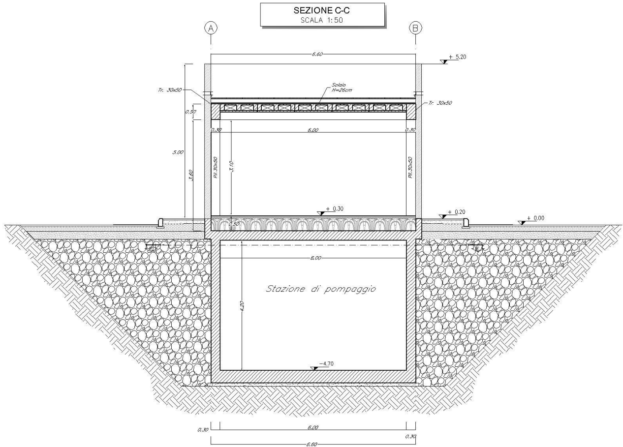
Figura 4: Sezione trasversale C-C
