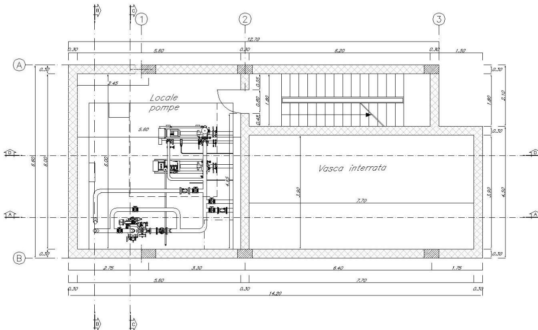
Figura 1: Carpenteria interrato - pianta
