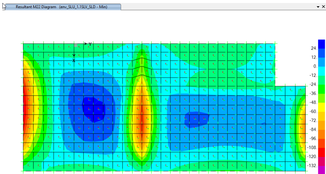
Figura 55: Diagramma momento flettente M22,min; comb. env_SLU/1.1SLV/SLD
