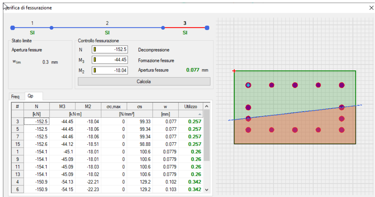
Figura 69: Verifica a fessurazione con rapporti D/C in comb. quasi permanente
