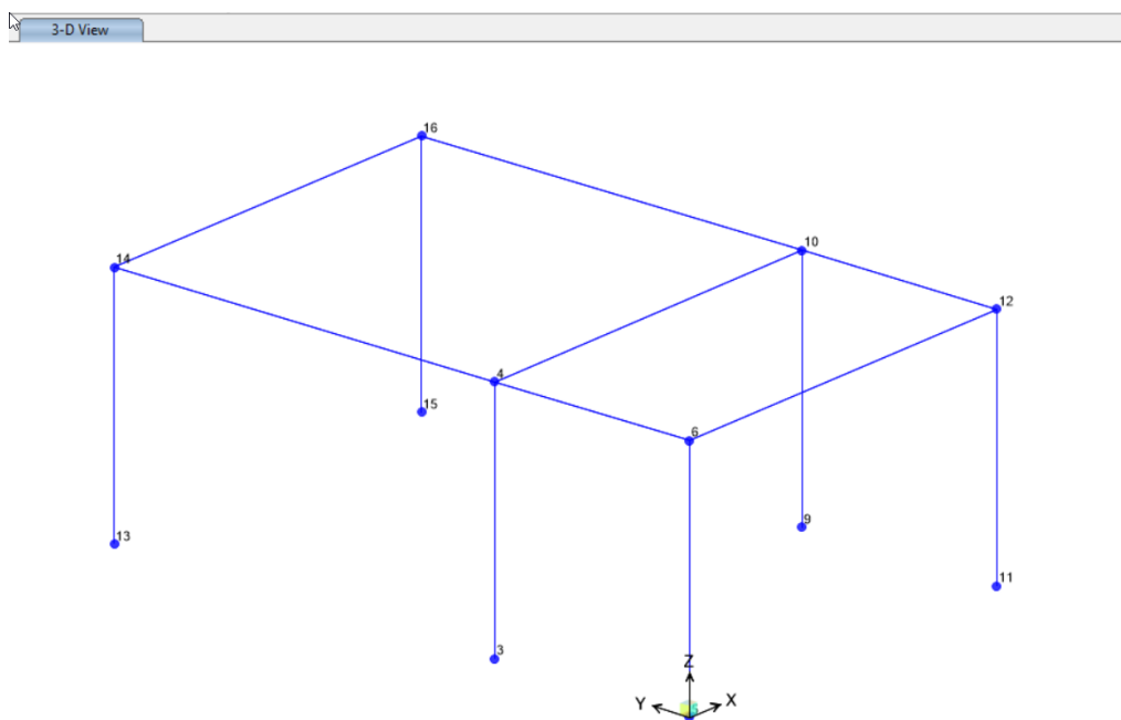
Figura 16: Modello di calcolo, numerazione nodi
