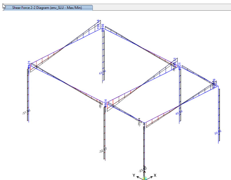
Figura 30: Diagramma forza di taglio V2; comb. env_SLU
