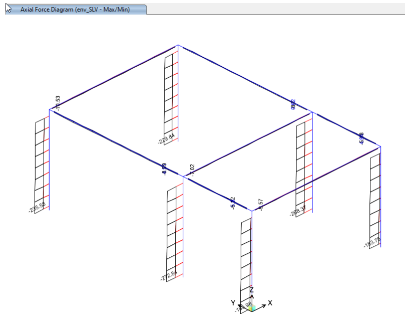
Figura 31: Diagramma sforzo normale N; comb. env_SLV
