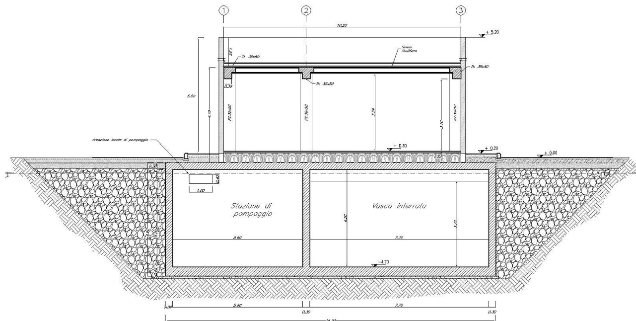
Figura 3: Sezione longitudinale
