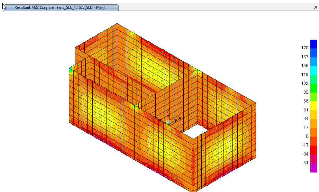
Figura 46: Diagramma momento flettente M_{22,max} ; comb. env_SLU/1.1SLV/SLD
