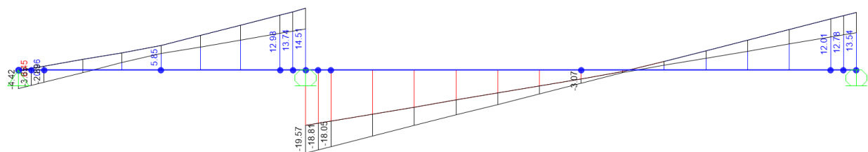
Figura 62: Diagramma forza di taglio V2 – involucro SLU [kNm]
