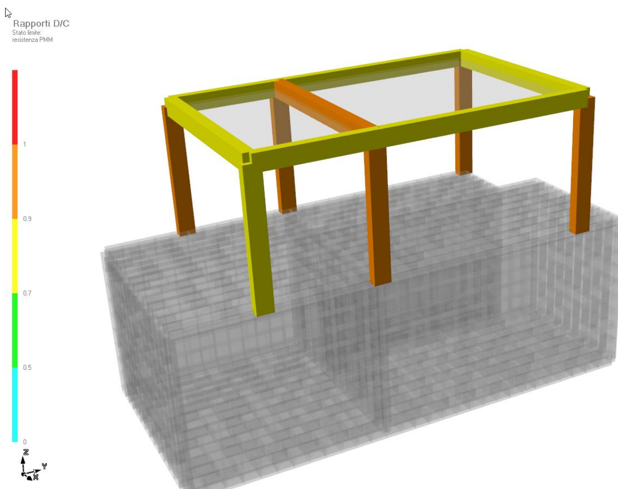
Figura 64: Struttura in elevazione; rapporti D/C verifiche PMM, comb. SLU-SLV-SLD
