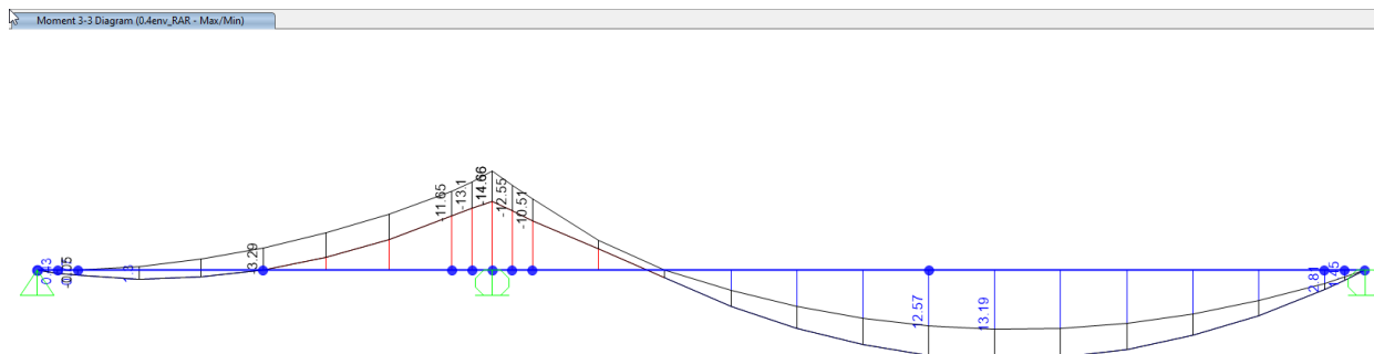
Figura 63: Diagramma momento flettente M3 – involuppo SLE-rara [kNm]
