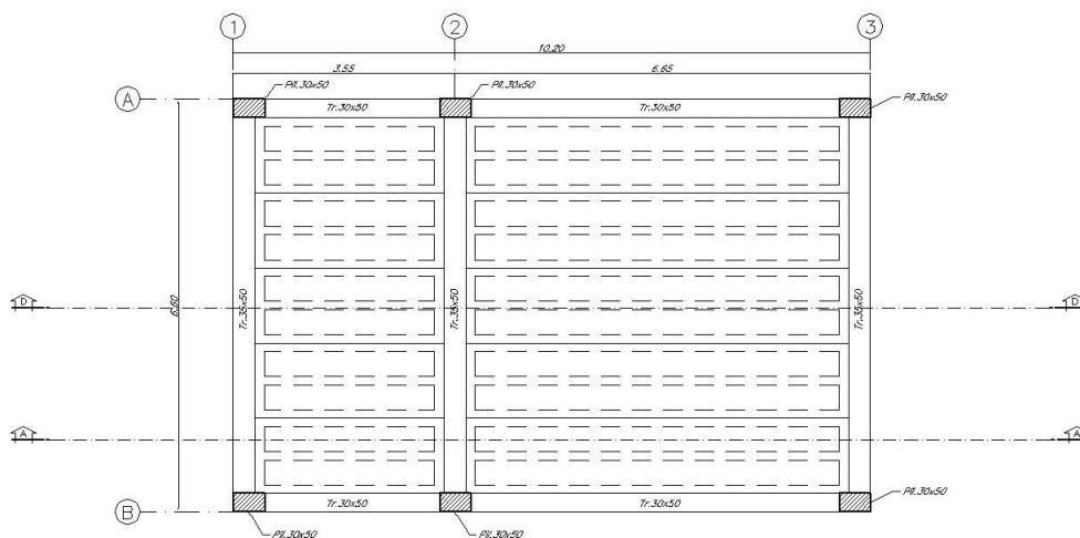
Figura 2: Carpenteria piano copertura
