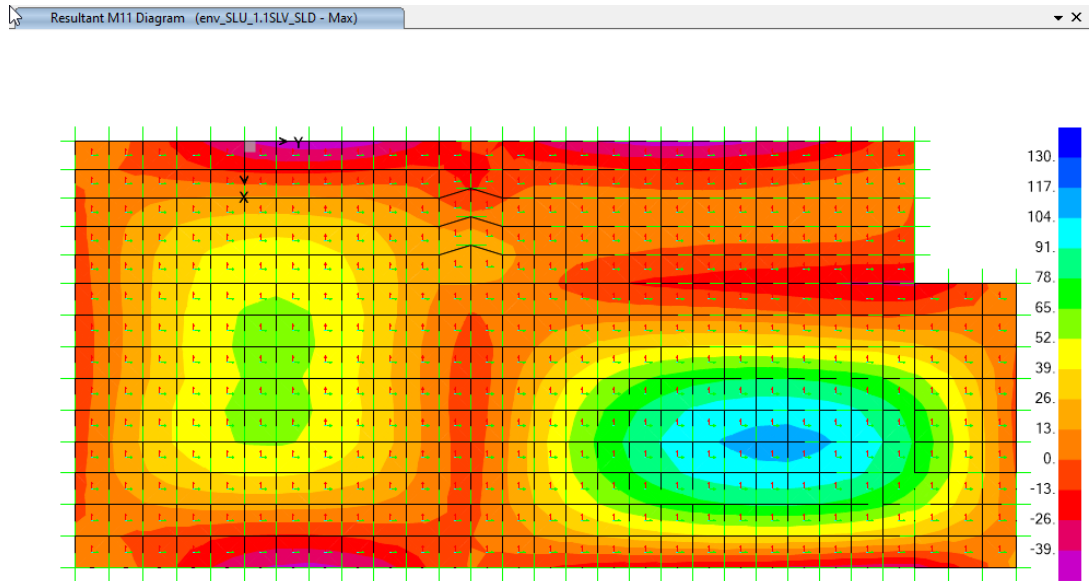
Figura 52: Diagramma momento flettente M11,max; comb. env_SLU/1.1SLV/SLD
