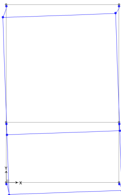
Figura 27: Forma modale 2 ; vista in pianta
