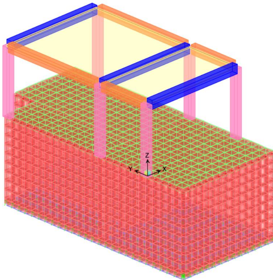
Figura 15: Modello di calcolo, vista assometrica elementi estrusi
