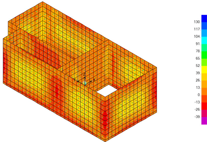
Figura 43: Diagramma momento flettente M11,max; comb. env_SLU/1.1SLV/SLD
