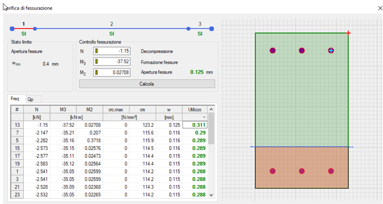
Figura 72: Verifica a fessurazione con rapporti D/C in comb. frequenti
