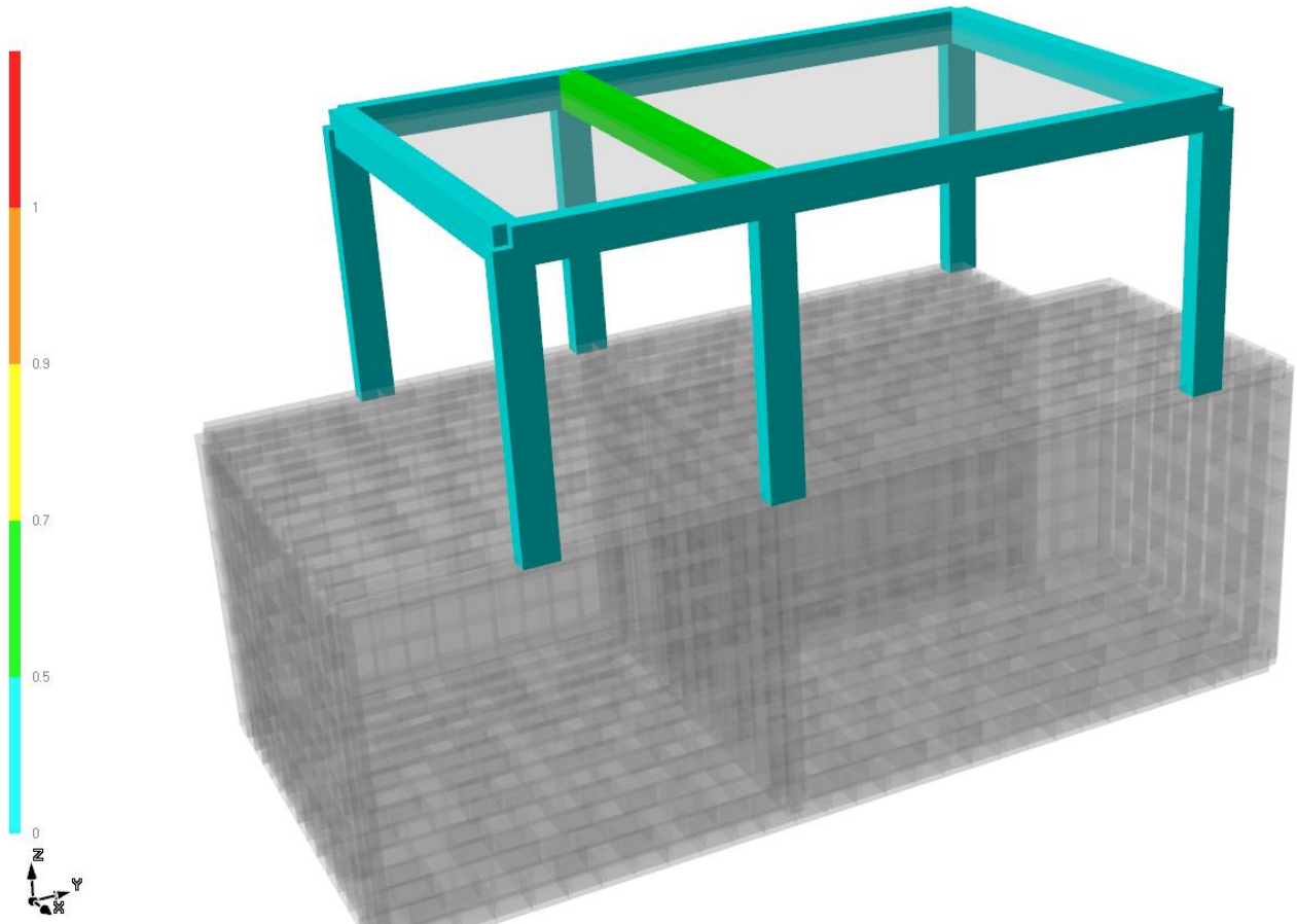
Figura 65: Struttura in elevazione; rapporti D/C verifiche a taglio, comb. SLU-SLV-SLD
