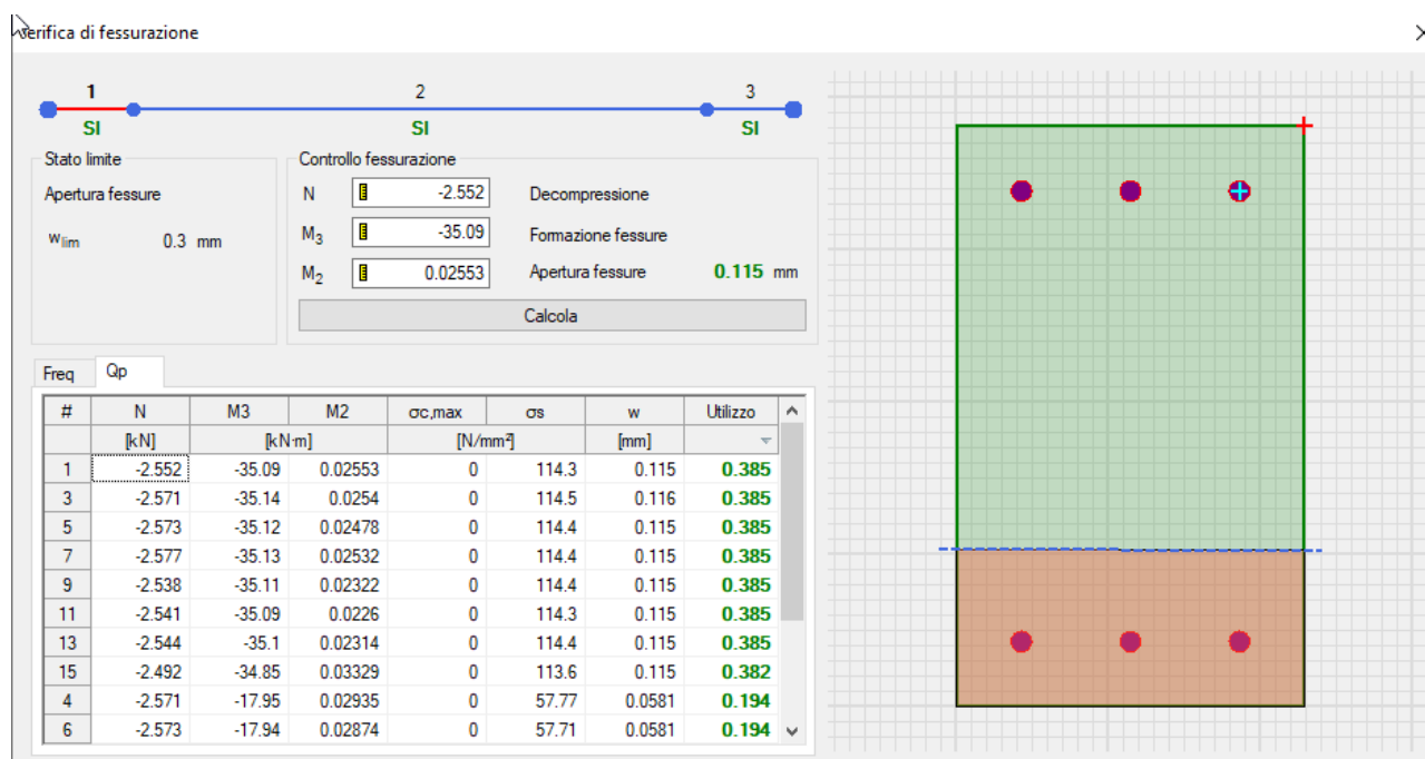
Figura 73: Verifica a fessurazione con rapporti D/C in comb. quasi permanente
