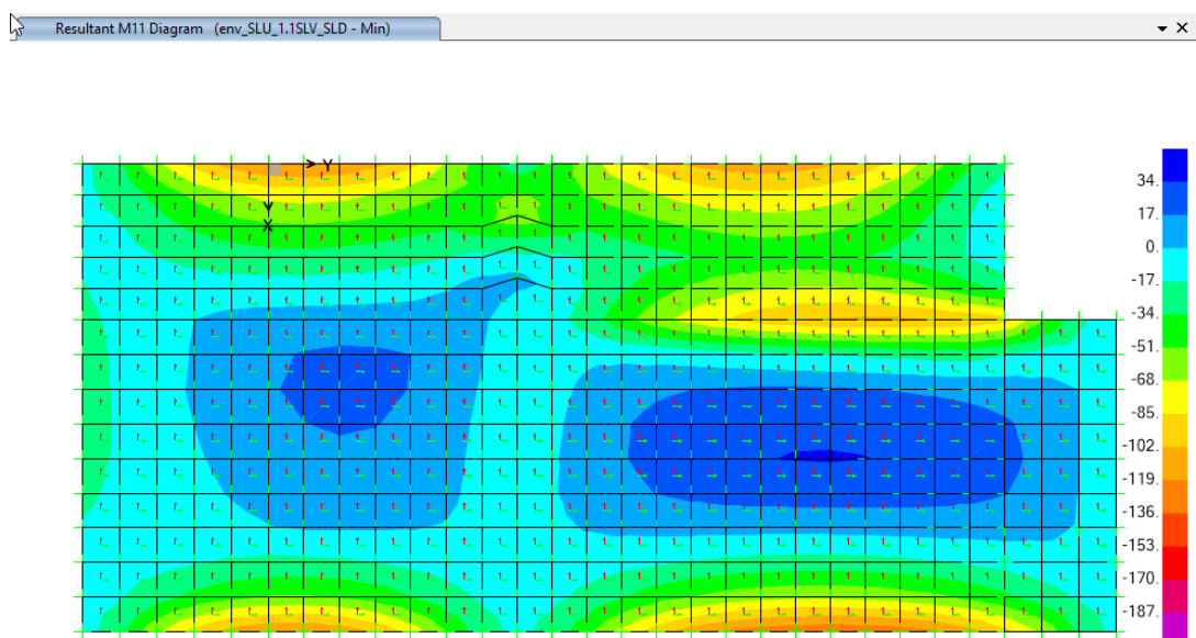
Figura 53: Diagramma momento flettente M11,min; comb. env_SLU/1.1SLV/SLD
