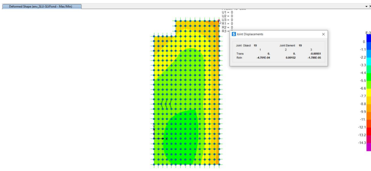
Figura 74: Diagramma involuppo spostamenti nodi fondazione; comb. env_SLU/SLV
