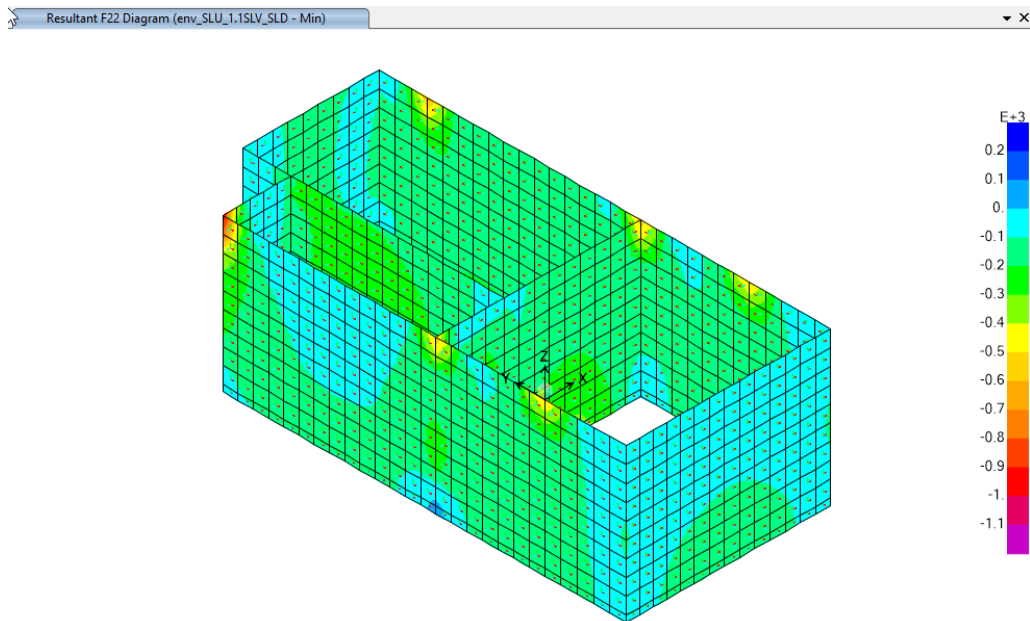
Figura 45: Diagramma sforzo normale N_{22,min} ; comb. env_SLU/1.1SLV/SLD
