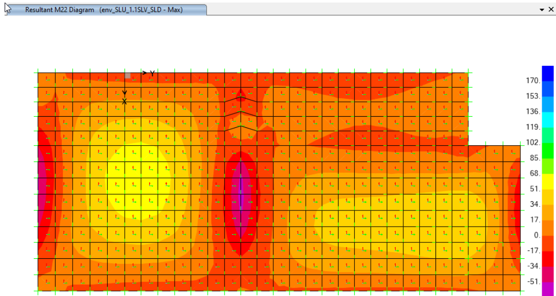
Figura 54: Diagramma momento flettente M22,max; comb. env_SLU/1.1SLV/SLD
