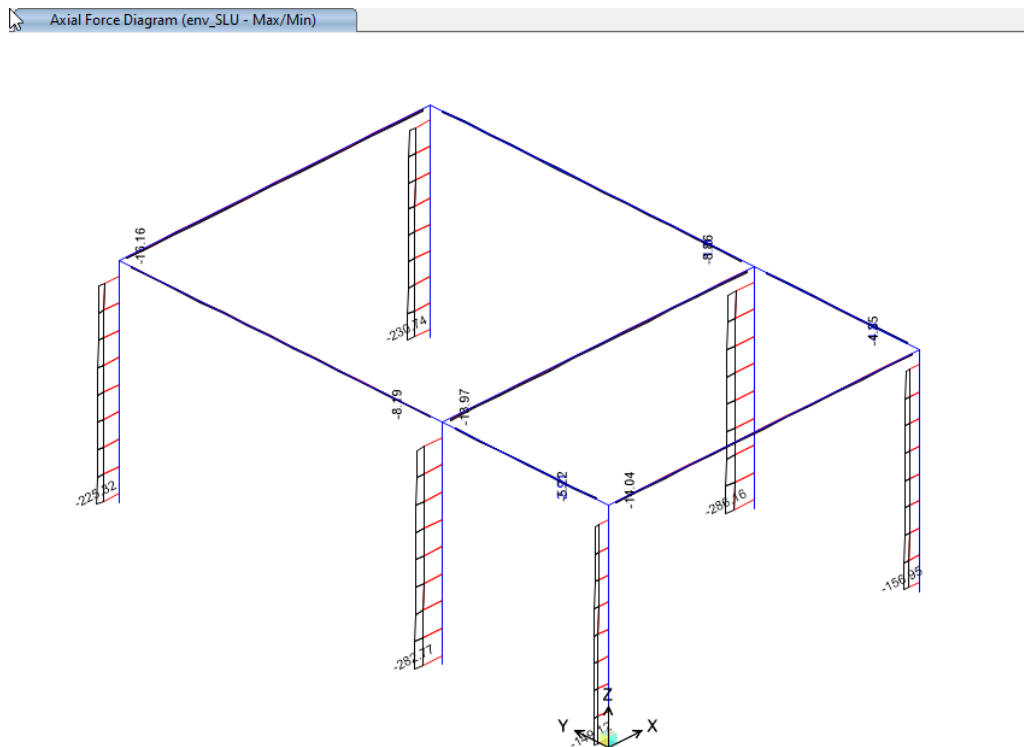
Figura 28: Diagramma sforzo normale N; comb. env_SLU
