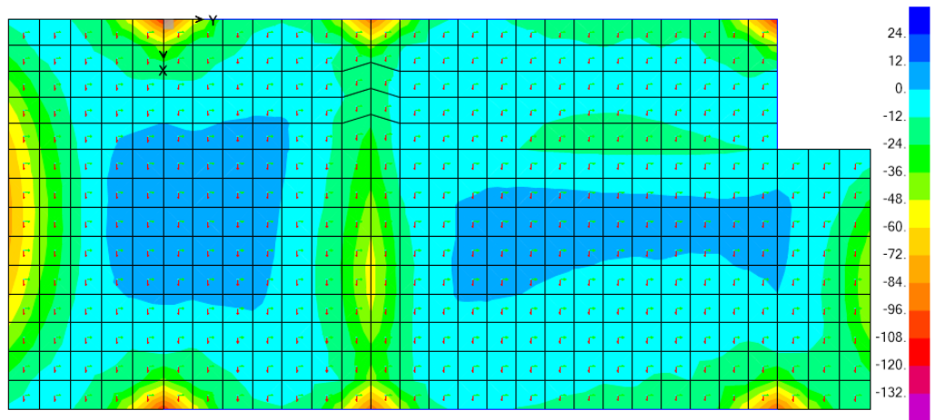
Figura 37: Diagramma momento flettente M22,min; comb. env_SLU/1.1SLV/SLD
