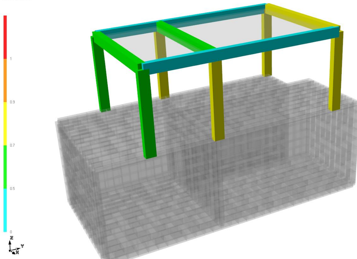
Figura 67: Struttura in elevazione; rapporti D/C verifiche tensionali in esercizio
