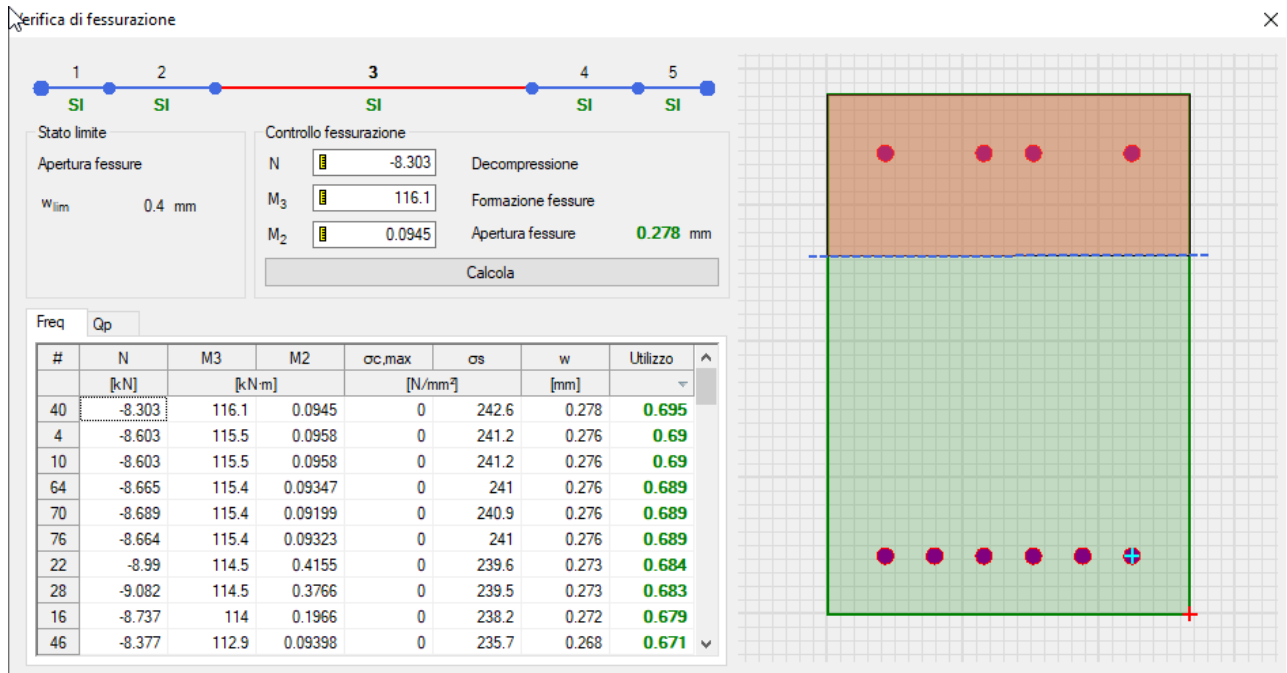
Figura 70: Verifica a fessurazione con rapporti D/C in comb. frequenti
