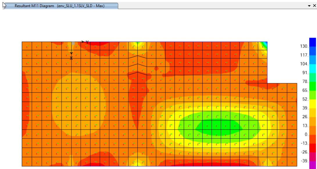
Figura 34: Diagramma momento flettente M11,max; comb. env_SLU/1.1SLV/SLD
