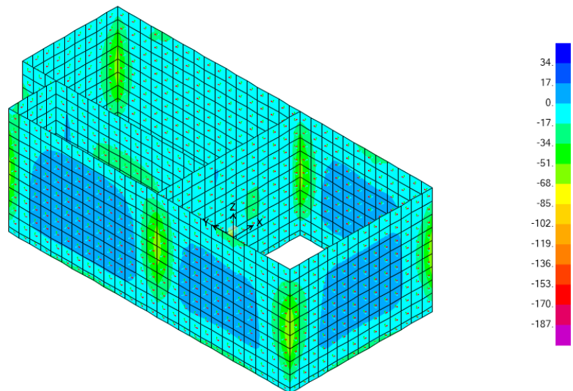
Figura 44: Diagramma momento flettente M11,min; comb. env_SLU/1.1SLV/SLD
