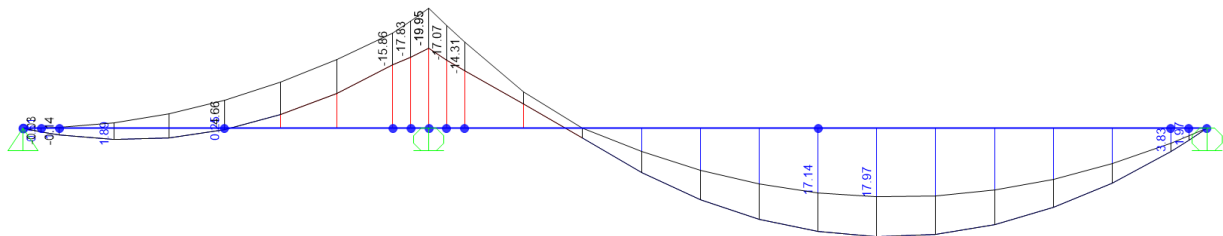
Figura 61: Diagramma momento flettente M3 – involucro SLU [kNm]
