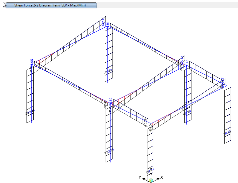
Figura 33: Diagramma forza di taglio V2; comb. env_SLV
