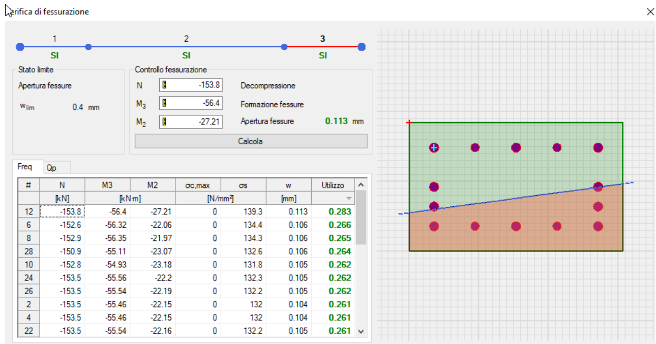
Figura 68: Verifica a fessurazione con rapporti D/C in comb. frequenti
