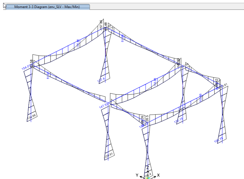
Figura 32: Diagramma momento flettente M3; comb. env_SLV
