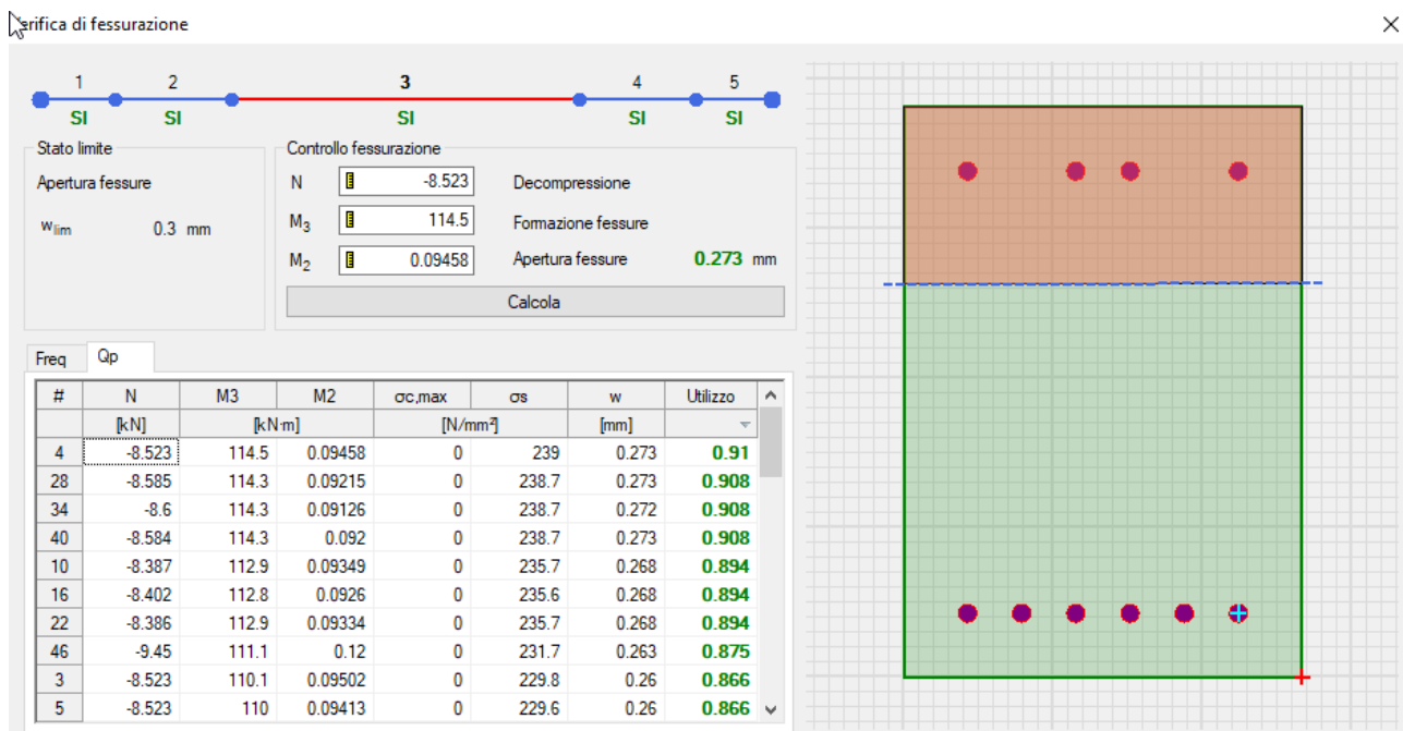
Figura 71: Verifica a fessurazione con rapporti D/C in comb. quasi permanente
