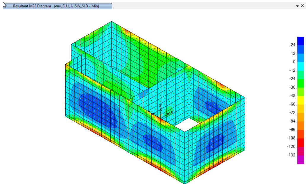
Figura 47: Diagramma momento flettente M22,min; comb. env_SLU/1.1SLV/SLD
