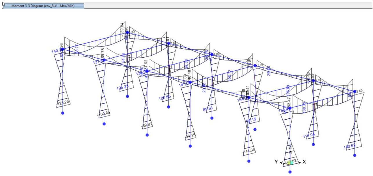
Figura 33: Diagramma momento flettente M3; comb. env_SLV
