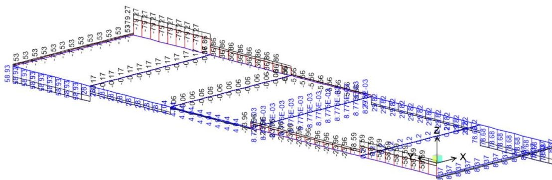
Figura 37: Diagramma momento torcente T; comb. env_SLU
