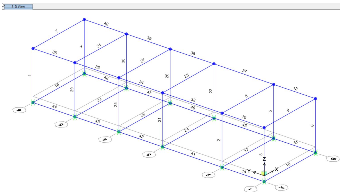
Figura 17: Modello di calcolo, numerazione aste
