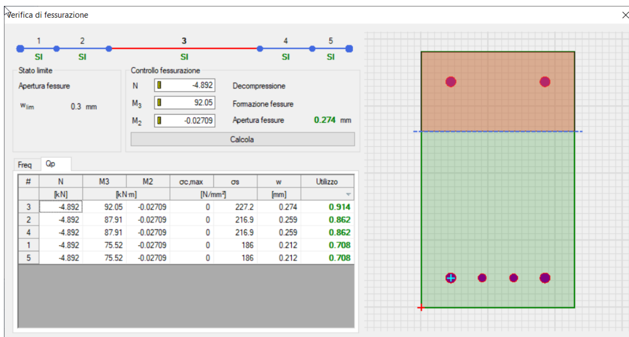
Figura 52: Verifica a fessurazione con rapporti D/C in comb. quasi permanente
