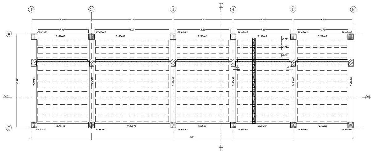
Figura 2: Carpenteria piano copertura
