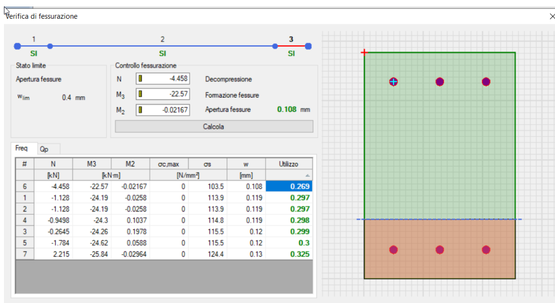
Figura 55: Verifica a fessurazione con rapporti D/C in comb. frequenti
