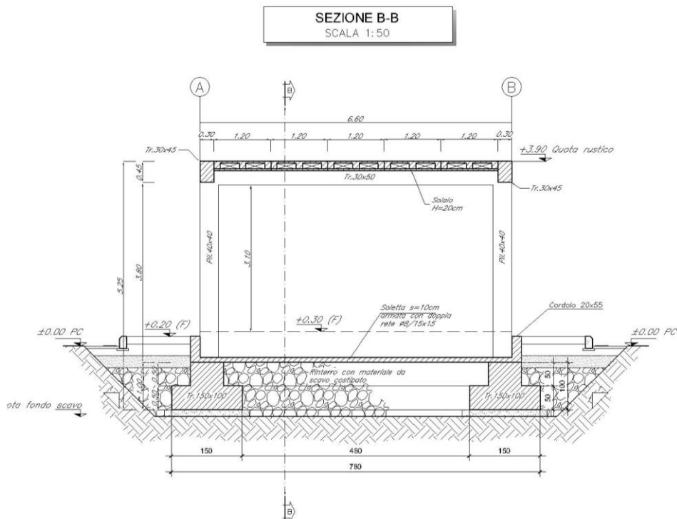
Figura 4: Sezione trasversale
