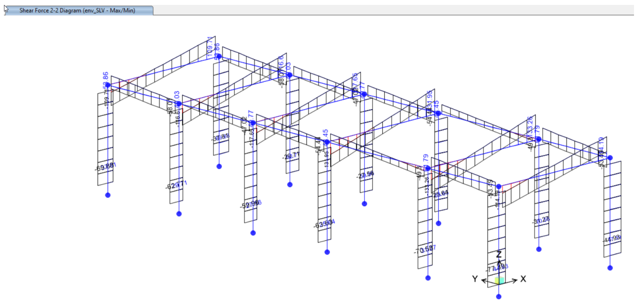
Figura 34: Diagramma forza di taglio V2; comb. env_SLV
