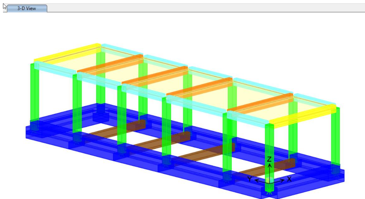
Figura 15: Modello di calcolo, vista assonometrica elementi estrusi
