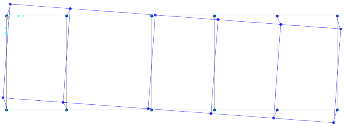
Figura 27: Forma modale 2 ; vista in pianta
