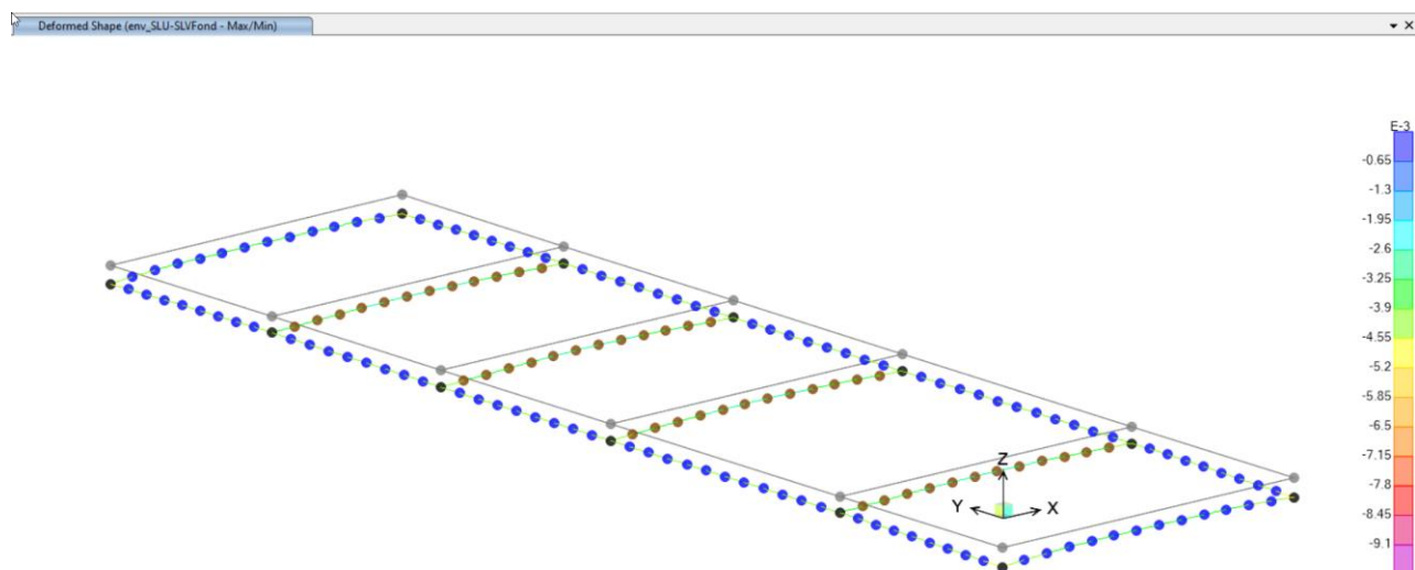
Figura 57: Diagramma involucro spostamenti nodi fondazione; comb. env_SLU/SLV
