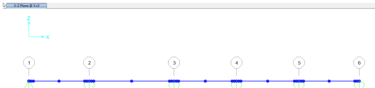
Figura 41: Schema statico solaio copertura
