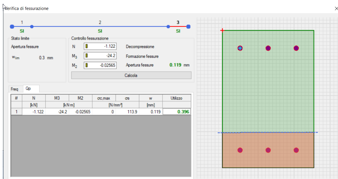
Figura 56: Verifica a fessurazione con rapporti D/C in comb. quasi permanente
