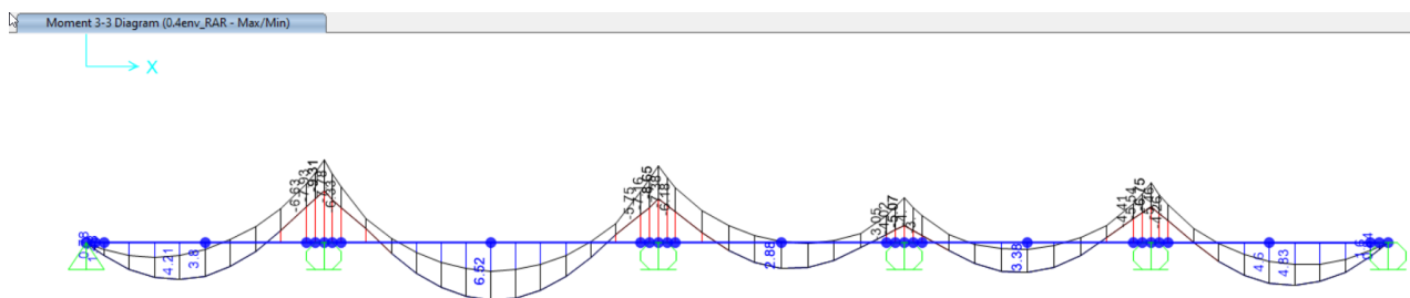
Figura 44: Diagramma momento flettente M3 – involuppo SLE-rara [kNm]
