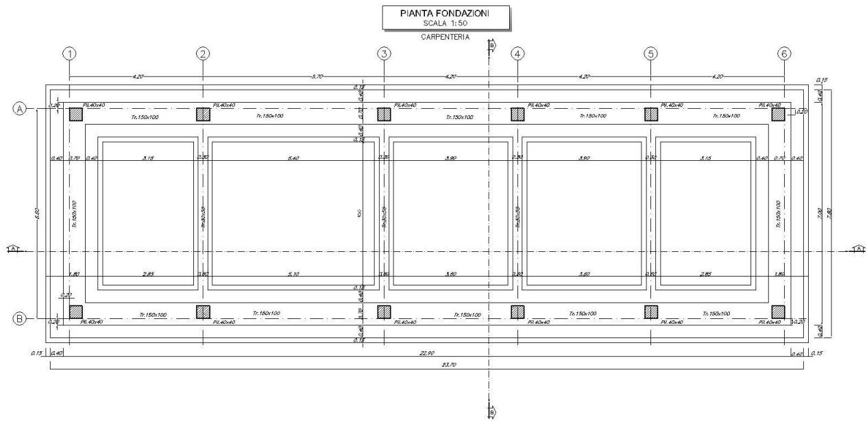
Figura 1: Carpenteria fondazione
