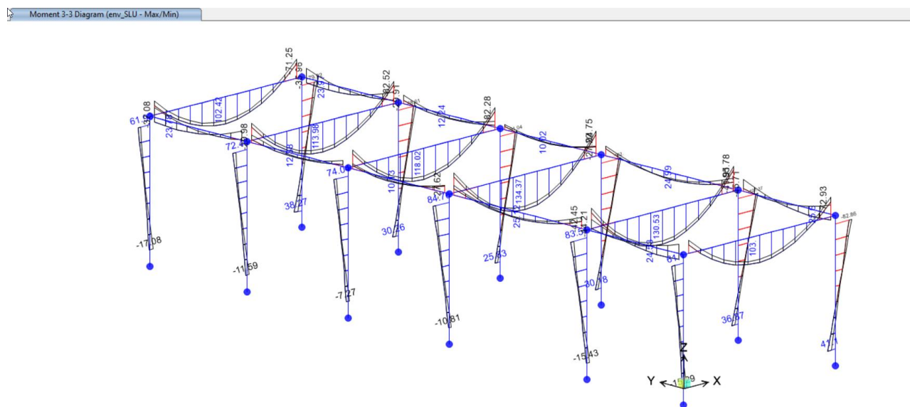
Figura 30: Diagramma momento flettente M3; comb. env_SLU
