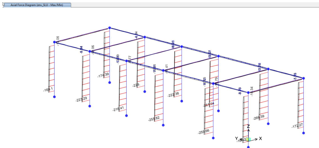
Figura 29: Diagramma sforzo normale N; comb. env_SLU
