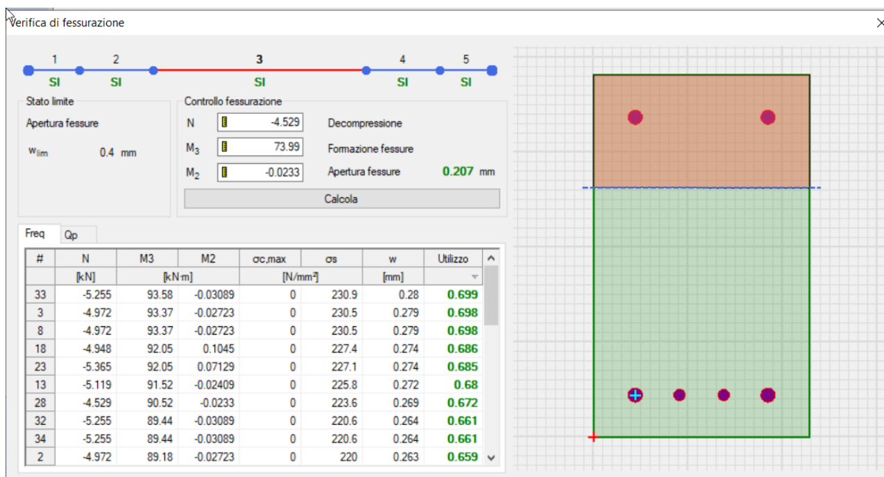
Figura 51: Verifica a fessurazione con rapporti D/C in comb. frequenti
