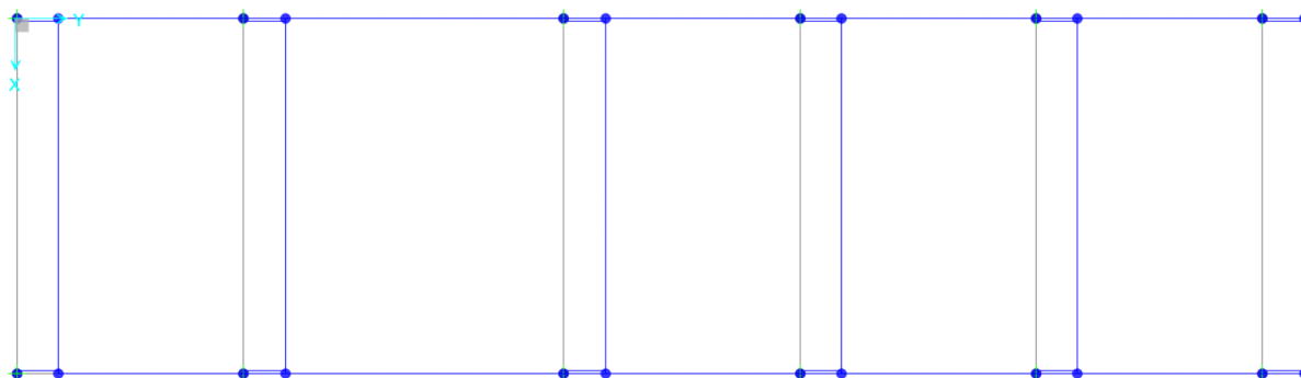
Figura 28: Forma modale 3 (dir. Y); vista in pianta
