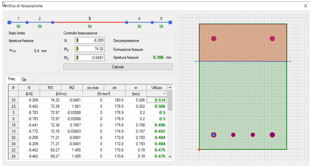
Figura 53: Verifica a fessurazione con rapporti D/C in comb. frequenti
