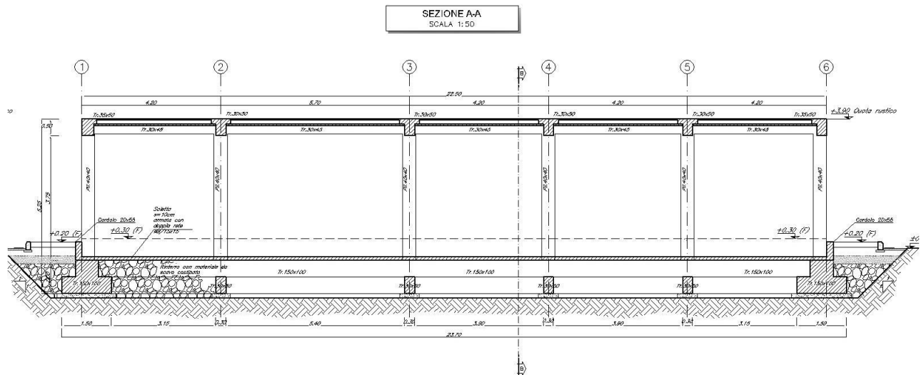
Figura 3: Sezione longitudinale
