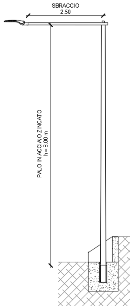
Fig2. Palo di illuminazione in trincea
