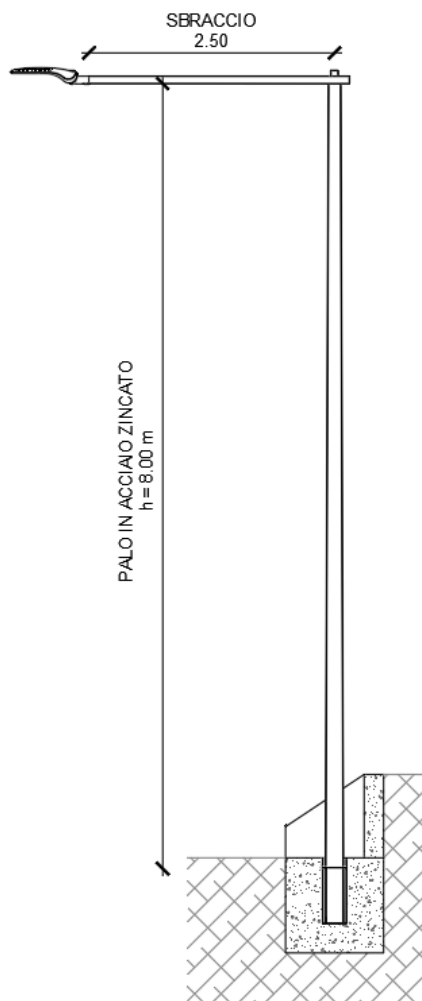
Fig2. Palo di illuminazione in trincea
