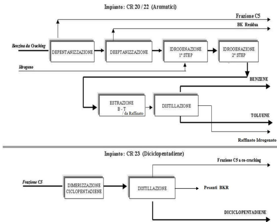
Figura III.2 - Schema a blocchi semplificato dell'impianto CR20-23
