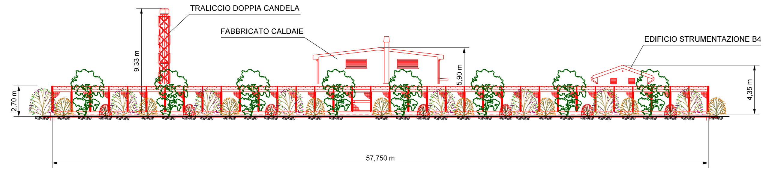
PROSPETTO B
