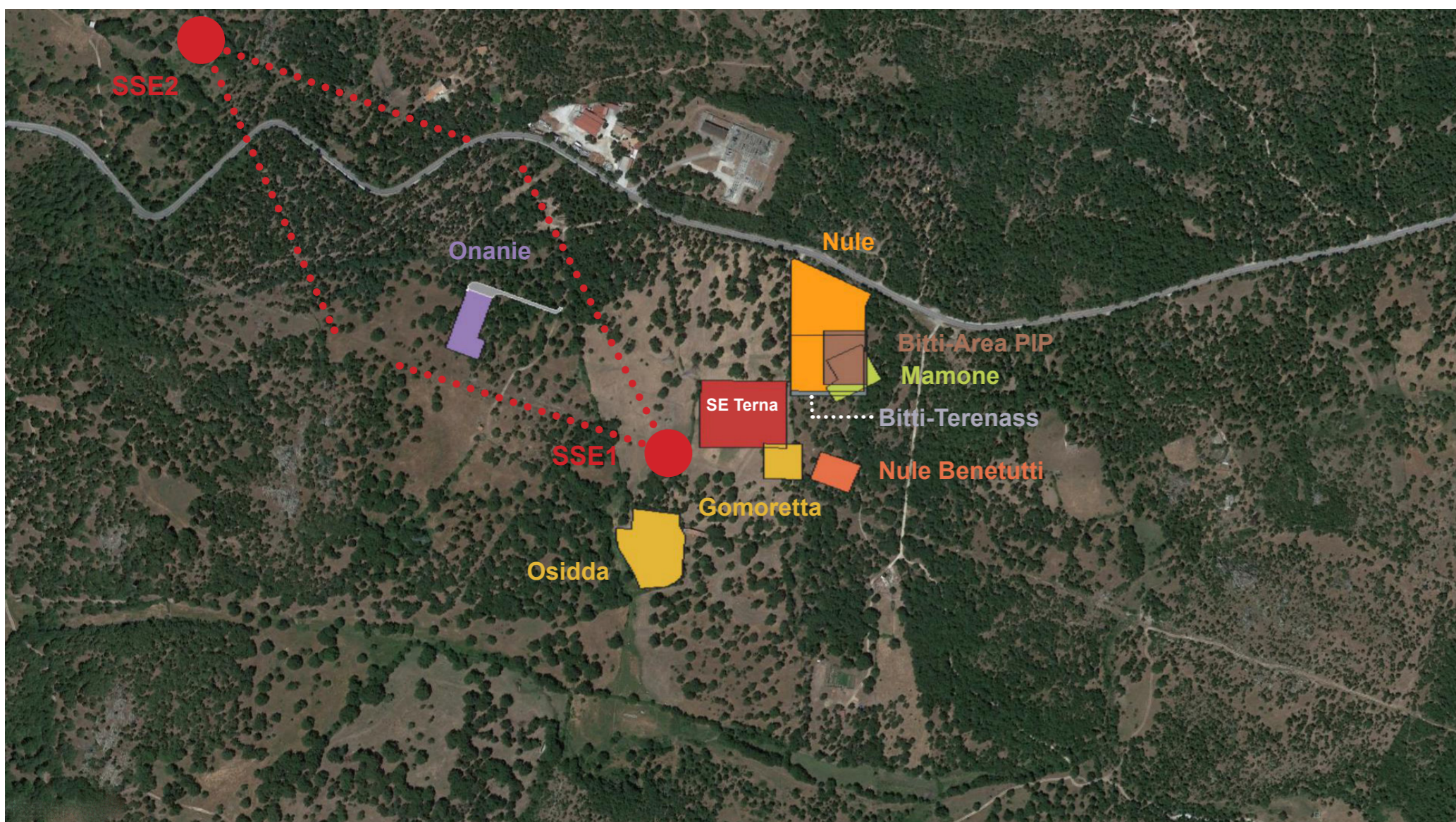
Inquadramento territoriale e cono visivo del progetto in proposta e delle SSE utente dei progetti eolici esistenti o in istruttoria
