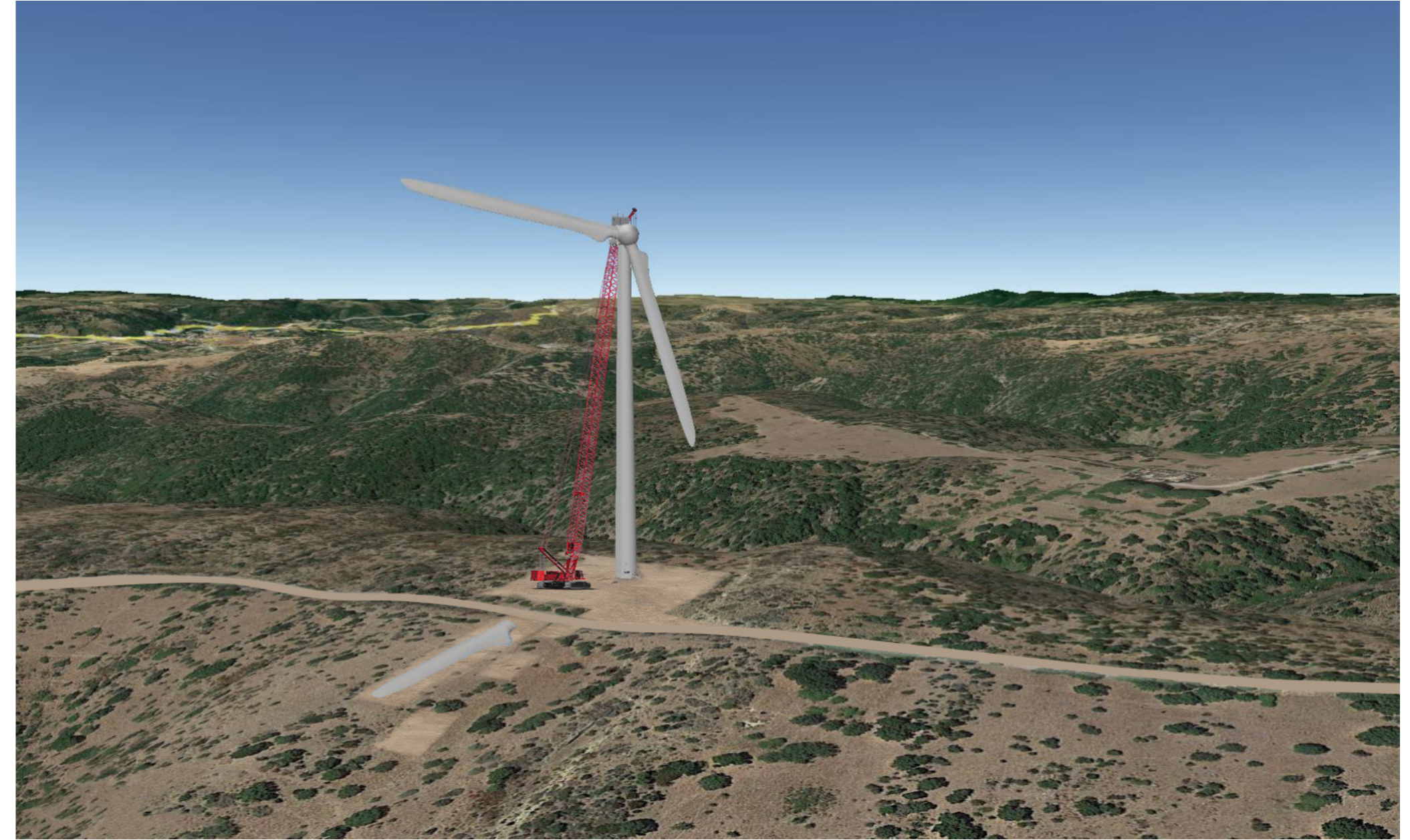
Rendering - piazzole temporanee e di cantiere
