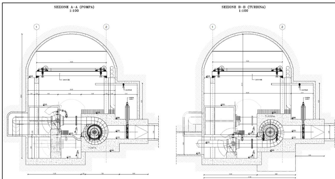
Figura 10 – Sezione della centrale in asse pompa (sx) e turbina (dx)
