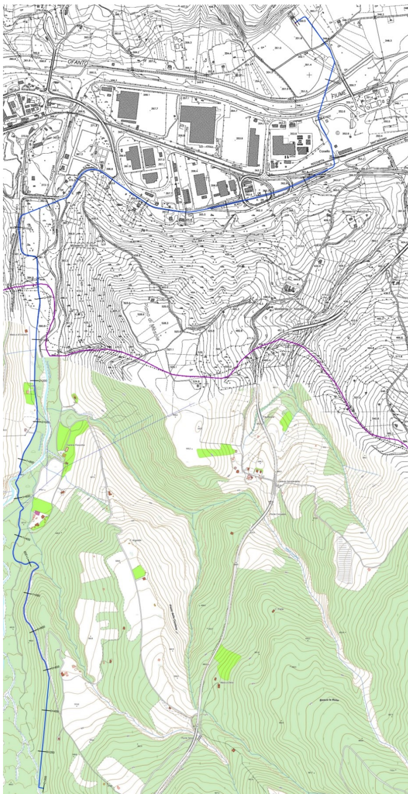
Figura 16: stralcio della corografia di progetto su CTR (in blu il tracciato del cavo interrato)
