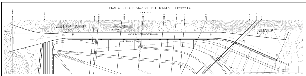
Figura 12 – Pianta della Deviazione del Torrente Ficocchia (Monte a Sx, Valle a Dx)
