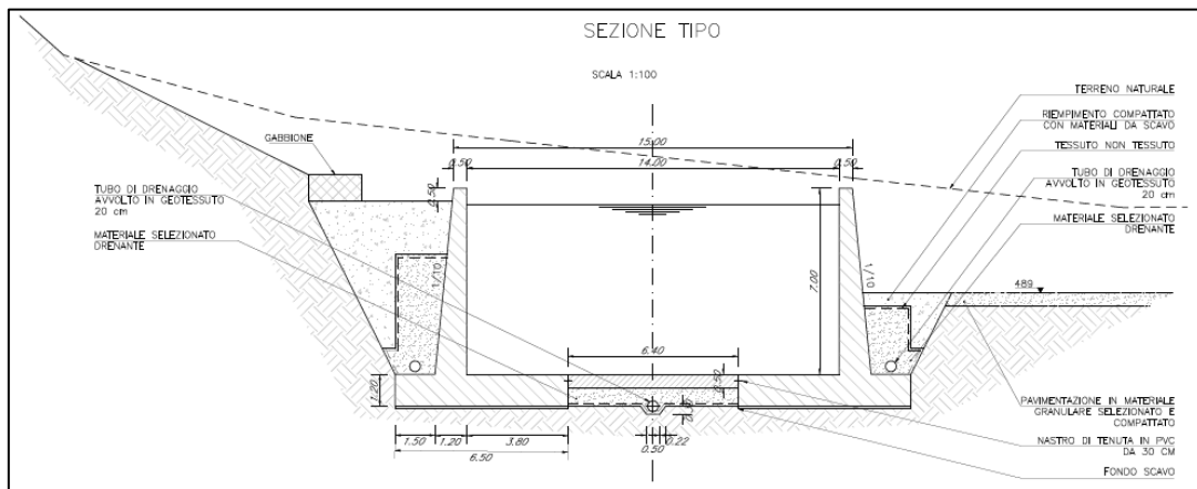
Figura 13 – Sezione Tipo della Canalizzazione del Torrente Ficocchia
