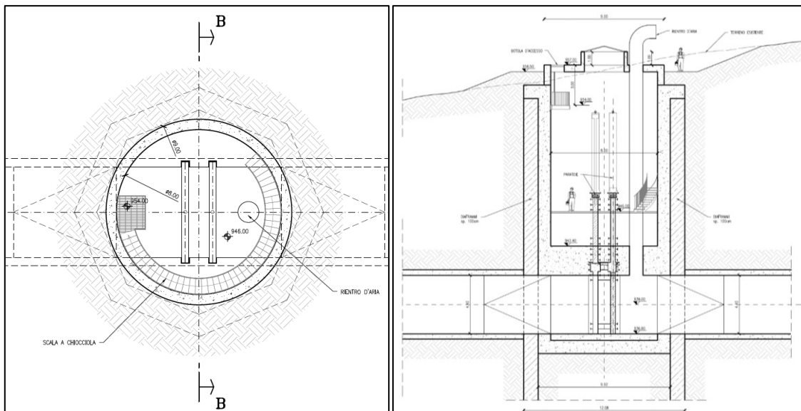
Figura 5 – Pianta e sezione del pozzo paratoie
