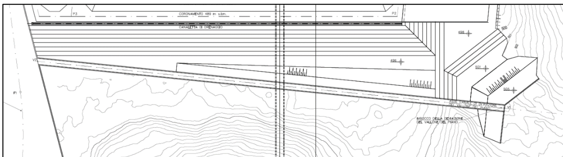
Figura 14 – Pianta della deviazione del torrente Vallone del Piano (monte a dx, valle a sx)
