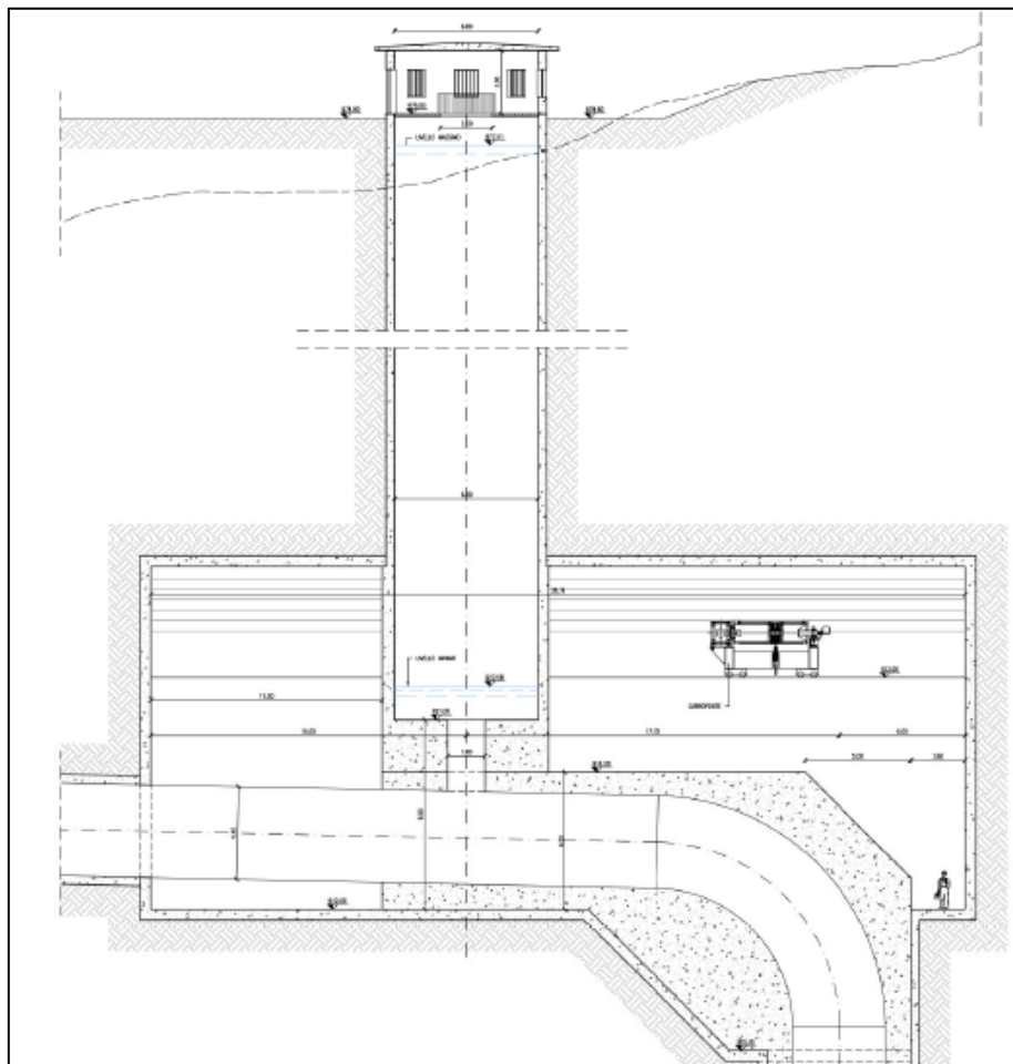
Figura 6 – Sezione del pozzo piezometrico e della caverna alla sua base
