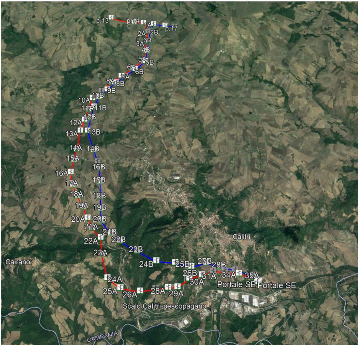
Figura 17: inquadramento dei raccordi aerei a 380 kV su ortofoto
