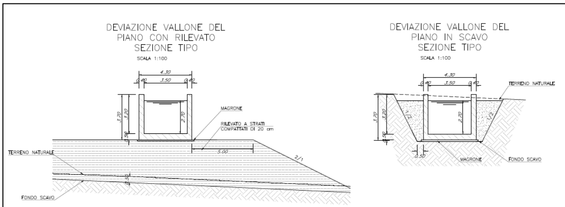
Figura 15 – Sezione tipo della canalizzazione del torrente Ficocchia
