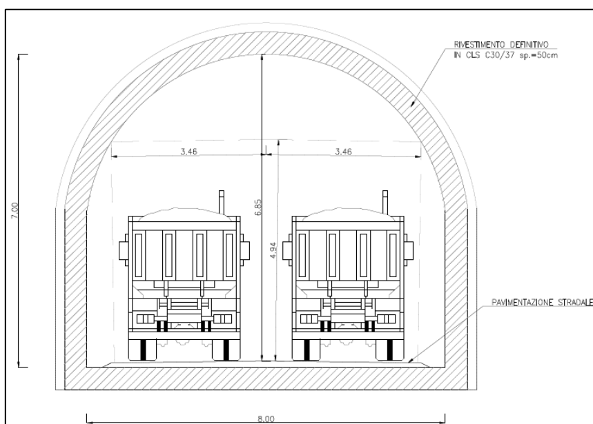
Figura 7 – Sezione tipo della galleria d'accesso alla camera alla base del pozzo piezometrico
