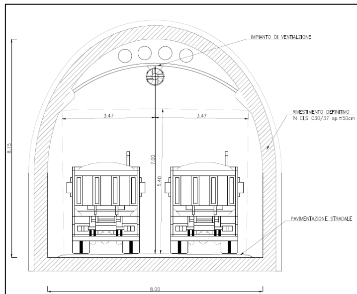
Figura 11 – Sezione tipo della galleria di accesso alla centrale
