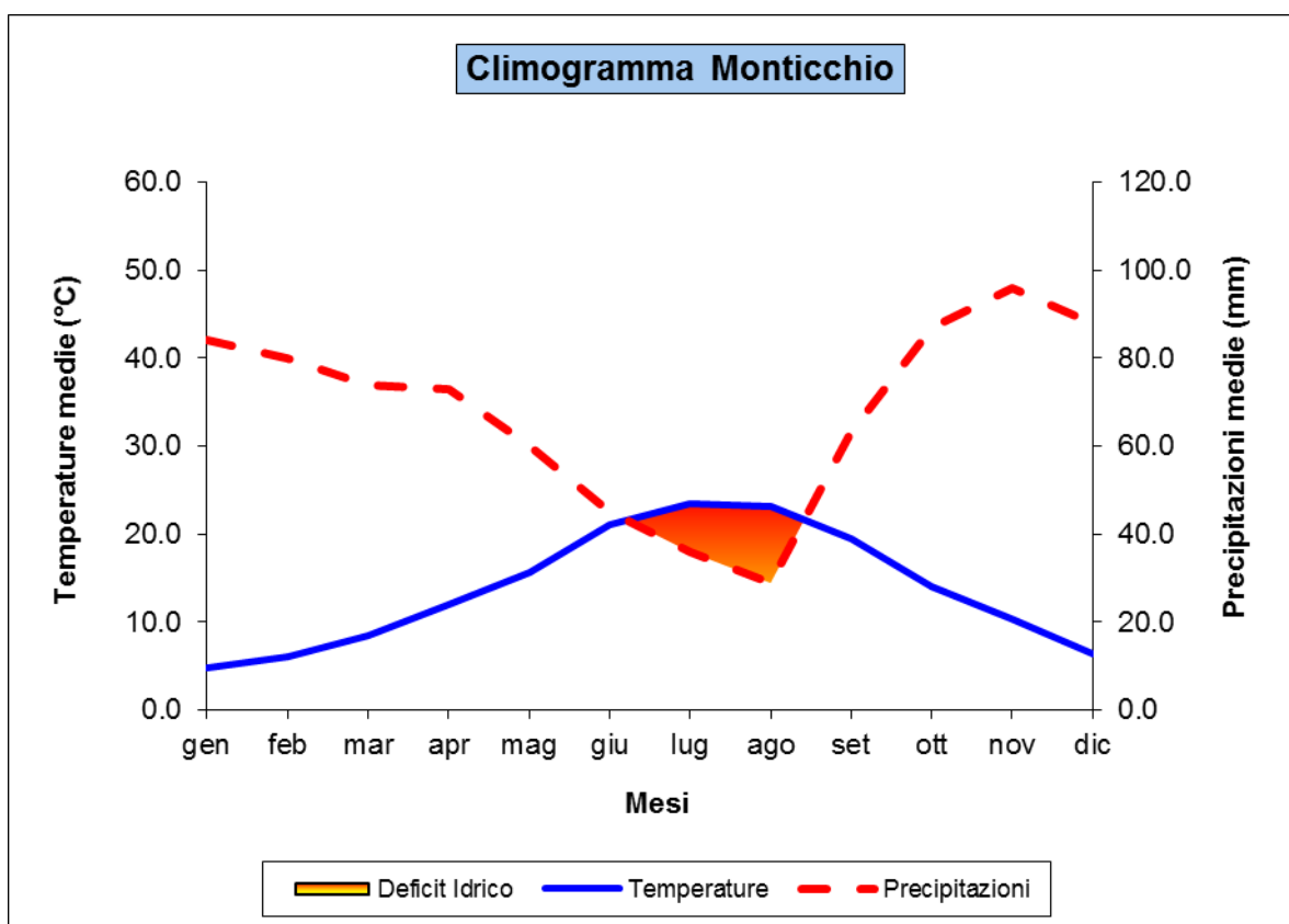
Figura 1: climogramma stazione di Monticchio
