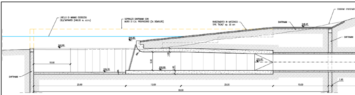
Figura 4 – Sezione Opera di Presa Saetta
