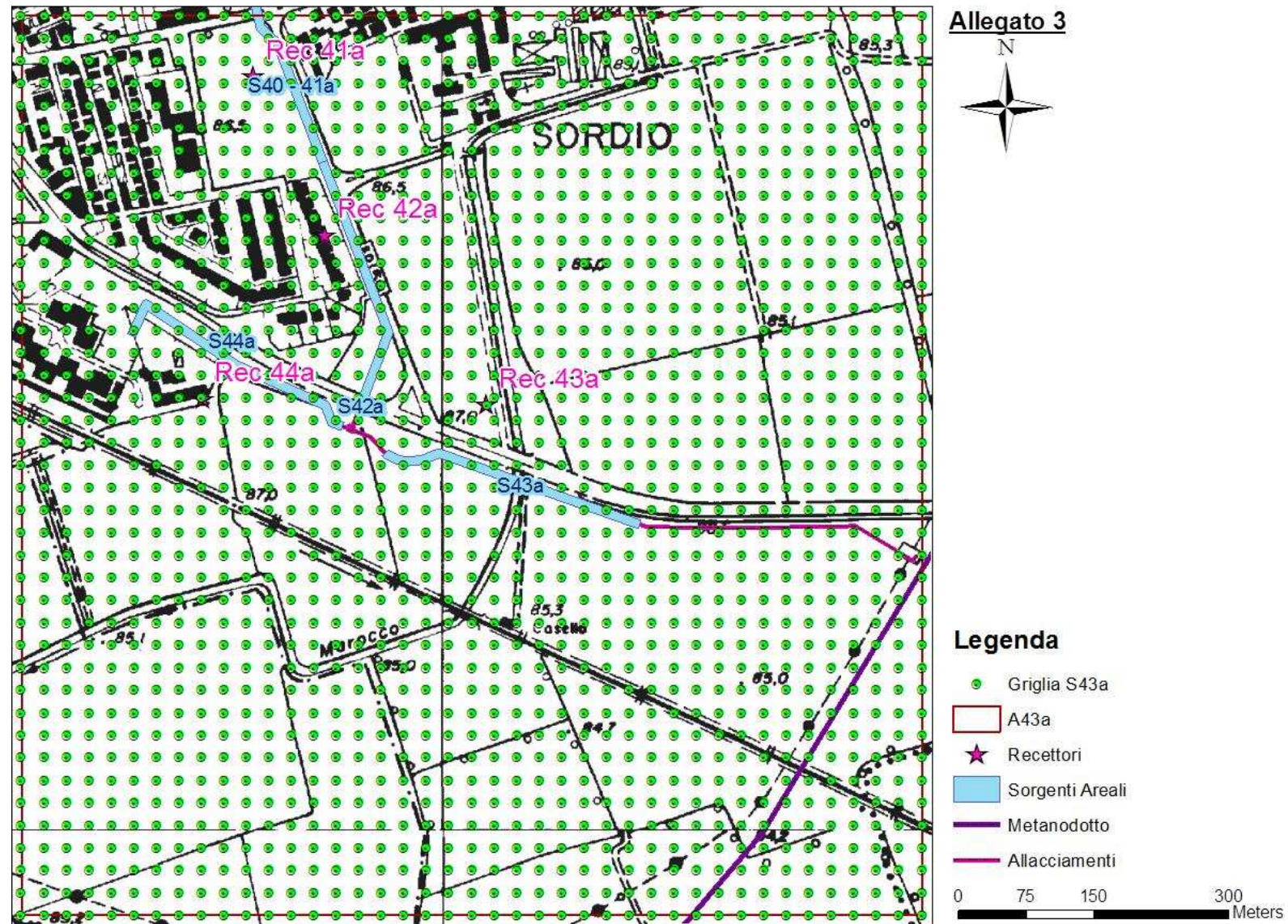
Figura 61 - Localizzazione Griglia di Calcolo Sorgente S43a.
