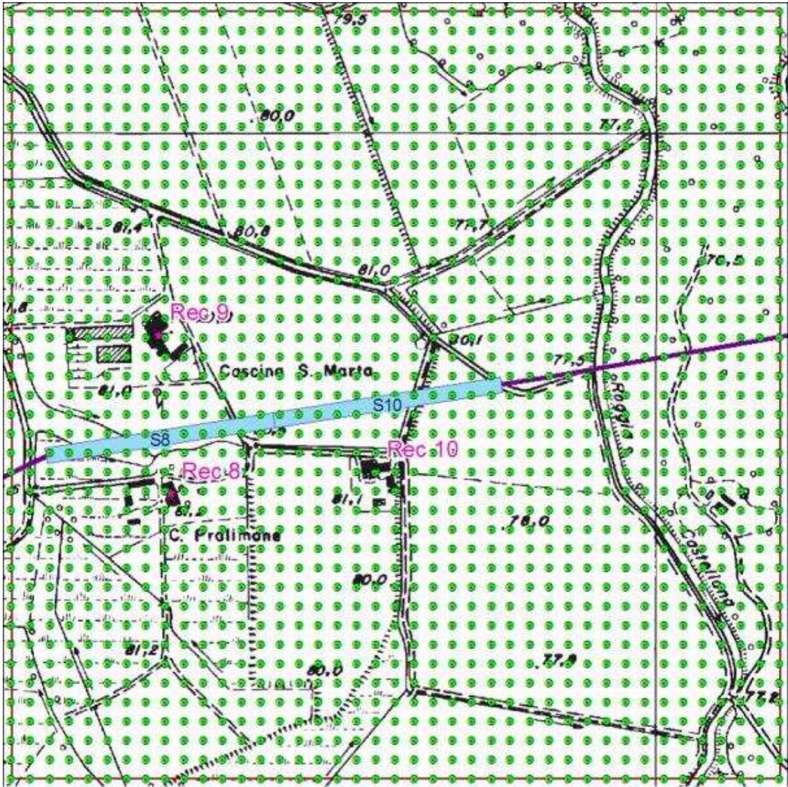
Figura 7 - Localizzazione Griglia di Calcolo Sorgente S10.
