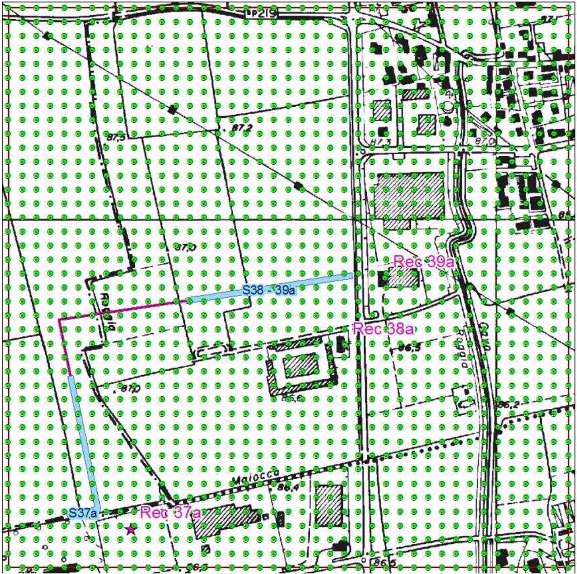
Figura 58 - Localizzazione Griglia di Calcolo Sorgente S38-39a.
