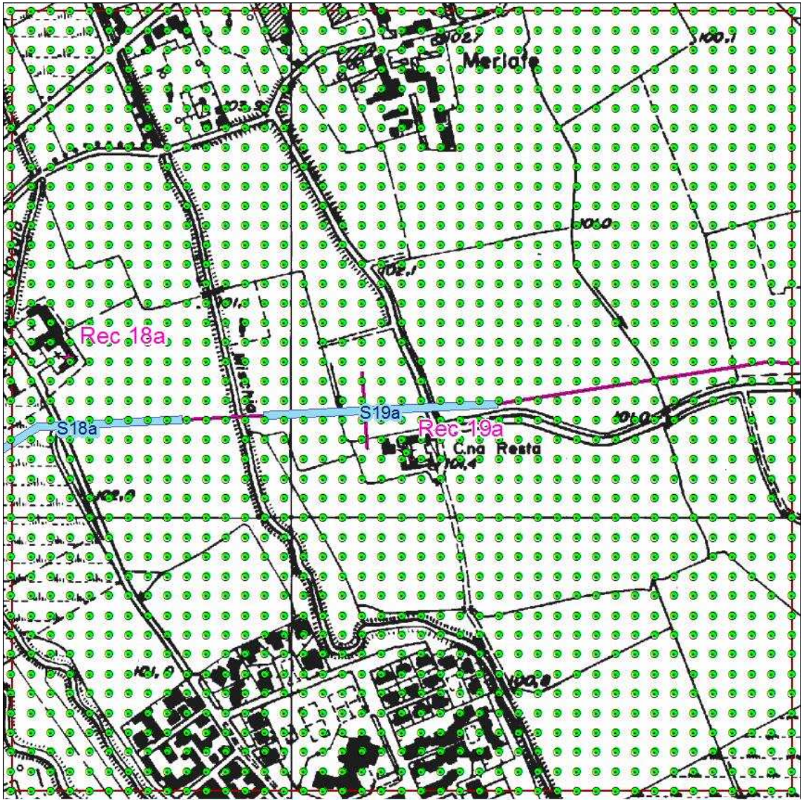
Figura 43 - Localizzazione Griglia di Calcolo Sorgente S19a.
