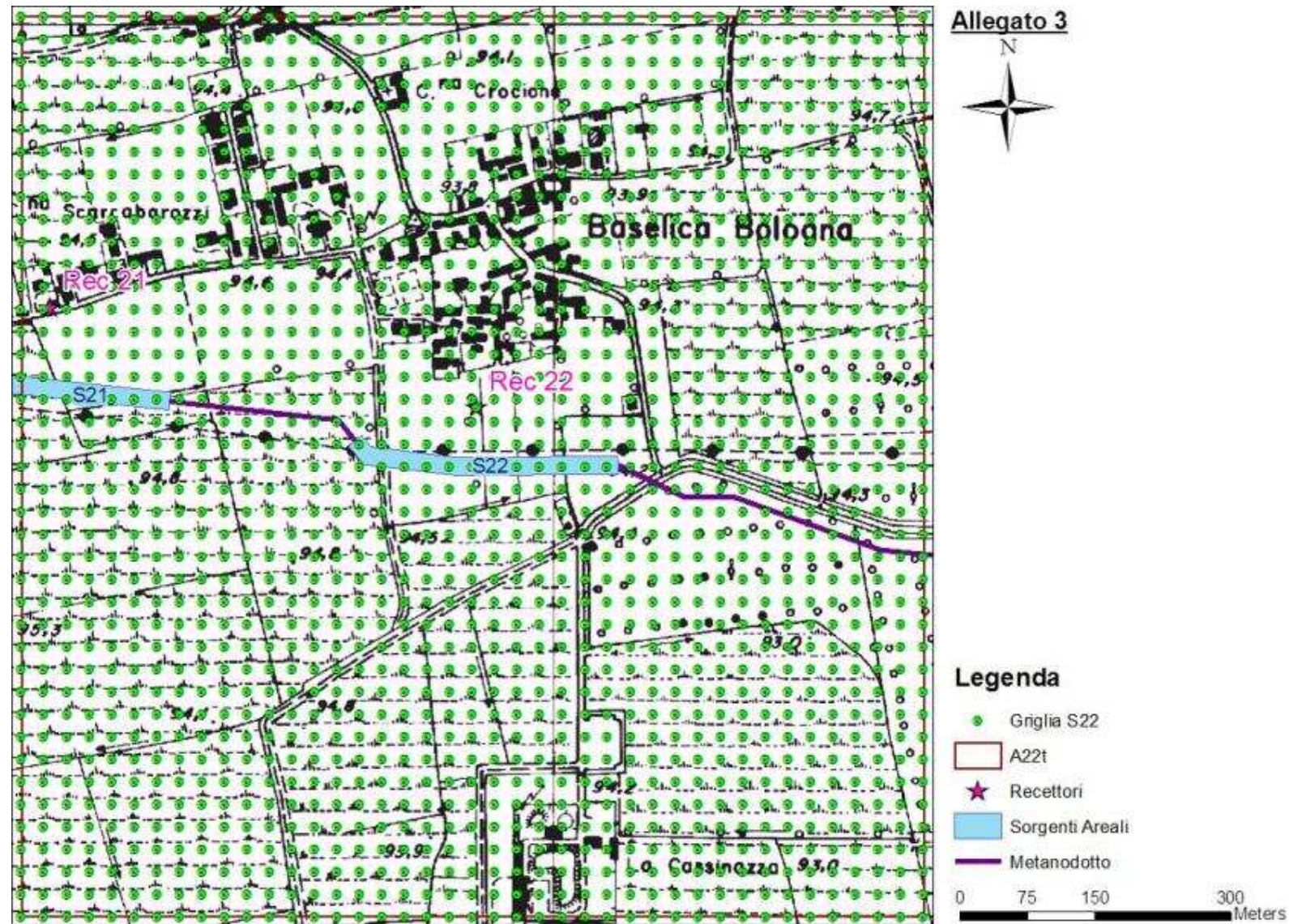
Figura 19 - Localizzazione Griglia di Calcolo Sorgente S22.
