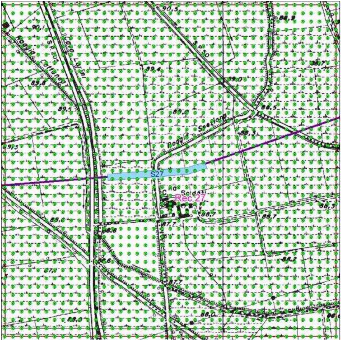
Figura 24 - Localizzazione Griglia di Calcolo Sorgente S27.
