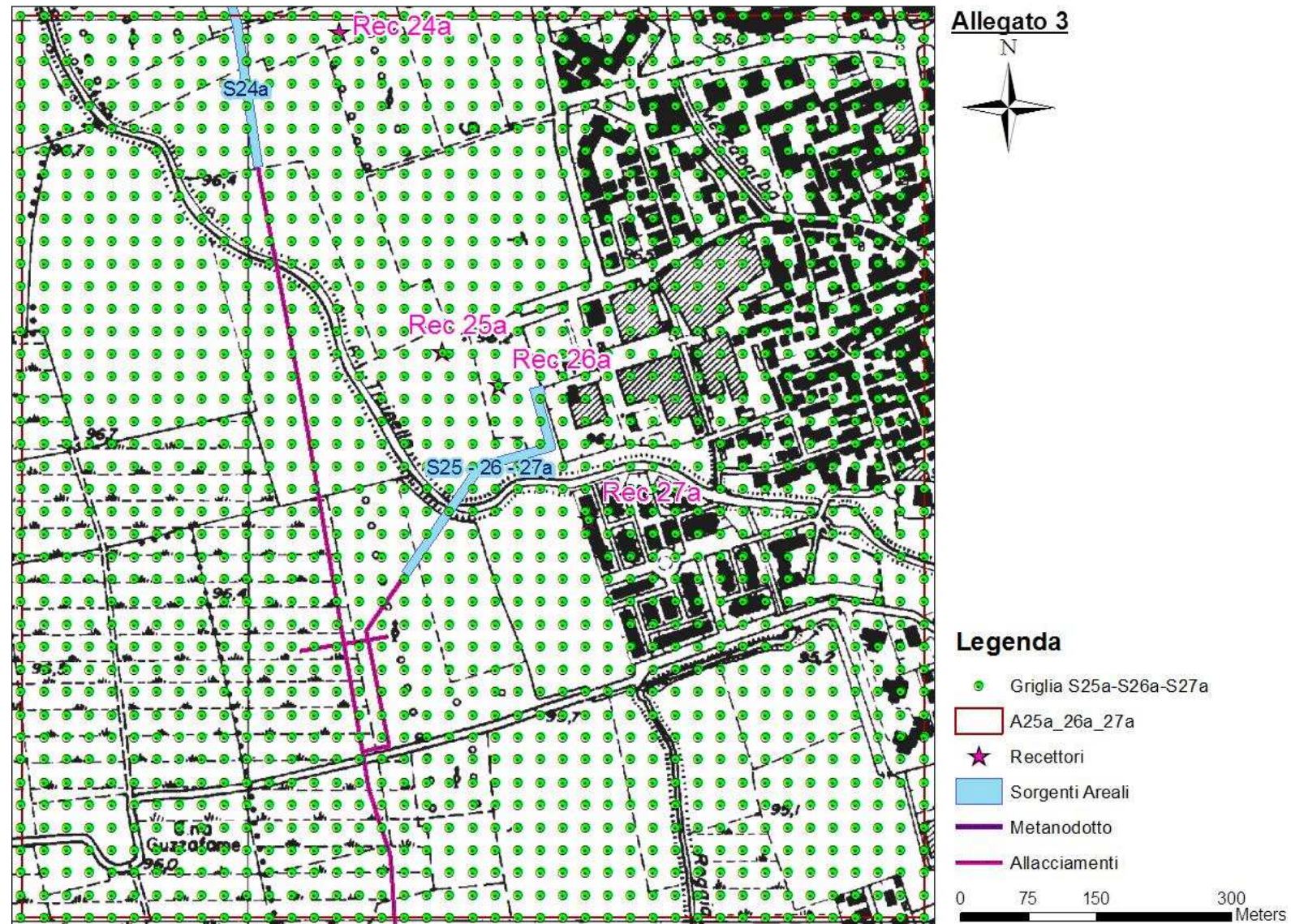
Figura 48 - Localizzazione Griglia di Calcolo Sorgente S25-26-27a.
