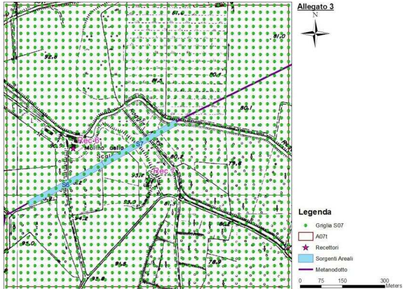
Figura 5 - Localizzazione Griglia di Calcolo Sorgente S7.
