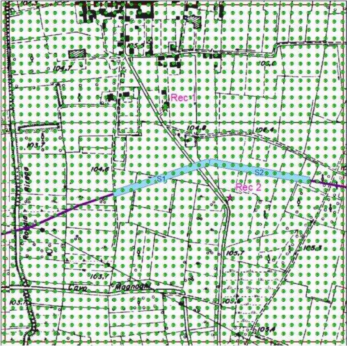
Figura 1 - Localizzazione Griglia di Calcolo Sorgente S1.
