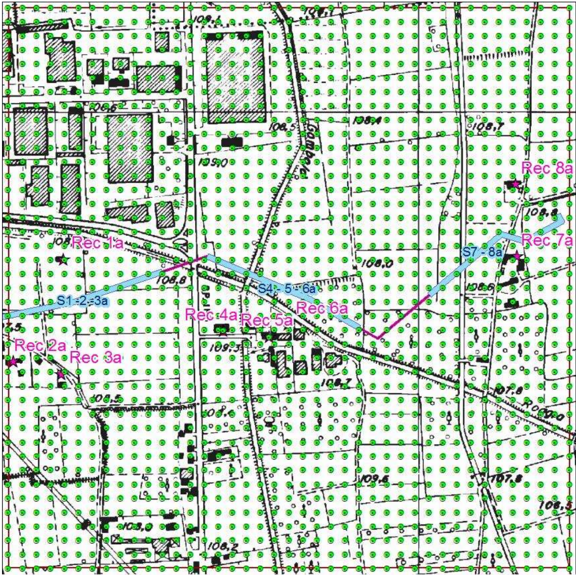
Figura 34 - Localizzazione Griglia di Calcolo Sorgente S4-5-6a.
