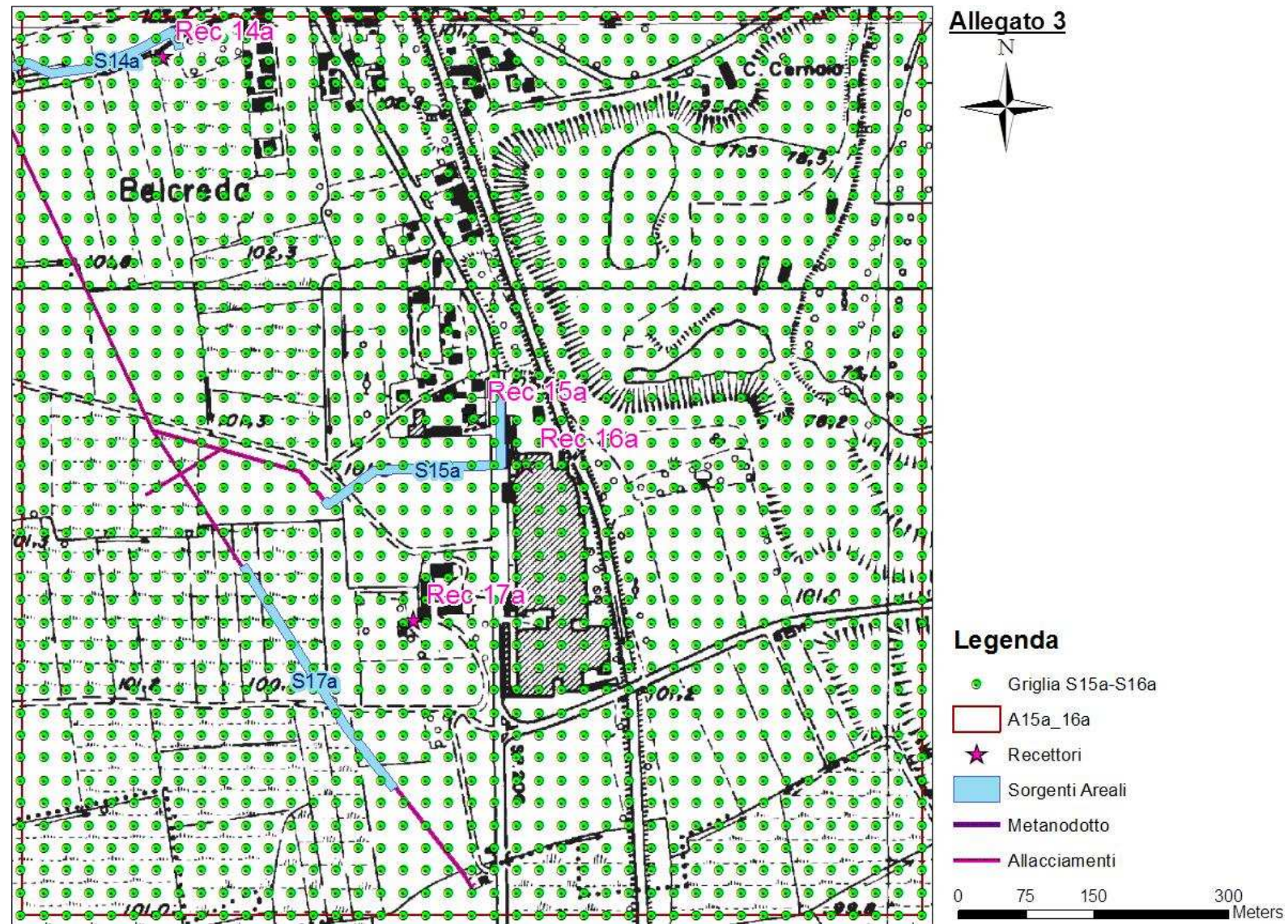
Figura 40 - Localizzazione Griglia di Calcolo Sorgente S15-16a.
