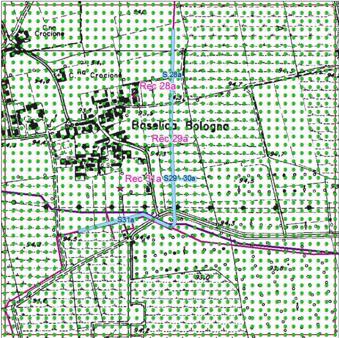
Localizzazione Griglia di Calcolo Sorgente S29-30a.
