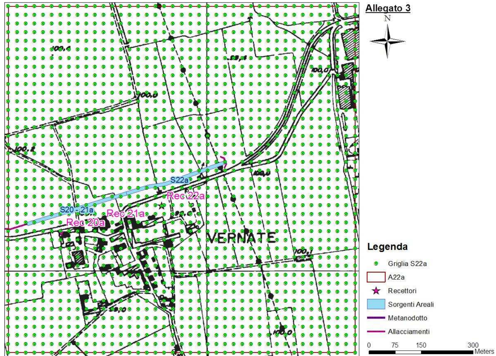
Figura 45 - Localizzazione Griglia di Calcolo Sorgente S22a.
