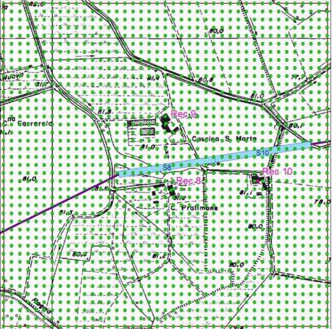
Figura 6 - Localizzazione Griglia di Calcolo Sorgente S08-09.
