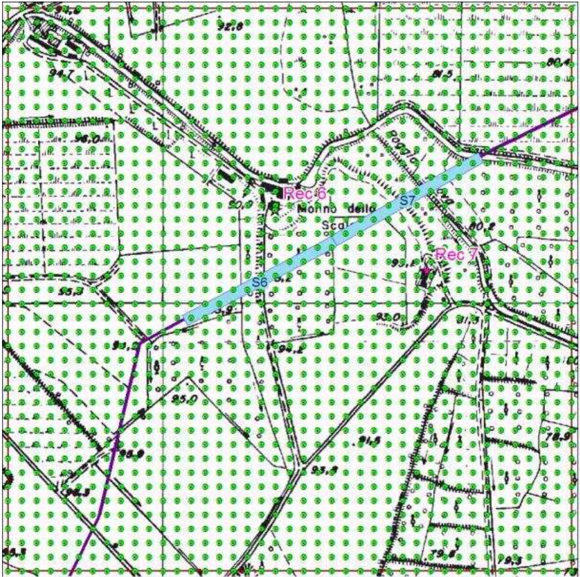
Figura 4 - Localizzazione Griglia di Calcolo Sorgente S6.
