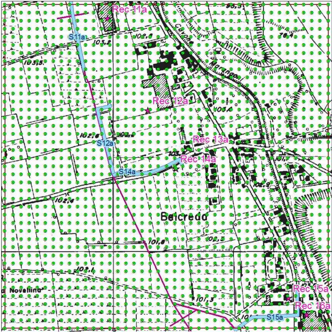
Figura 39 - Localizzazione Griglia di Calcolo Sorgente S13-14a.
