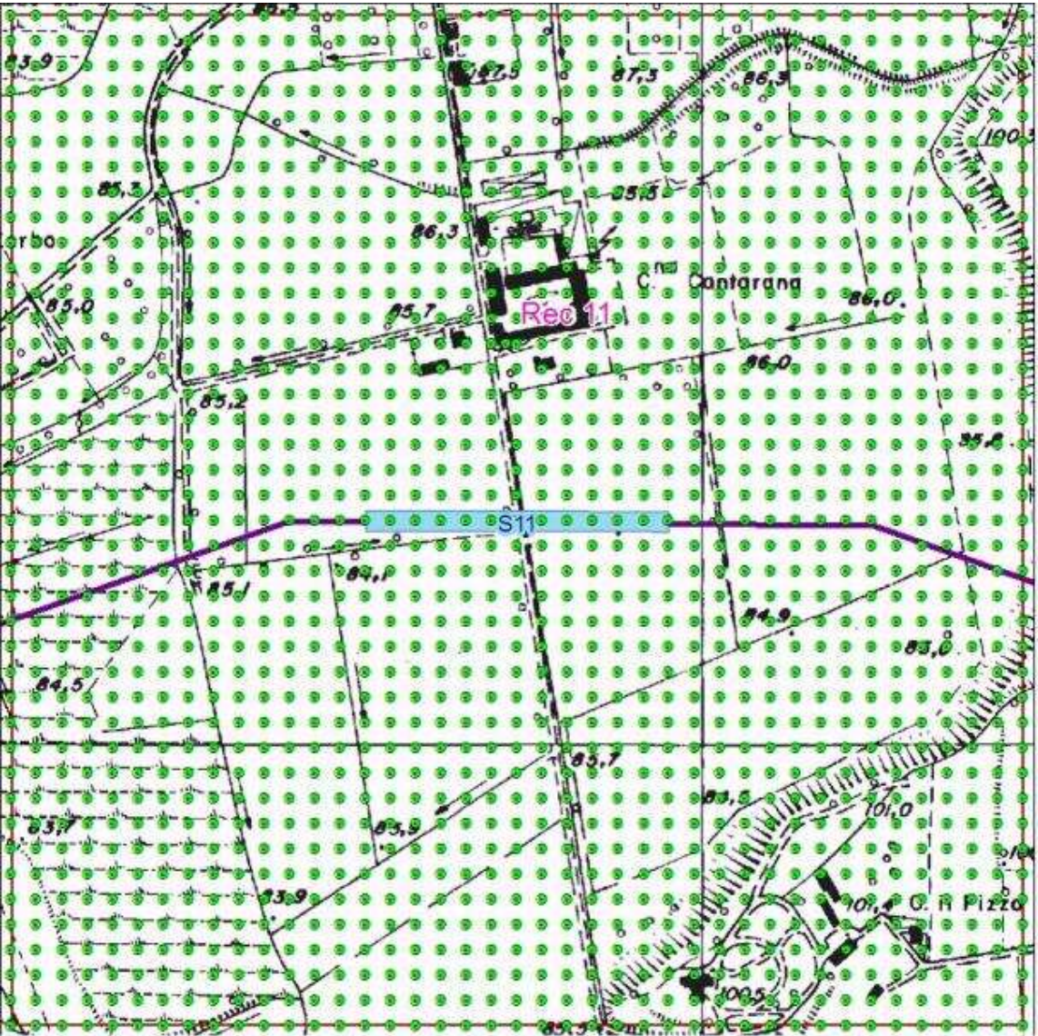
Figura 8 - Localizzazione Griglia di Calcolo Sorgente S11.
