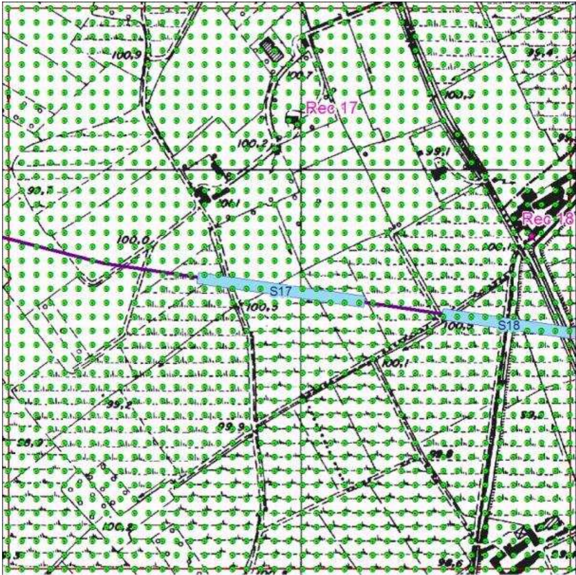
Figura 14 - Localizzazione Griglia di Calcolo Sorgente S17.
