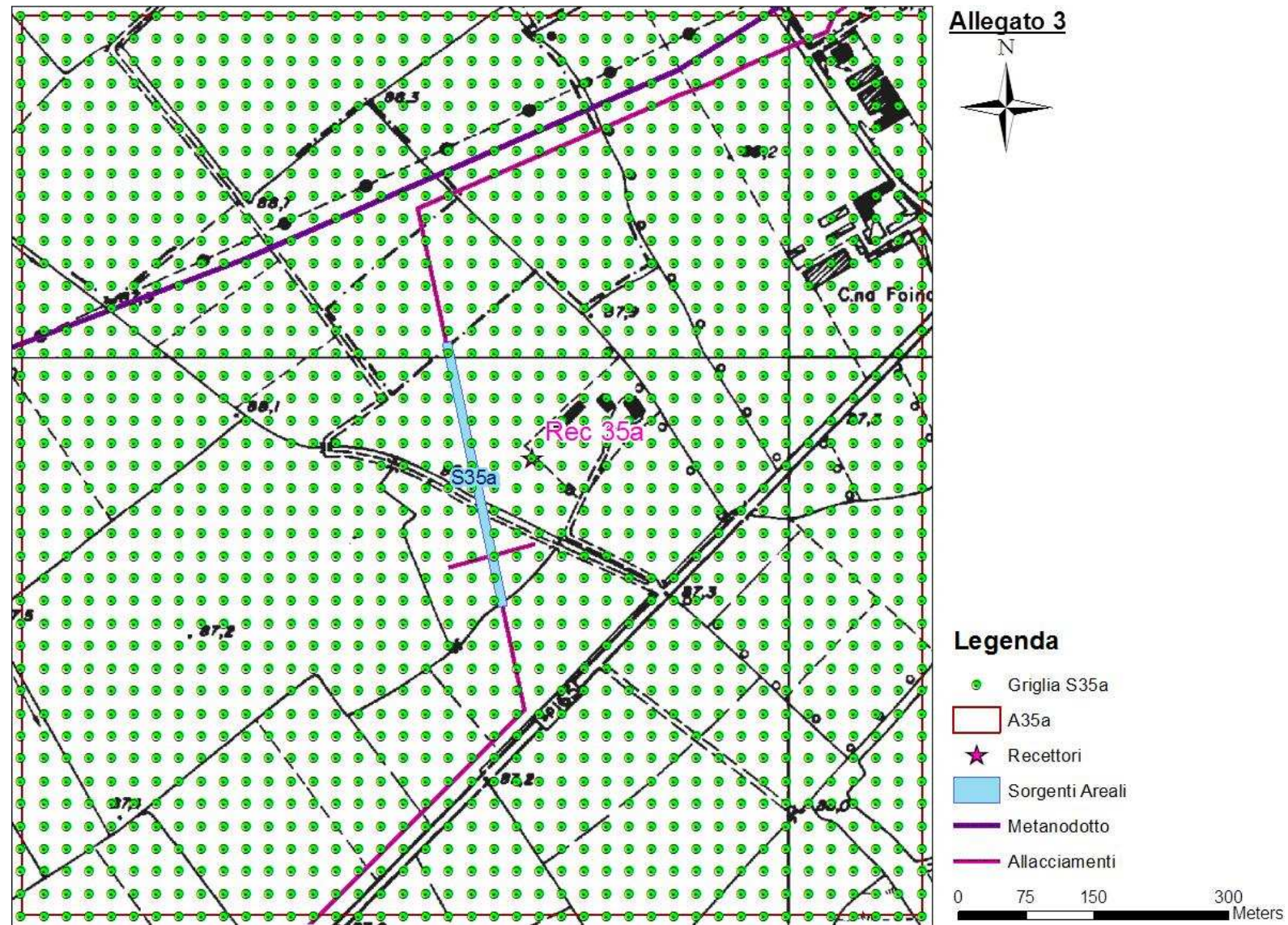
Figura 55 - Localizzazione Griglia di Calcolo Sorgente S35a.
