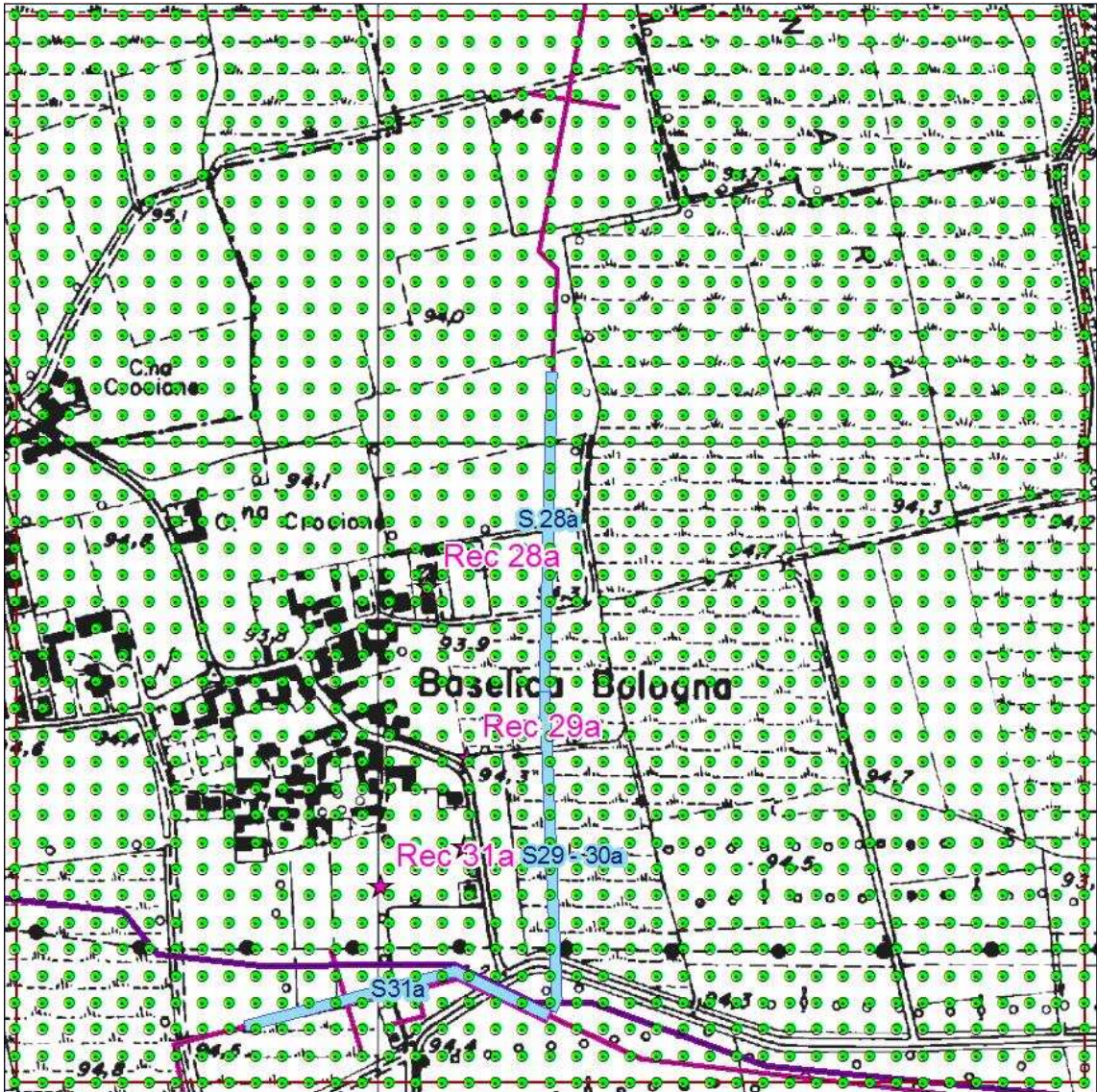
Figura 49 - Localizzazione Griglia di Calcolo Sorgente S28a.
