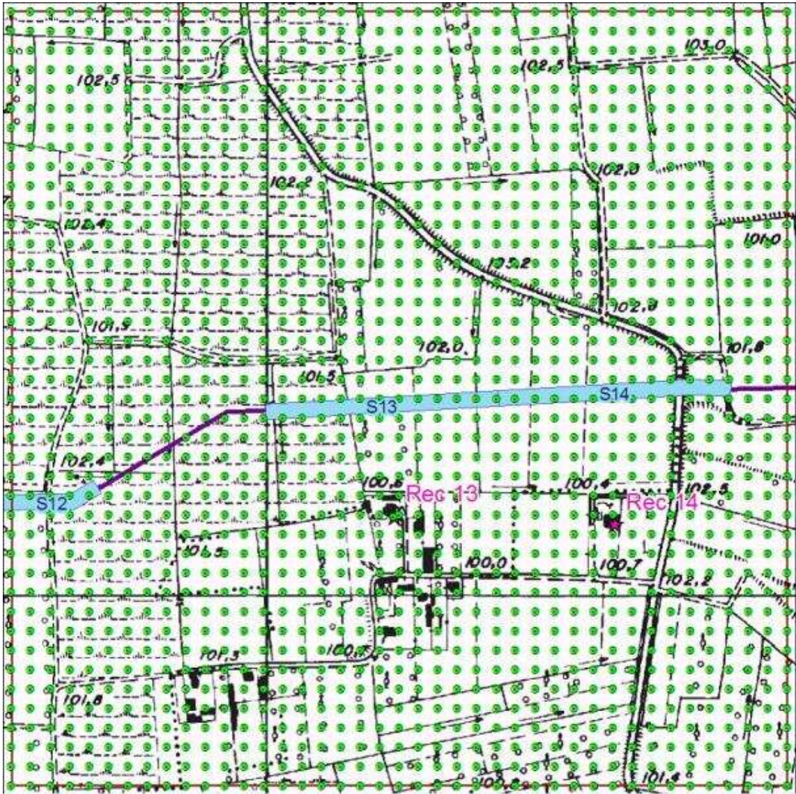
Figura 10 - Localizzazione Griglia di Calcolo Sorgente S13.
