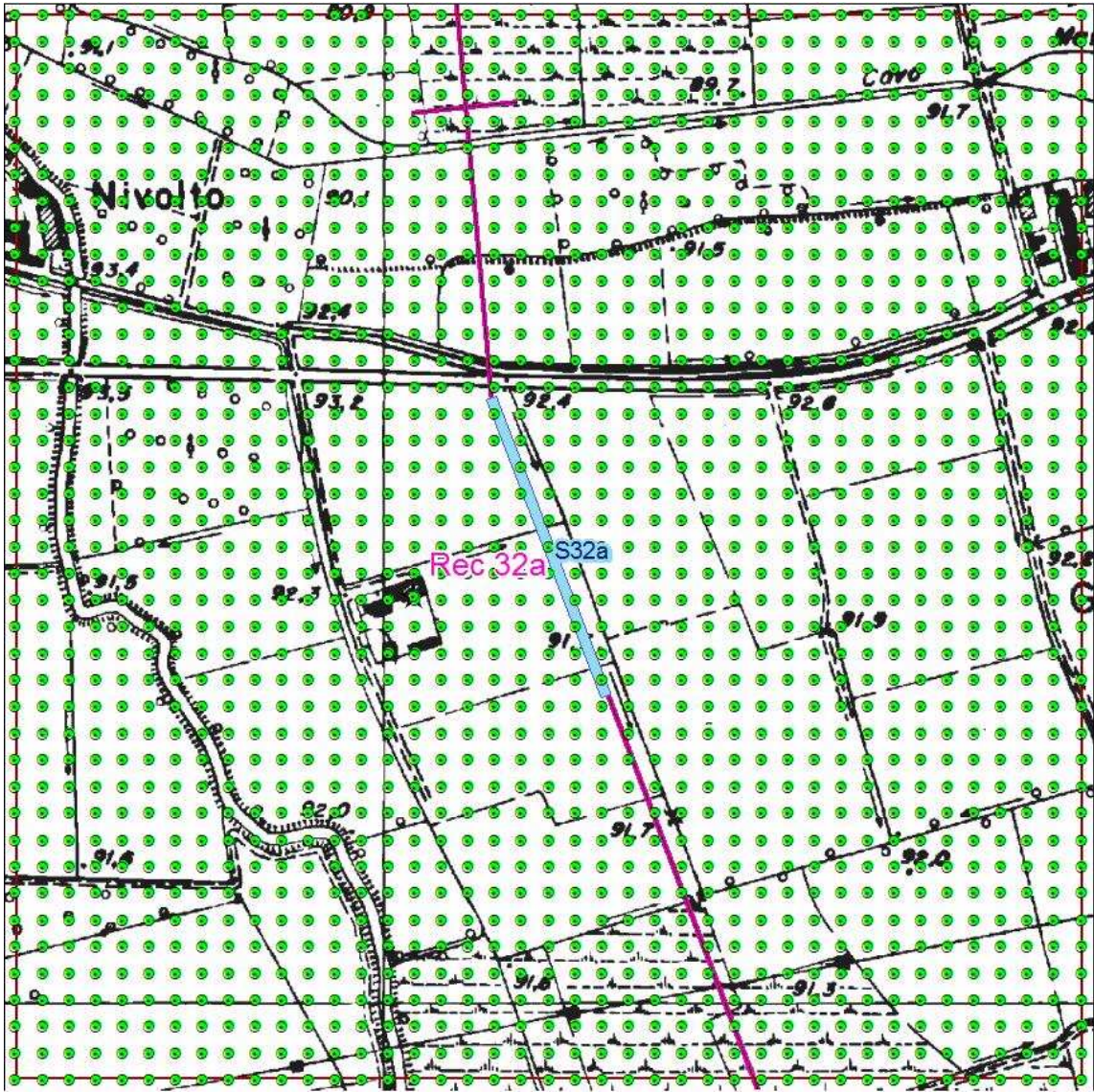
Figura 52 - Localizzazione Griglia di Calcolo Sorgente S32a.
