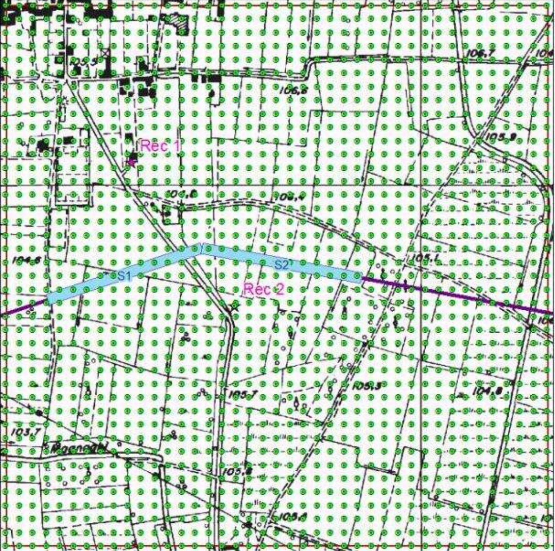
Figura 2 - Localizzazione Griglia di Calcolo Sorgente S2.
