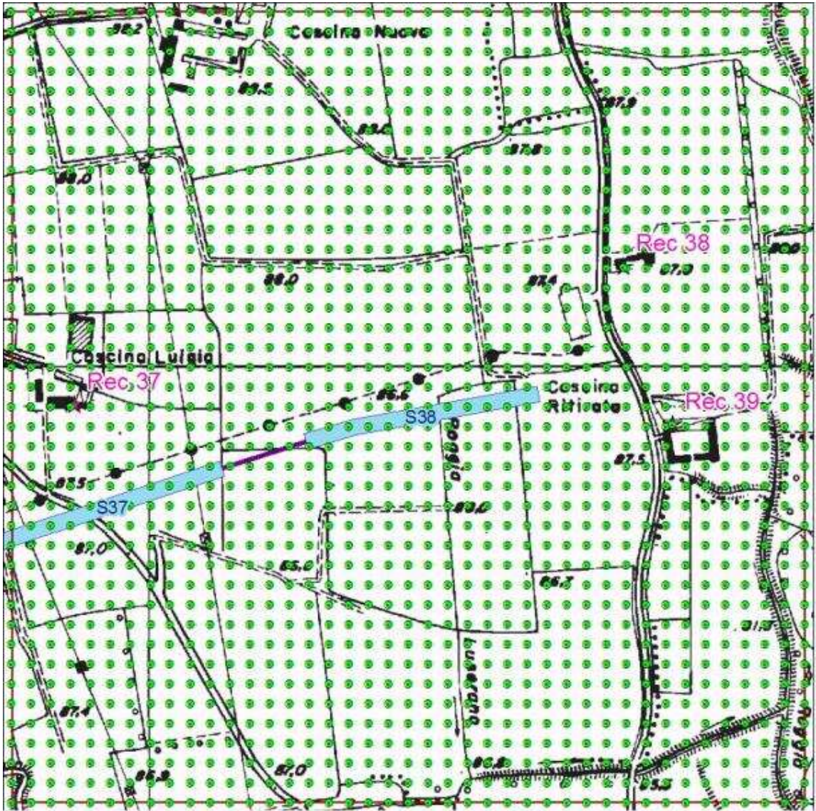
Figura 32 - Localizzazione Griglia di Calcolo Sorgente S38-39.
