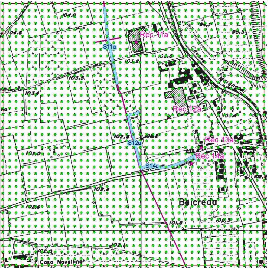
Figura 38 - Localizzazione Griglia di Calcolo Sorgente S12a.
