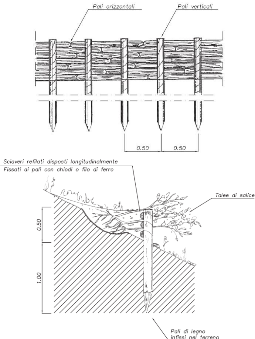
Fig. 10.2 – Ripristino scarpate con palizzate in legname
