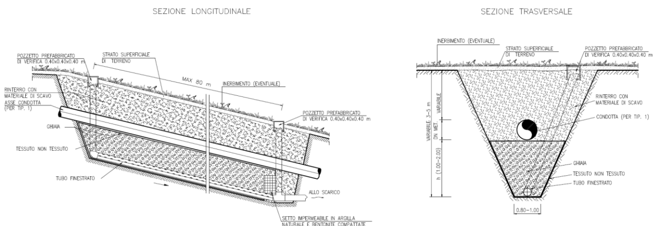
Fig. 10.10: Trincea drenante.
