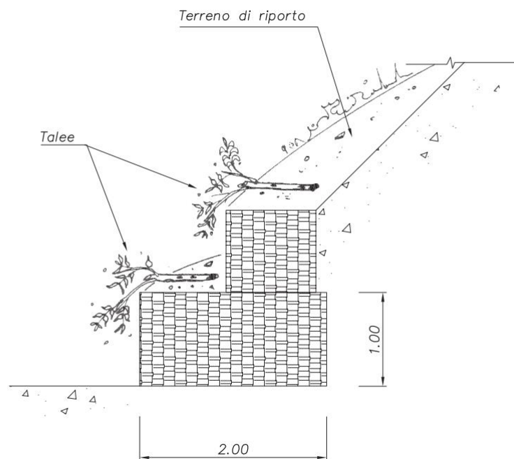
Fig. 10.6: Ricostruzione spondale con gabbioni interrati
