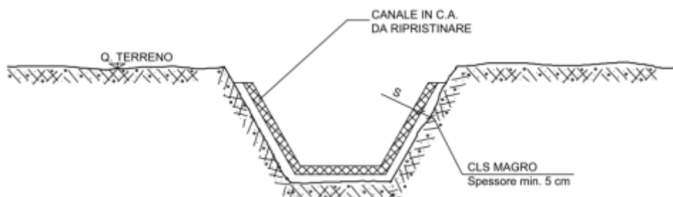
Fig. 10.9: Ripristino canale in c.a.
