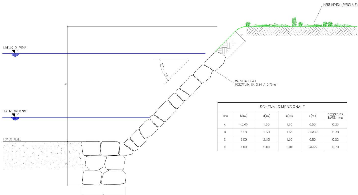
Fig. 10.8: Ricostruzione spondale con rivestimento in massi.
