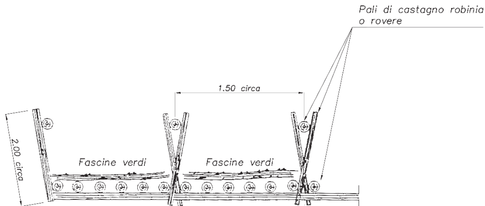
PIANTA DELLA PALIZZATA
