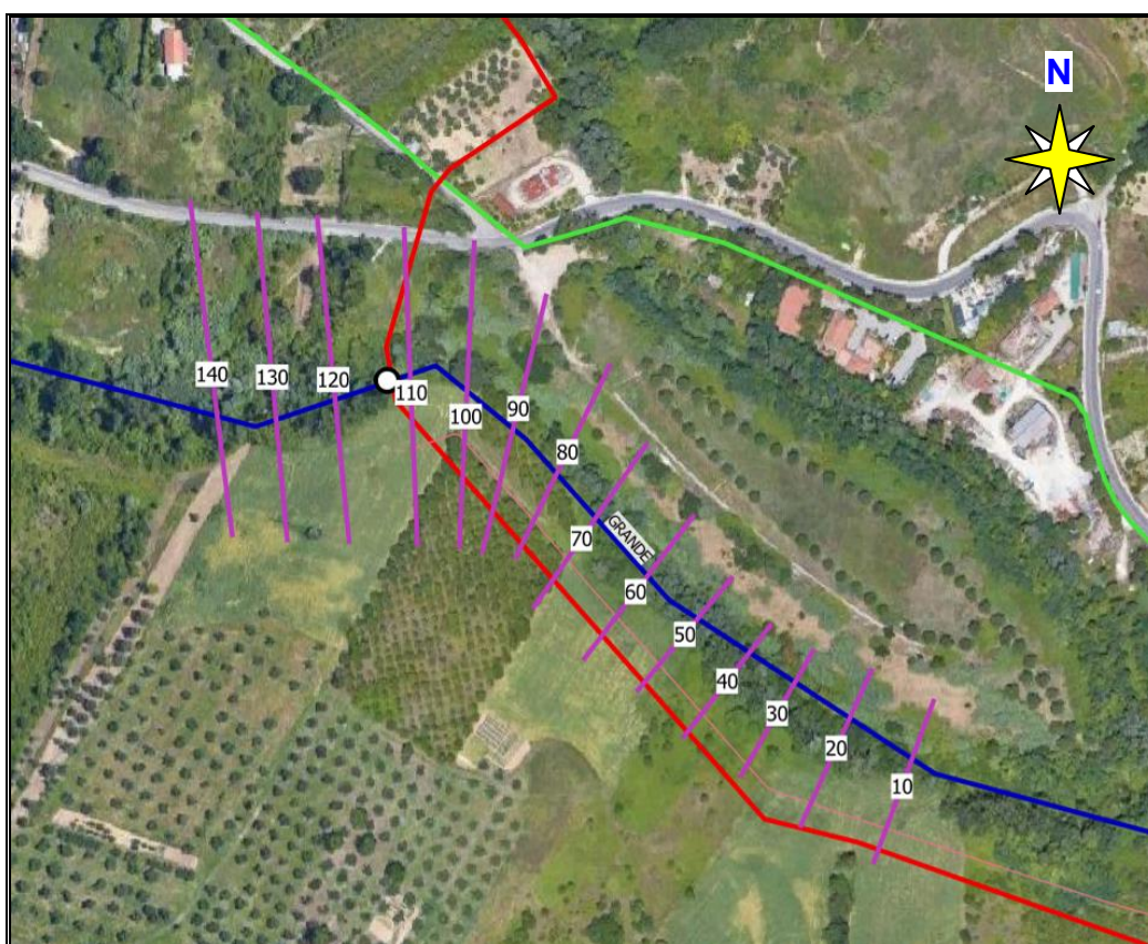
Fig.5.2/A: Foto aerea, con tronco d'alveo analizzato e sezioni di input
