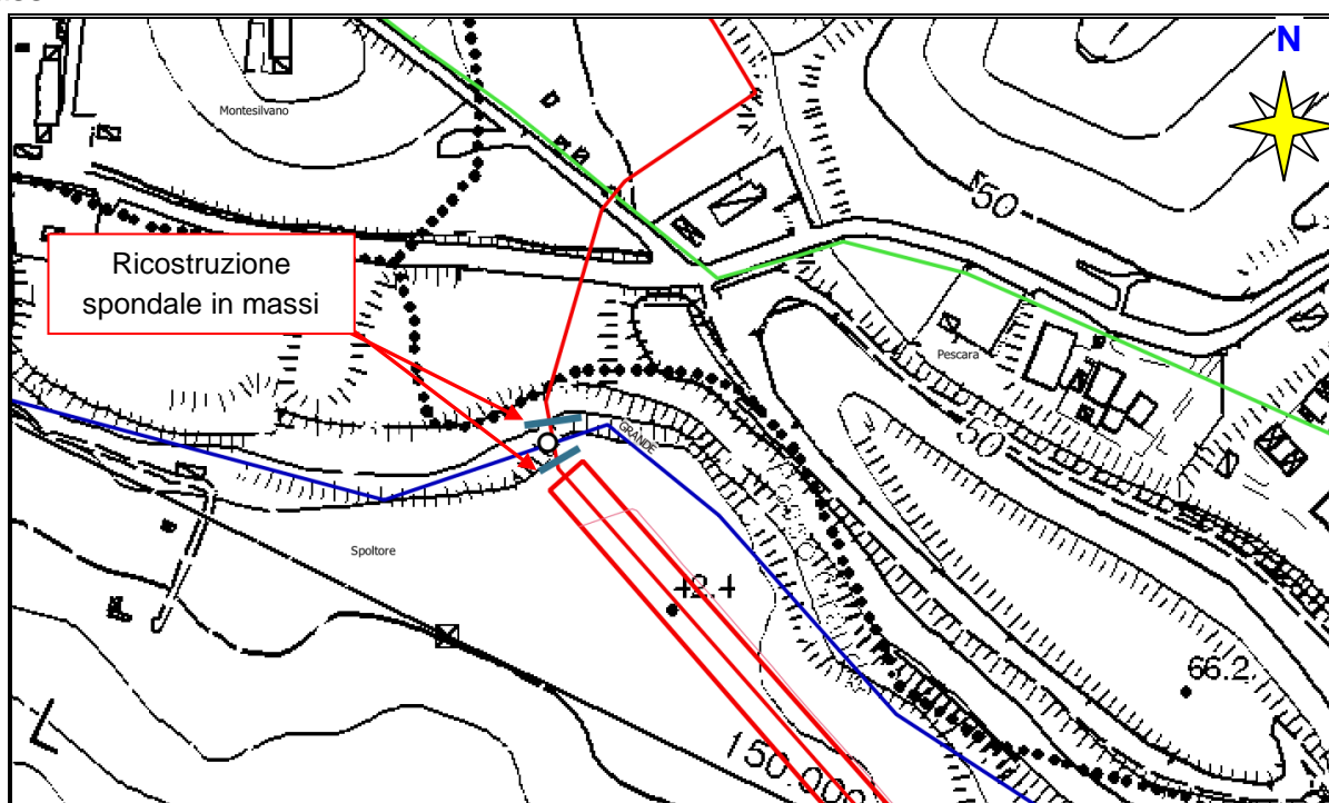
7.3/A-Stralcio C.T.R. al 10.000 con indicazione delle difese spondali di progetto.
