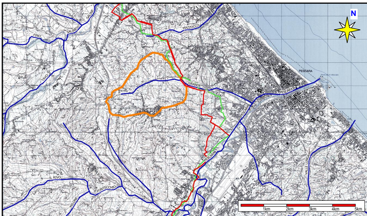
Fig.4.3/A: Bacino Imbrifero sotteso dalla sezione di studio
