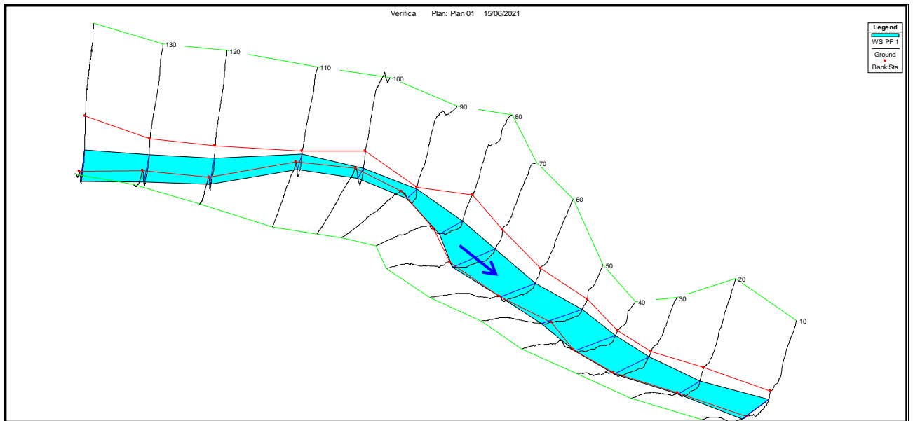
Fig.5.3/A: Schermata di Output del programma – visione prospettica (RS140: monte-RS10: valle)
