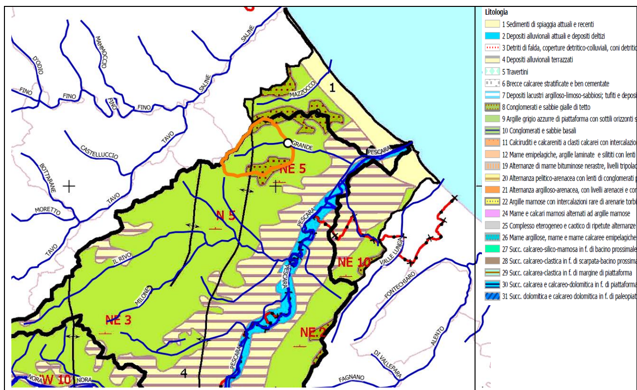
Fig.4.4/A: Bacino sulla Carta Litologica
