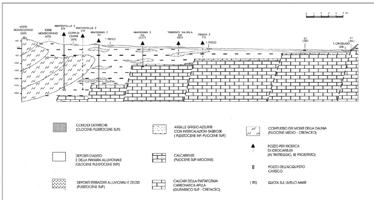
Figura 83 Sezione geologica schematica dei rapporti stratigrafici.
