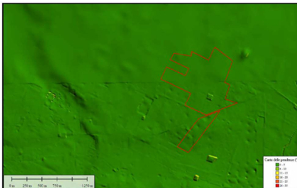
Figura 84 Carte delle pendenze dell'area
