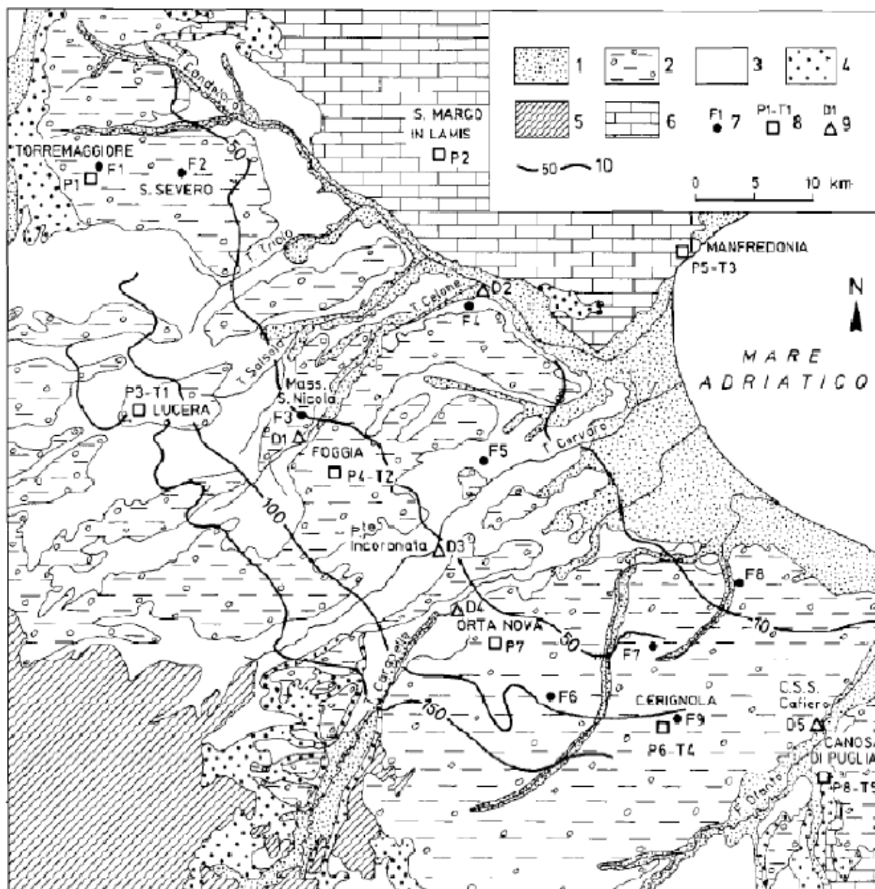
Figura 88 Carta geologica schematica del Tavoliere con indicazione delle piezometriche
