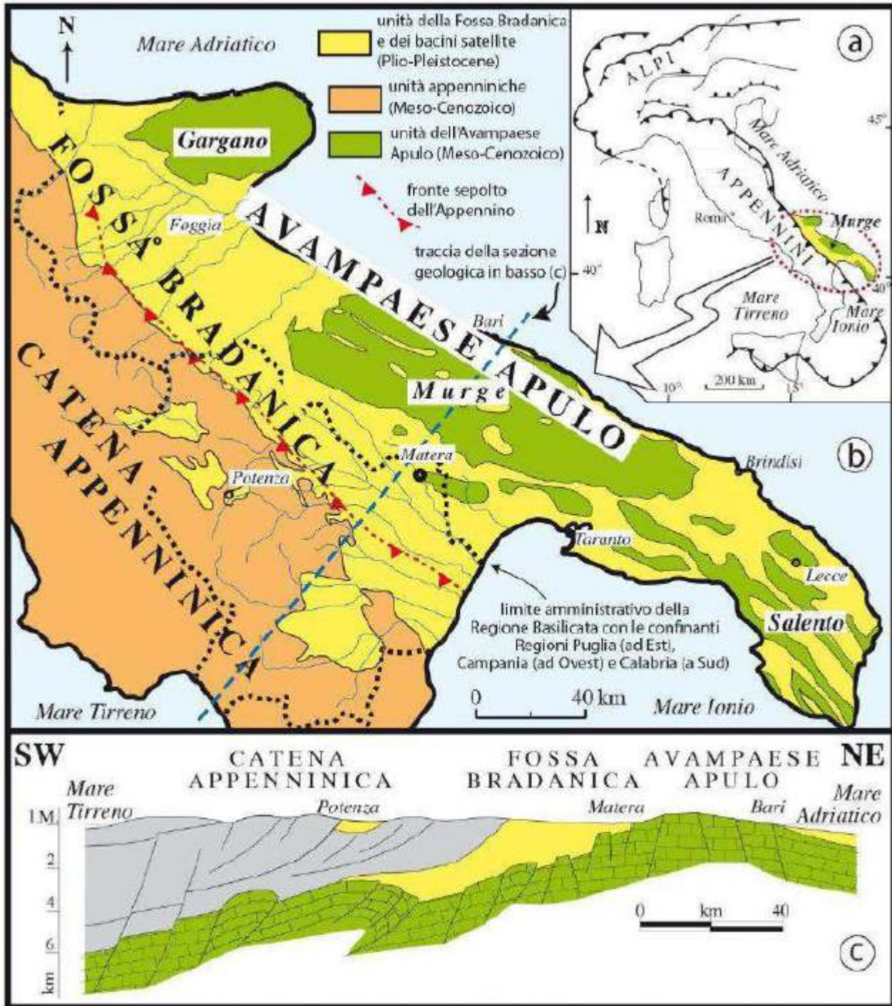
Figura 81 Schema geologico schematico della Fossa Bradanica e delle aree limitrofe (da Cotecchia V., 2014)
