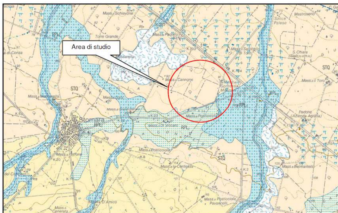
Figura 85 Stralcio carta geologica (fonte ISPRA)
