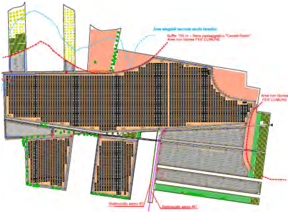
Layout dell'impianto FV
