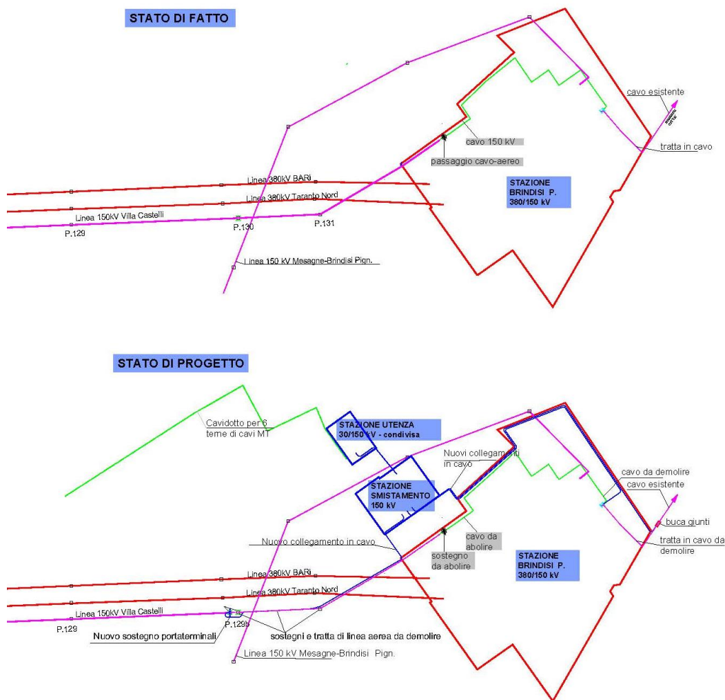
Figura 53: Stato di fatto dell'area interessata dall'iniziativa e stato di progetto dell'iniziativa in valutazione
