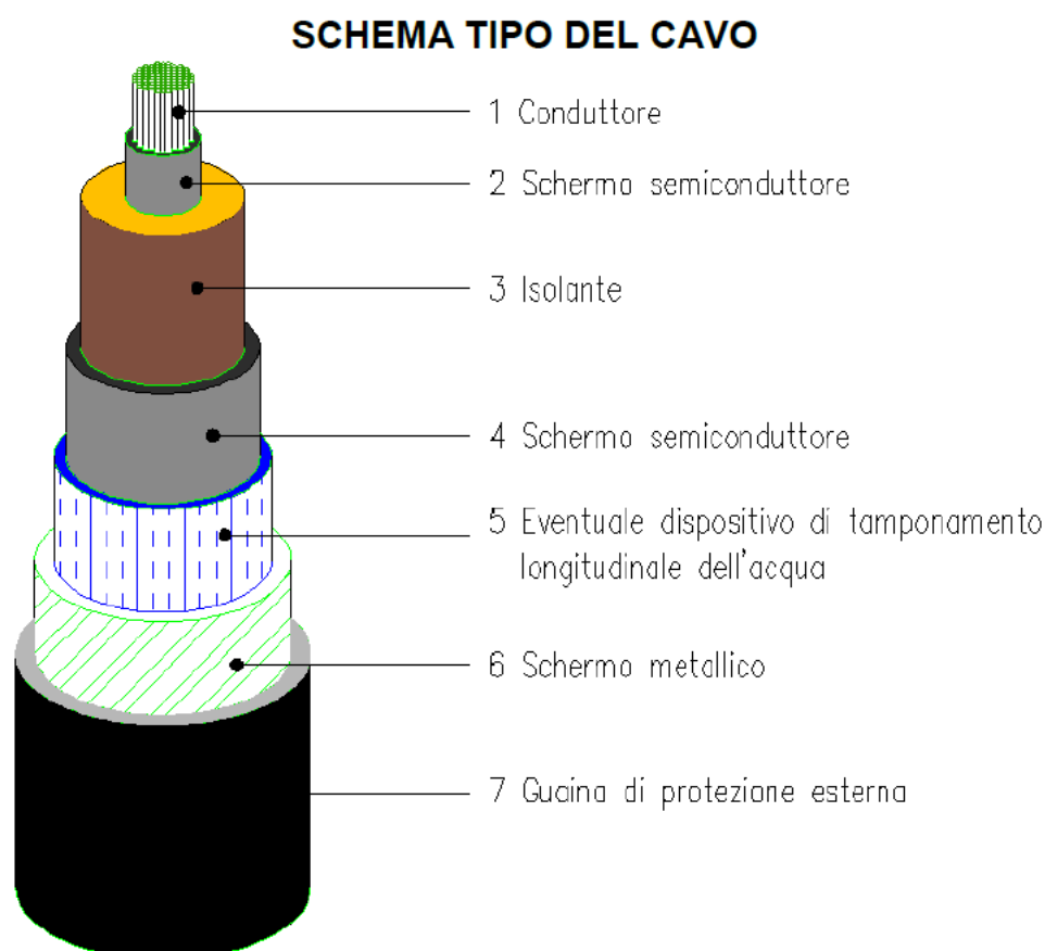
Figura 54: Schema tipo del cavo a 150 kV
