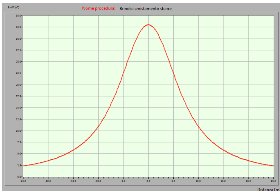
Figura 71: Profilo laterale induzione magnetica (B) sbarre 150 kV
