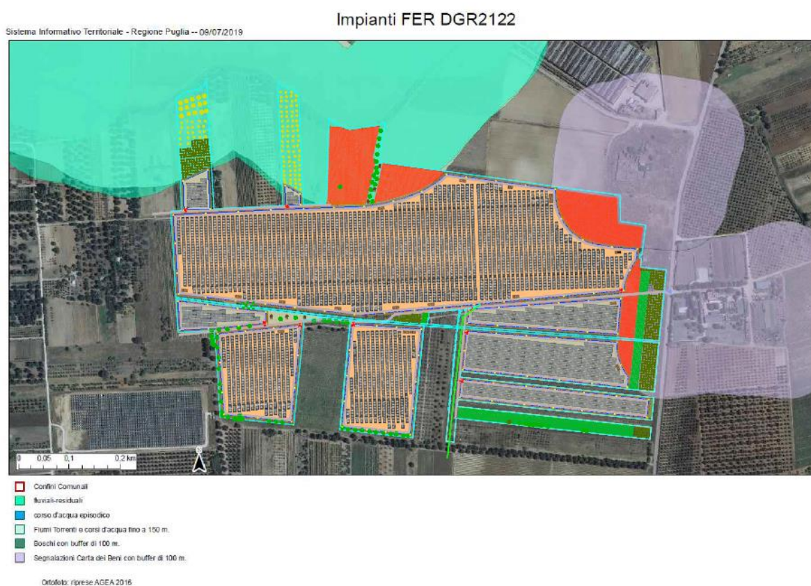
Figura 27: Stralcio Aree non idonee FER da WebGIS Puglia
