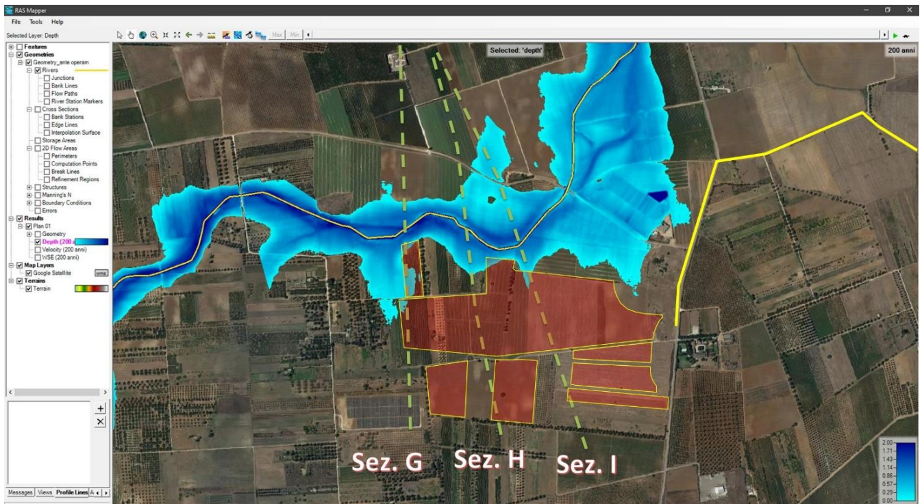
Figura 7: Risultati dello studio di compatibilità idrologica ed idraulica effettuato per tutti i reticoli presenti nell'intorno dell'area di impianto.
