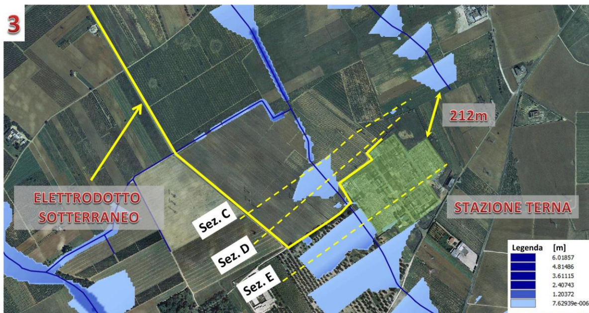
Figura 13: Risultati dello studio di compatibilità idrologica ed idraulica effettuato per tutti i reticoli presenti lungo il percorso dell'elettrodotta di connessione (punto 3).
