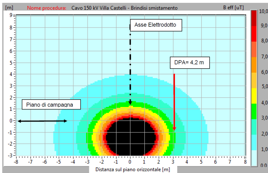
Figura 65: Mappa verticale induzione magnetica (B) sezione tipo con indicazione della DPA - V=150\text{ kV} I = 1045\text{ A}
