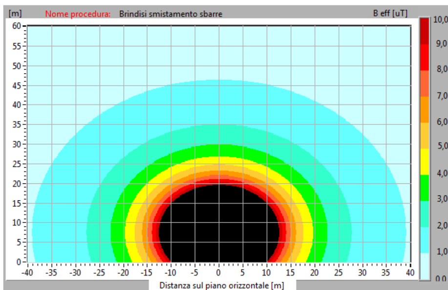
Figura 72: Mappa verticale induzione magnetica (B) sbarre 150 kV.
