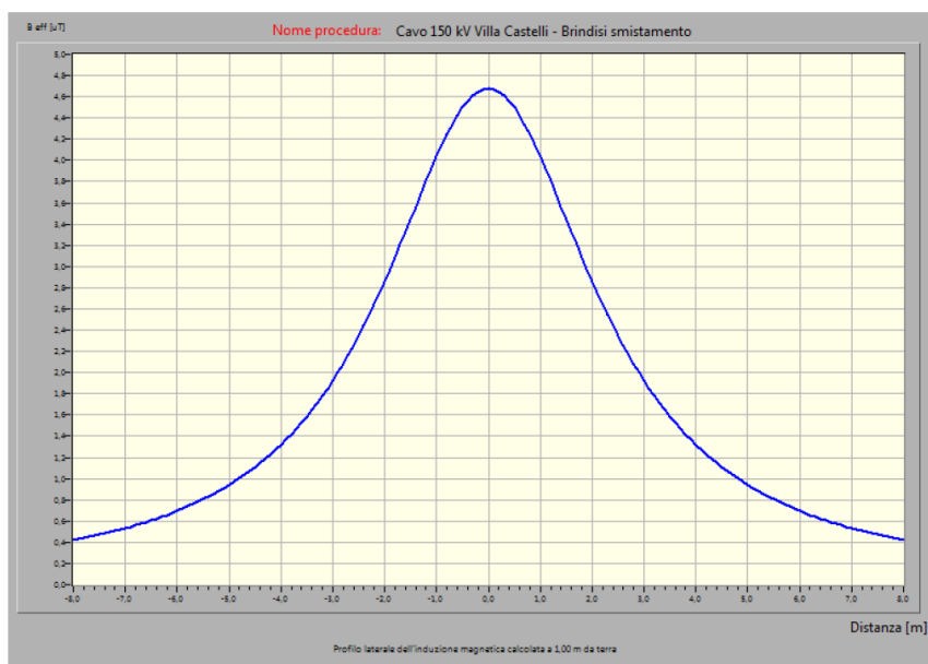
Figura 64: Profilo laterale induzione magnetica (B) sezione tipo con indicazione della DPA - V=150\text{ kV} I = 1045\text{ A}
