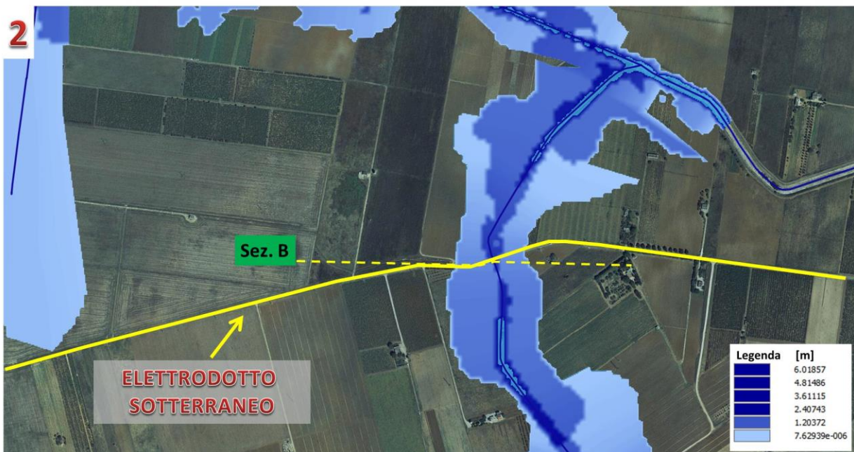
Figura 12: Risultati dello studio di compatibilità idrologica ed idraulica effettuato per tutti i reticoli presenti lungo il percorso dell'elettrodotto di connessione (punto 2).
