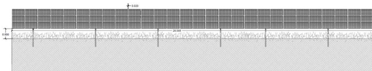
Figura 32: Vista frontale della struttura di supporto dei moduli
