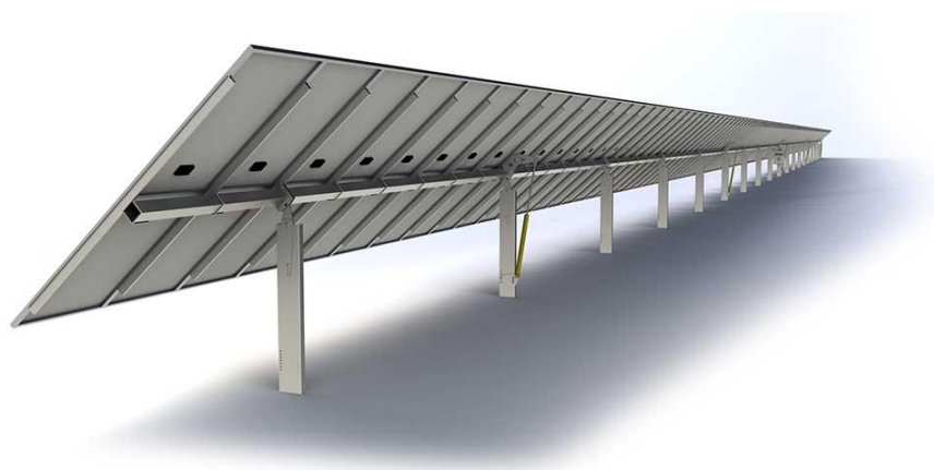
Figura 29: Prospetto frontale della struttura di sostegno dei moduli su tracker
