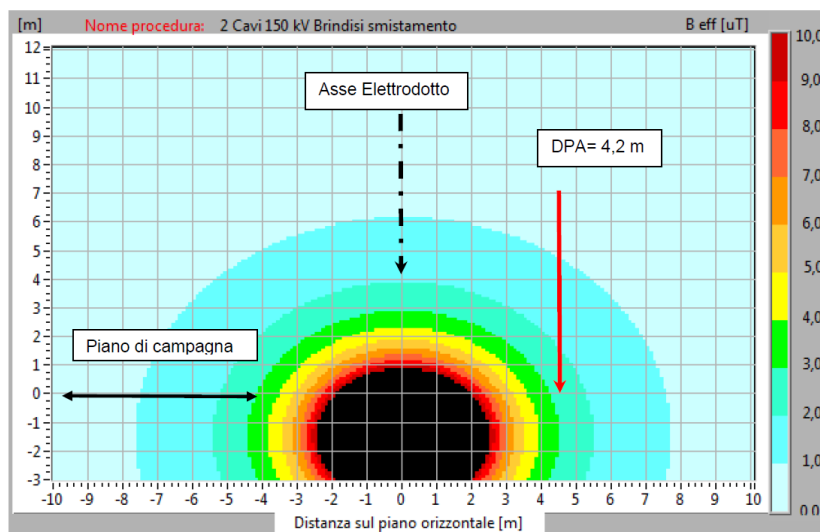
Figura 67: Mappa verticale induzione magnetica (B per terna di cavo, sezione tipo con indicazione della DPA - V=150 kV I = 1045 A)
