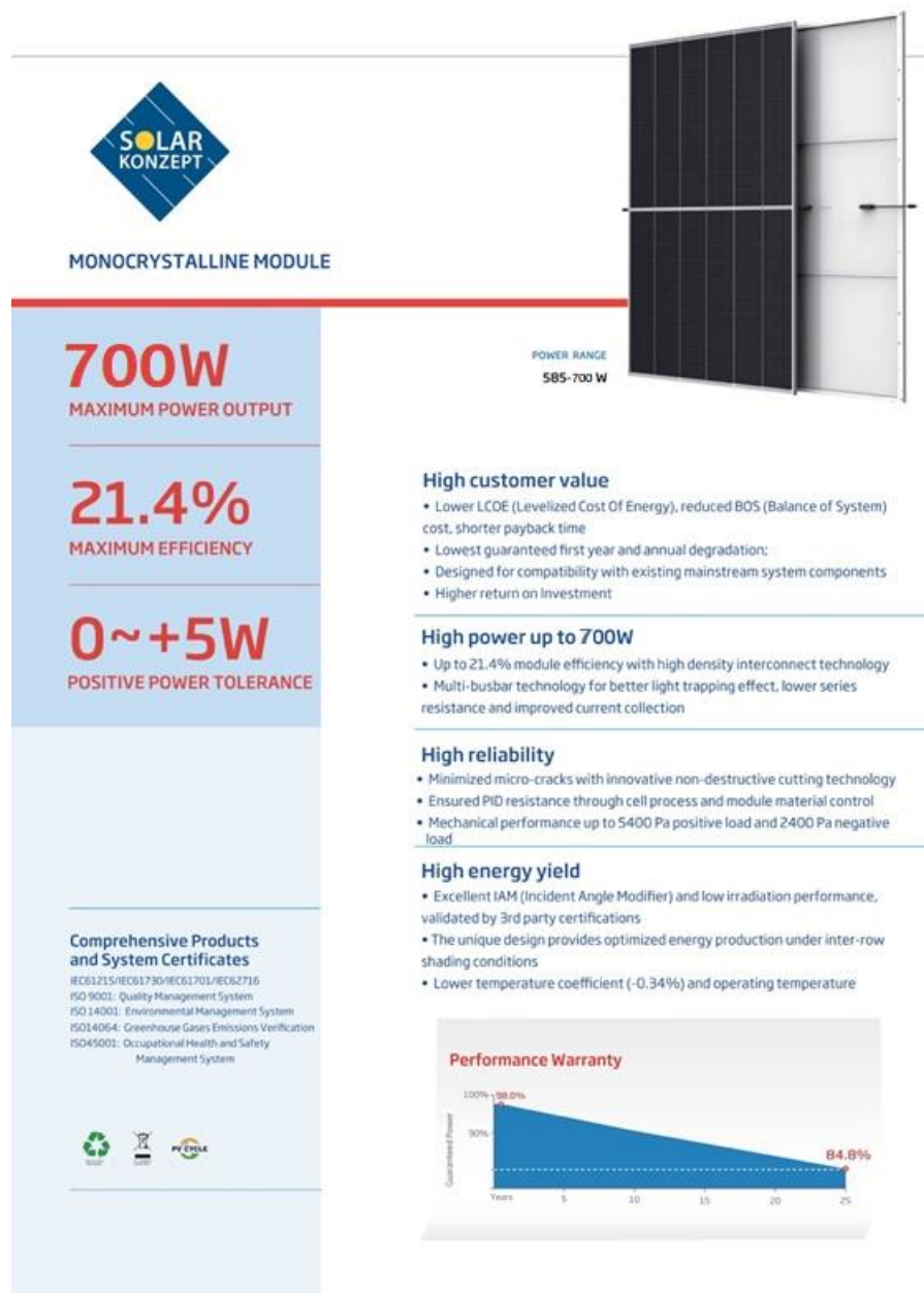
Figura 33: Scheda tecnica modulo fotovoltaico SKI
