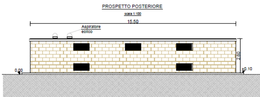
Figura 45: Prospetto anteriore della cabina di consegna.
