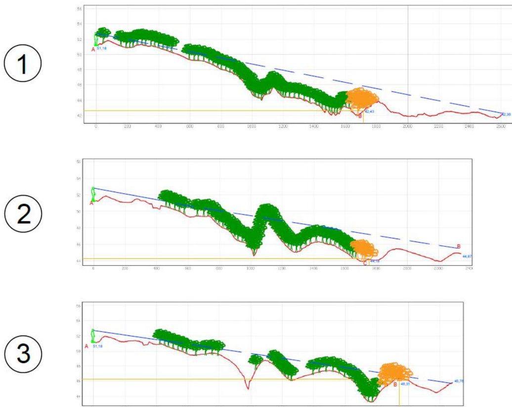
Figura 80: Profili longitudinali del terreno partendo da Masseria Chiusura Grande
