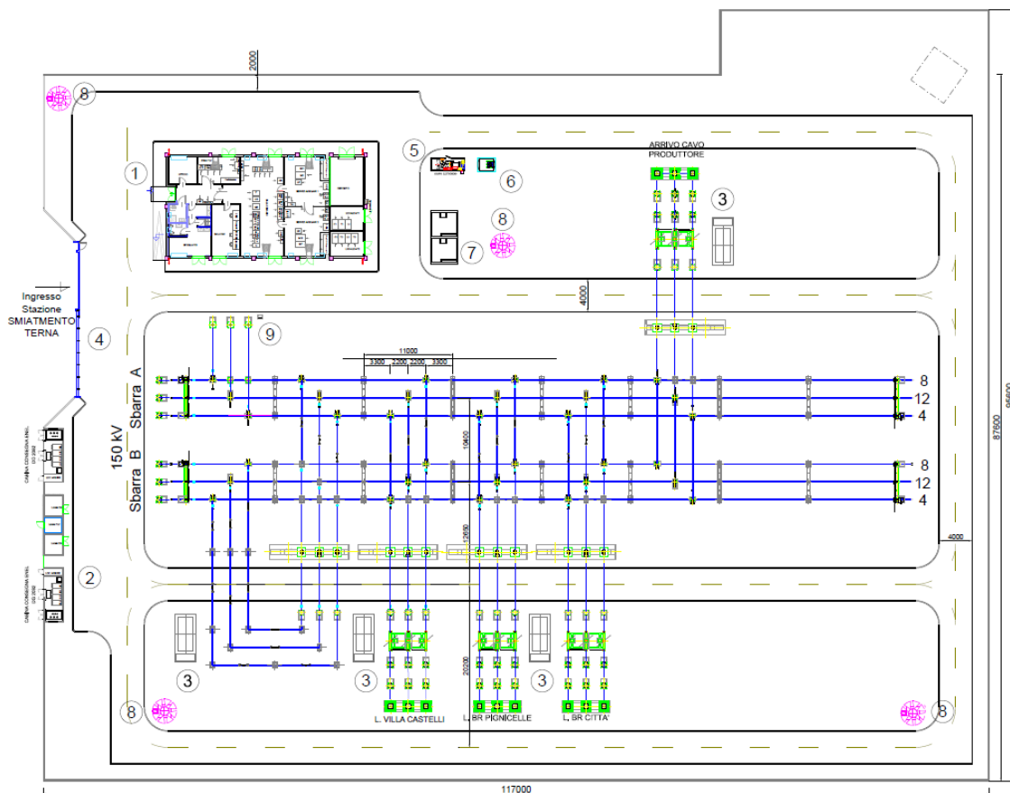
Figura 52: Layout definitivo della nuova stazione di smistamento da realizzare per la connessione dell'impianto alla RTN di TERNA
