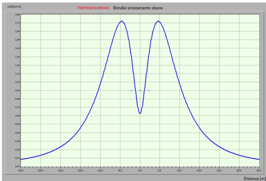
Figura 70: Profilo laterale campo elettrico (E) sbarre 150 kV.
