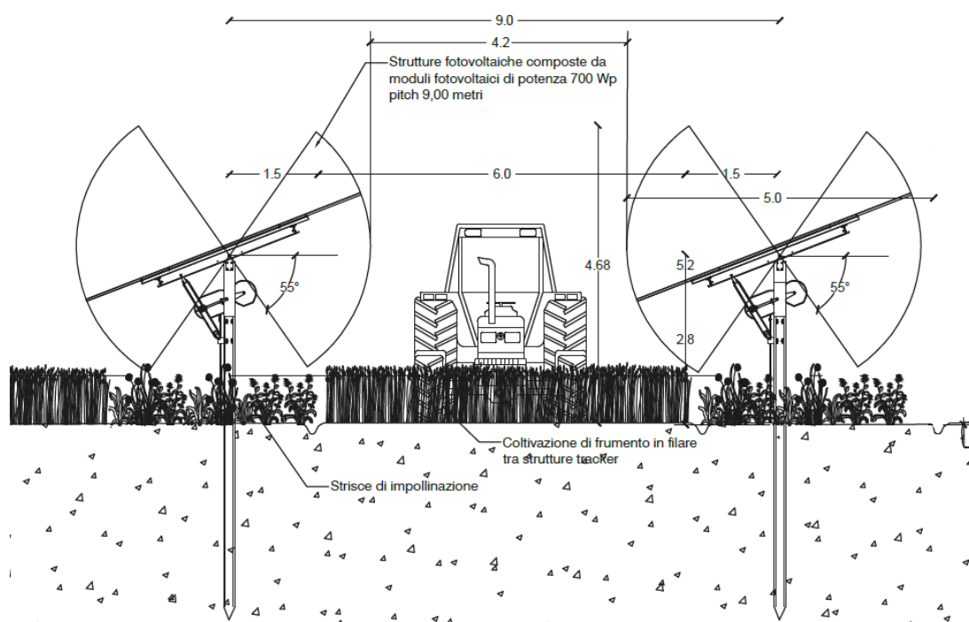
Figura 30: Prospetto frontale della struttura di sostegno dei moduli su tracker
