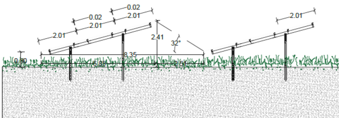
Figura 31: Vista in sezione delle strutture di supporto dei moduli con quotatura
