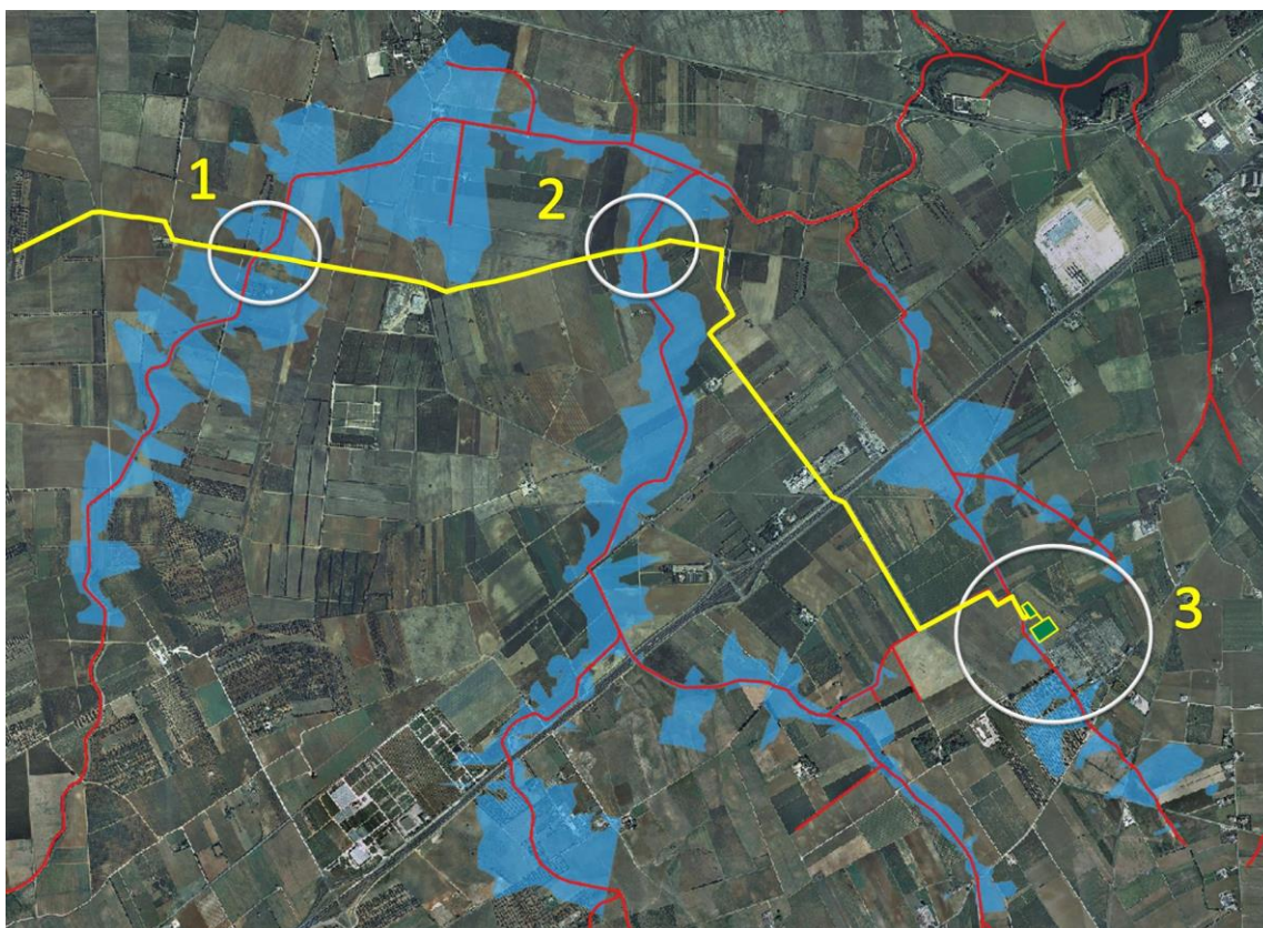
Figura 10: Risultati dello studio di compatibilità idrologica ed idraulica effettuato per tutti i reticoli presenti lungo il percorso dell'elettrodotto di connessione.
