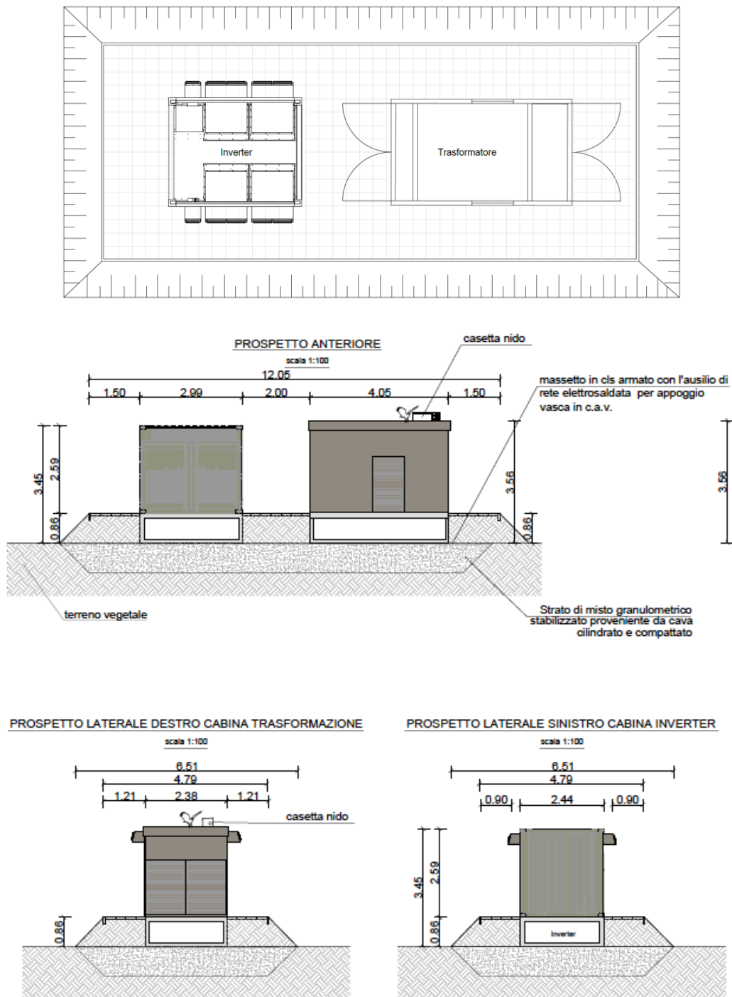
Figura 47: Pianta e particolari della cabina di campo
