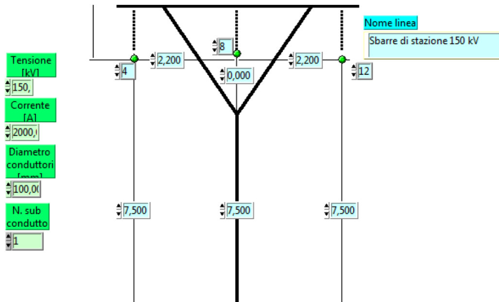
Figura 69: Schema sezione sbarre 150 kV nuova stazione Brindisi Smistamento con caratteristiche geometriche e di carico
