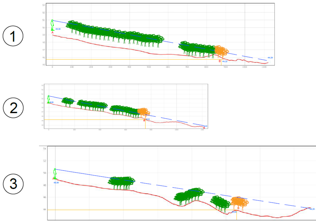
Figura 76: Profili longitudinali del terreno partendo da Masseria Buffi
