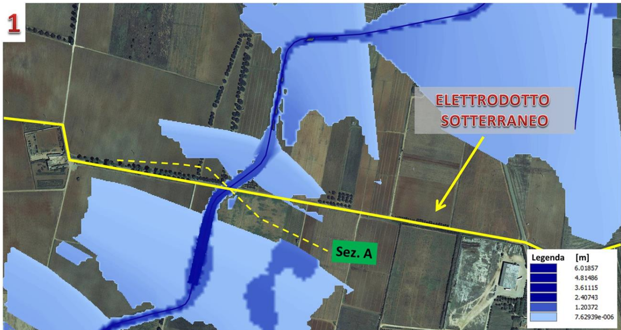
Figura 11: Risultati dello studio di compatibilità idrologica ed idraulica effettuato per tutti i reticoli presenti lungo il percorso dell'elettrodotto di connessione (punto 1)
