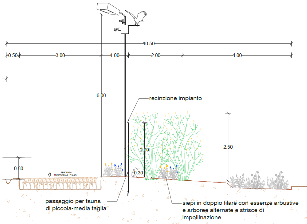
Figura 104: Particolare palo di videosorveglianza con stallo per uccelli
