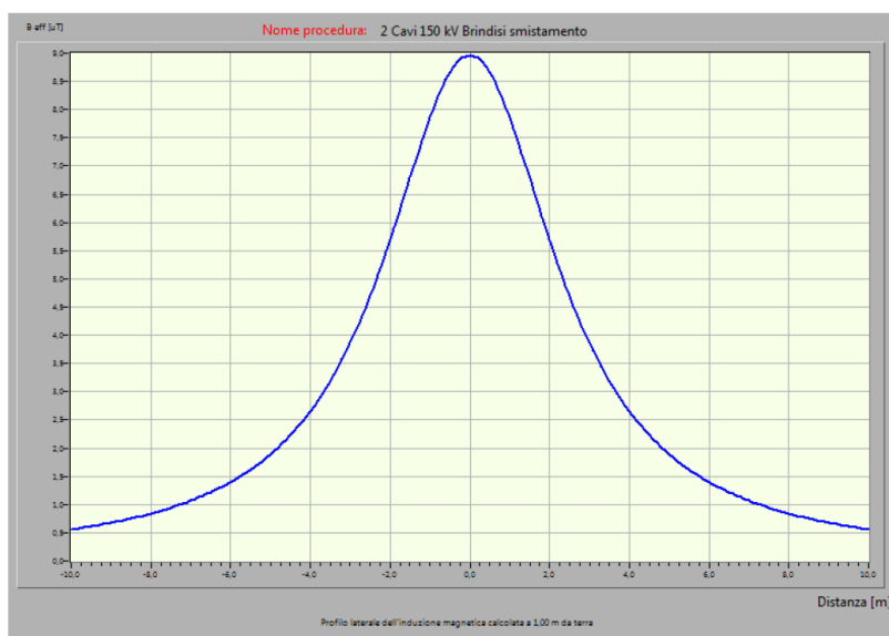
Figura 66: Profilo laterale induzione magnetica (B) - V=150 \text{ kV} I=1045 \text{ A} per ogni terna di cavo
