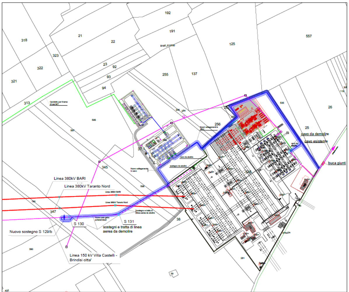
Figura 14: Stazione di Trasformazione 30/150 kV
