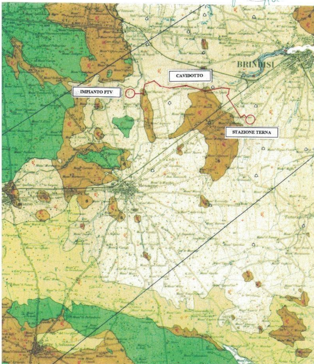
Figura 9: Stralcio Carta Geologica d'Italia - scala 1:100.000
