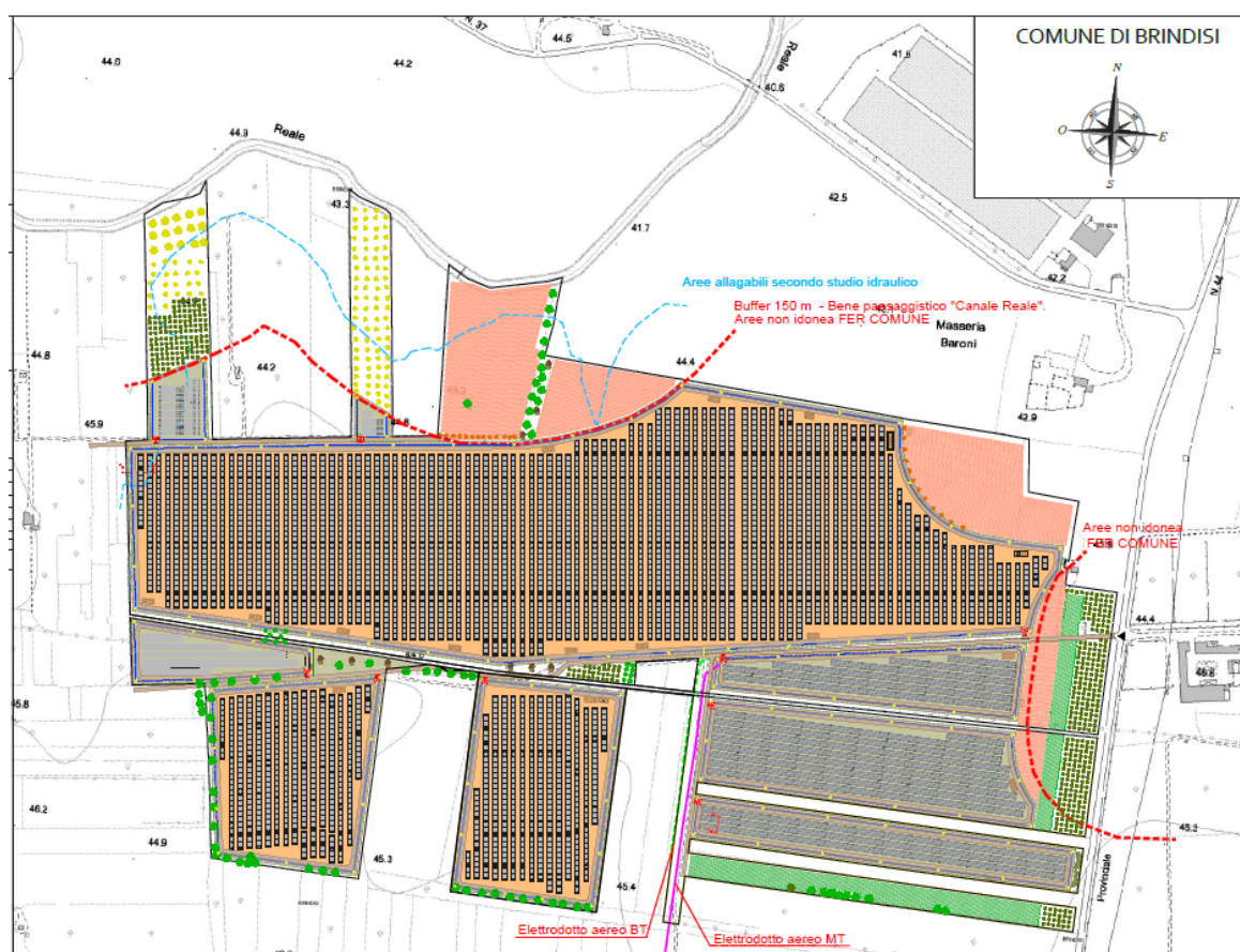
Figura 12: Campo Fotovoltaico
