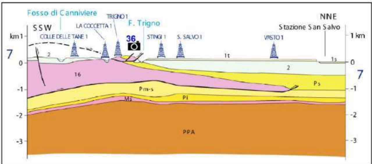
Figura 81 - Sezione geologica n. 7, Fosso di Canniviere – Staz. San Salvo
