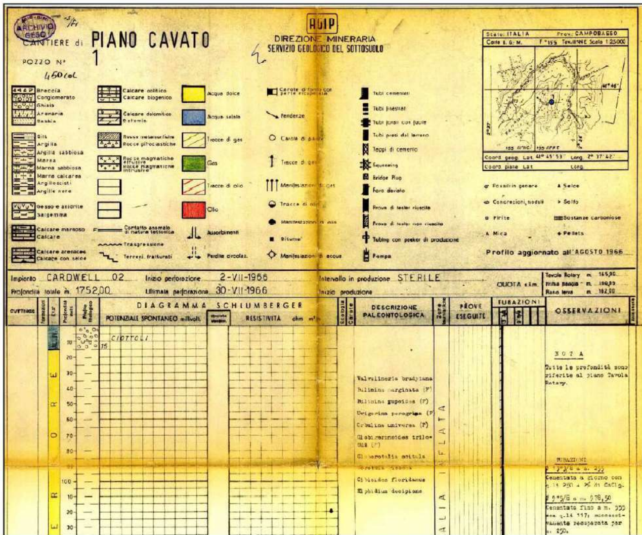
Figura 86 - Scheda dei primi 130 m della stratigrafia del pozzo per ricerca idrocarburi denominato "Piano"
