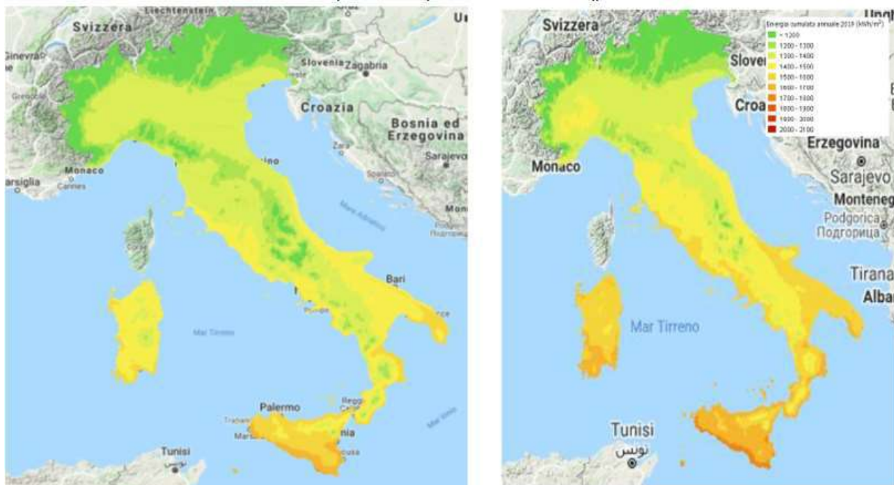
Figura 15 Radiazione solare cumulata annua nel 2018 e nel 2019
