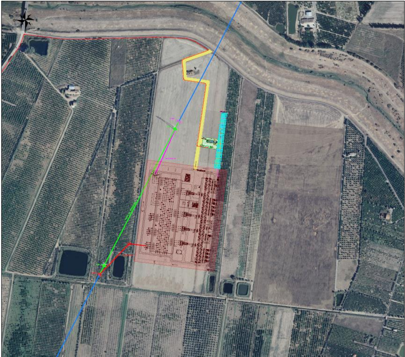
Figura 11- Lay out generale Impianto di Utenza e Impianto di Rete
