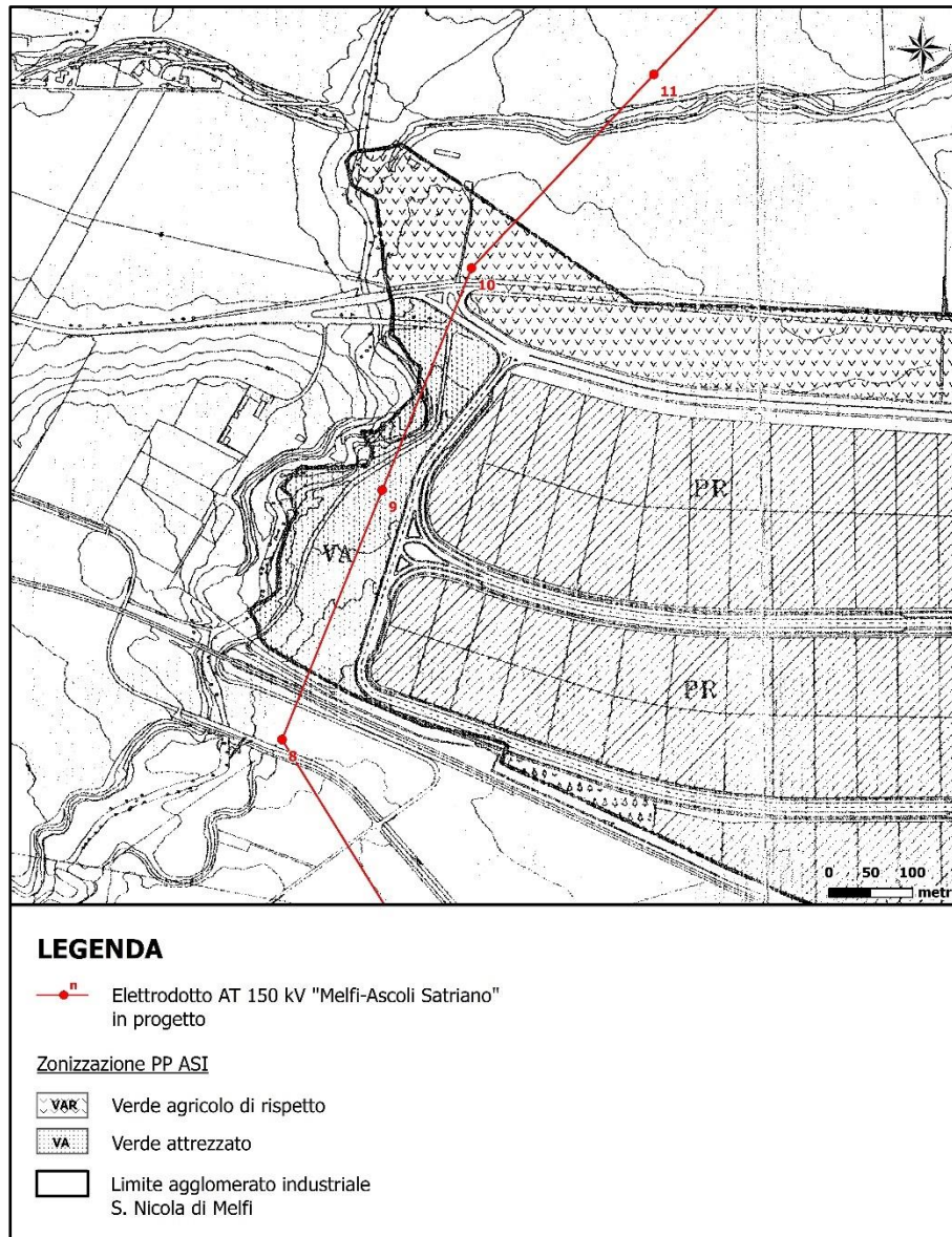
Figura 2.3.2.1a Estratto Tavola 4b "Planimetria generale di progetto – zonizzazione" del Piano Particolareggiato del Consorzio ASI
