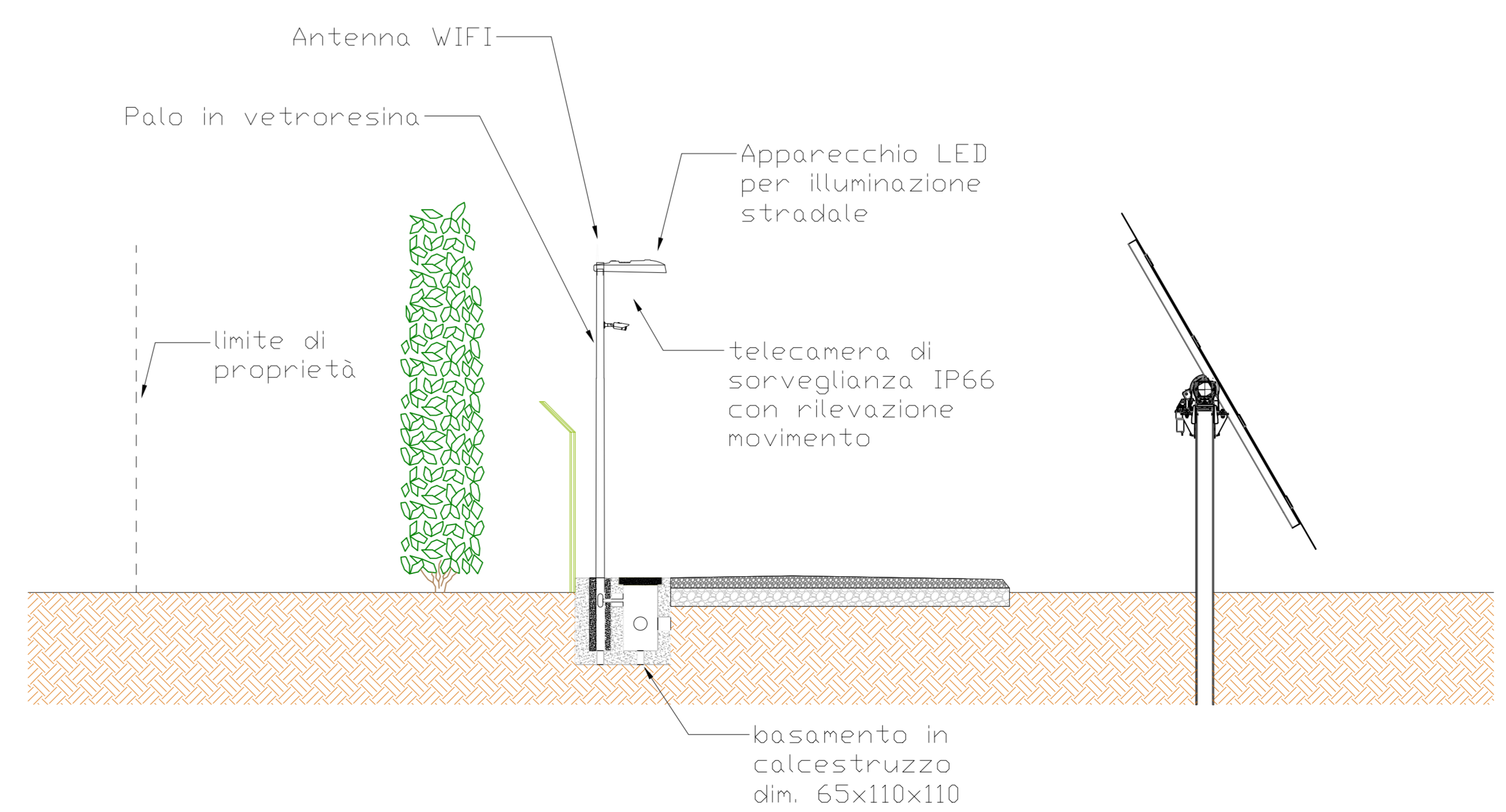
SEZIONE scala 1:50
