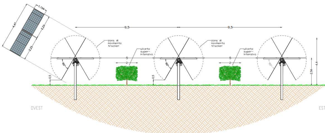
Fig. 1 Sistema Agro-fotovoltaico
